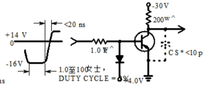
图2.关闭时间
