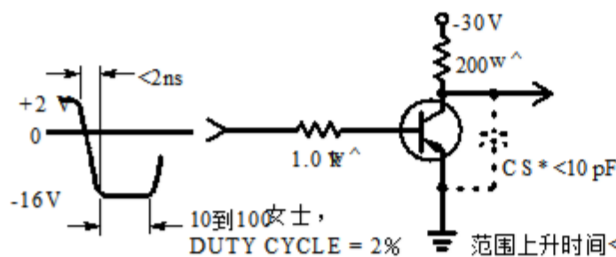
图1.开启时间
