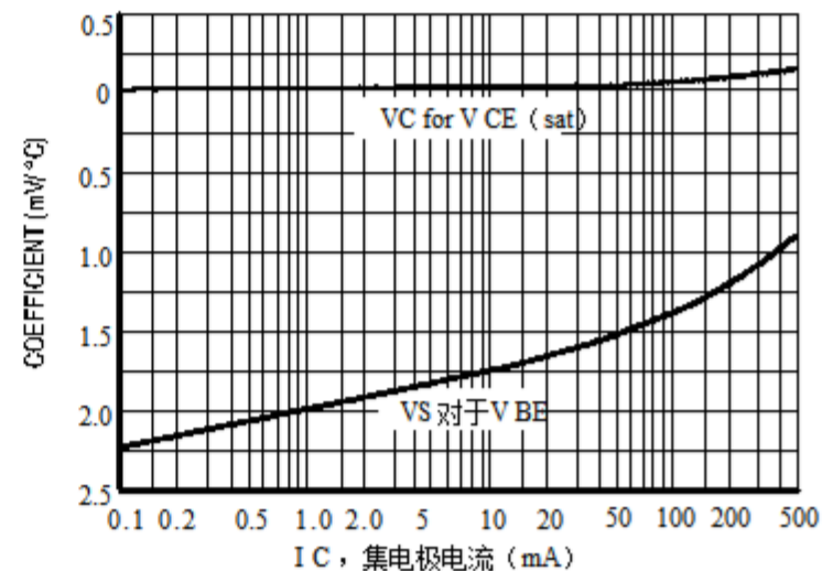
图6.温度系数
