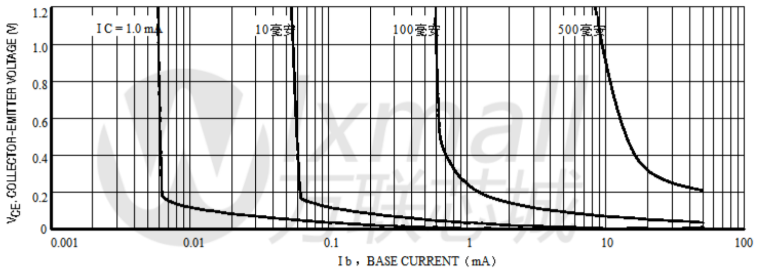
图4.收集器饱和区域
