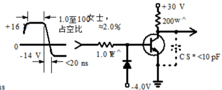
图2.关闭时间
