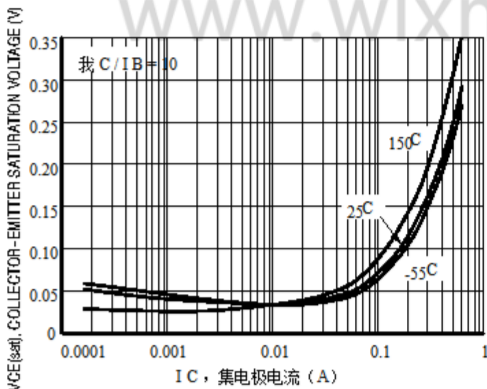
图5.集电极 - 发射极饱和电压 与收集器电流
