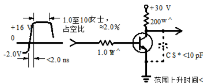
开关时间等效测试电路
