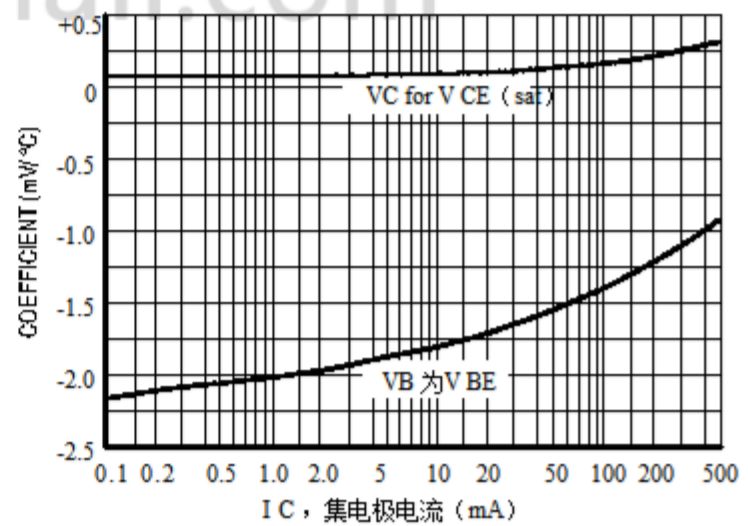
图6.温度系数
