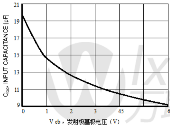
图9.输入电容与发射极基极 电压
