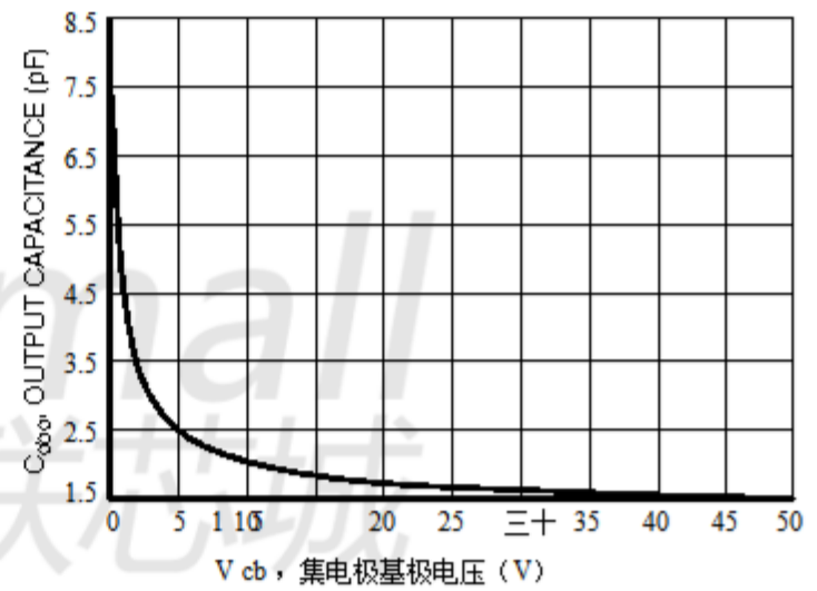
图10.输出电容与收集器 基极电压
