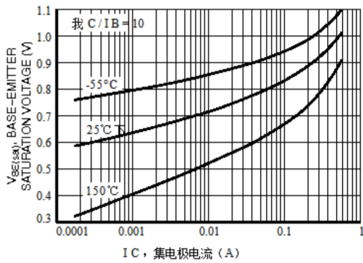
图7.基极发射极饱和电压与 集电极电流
