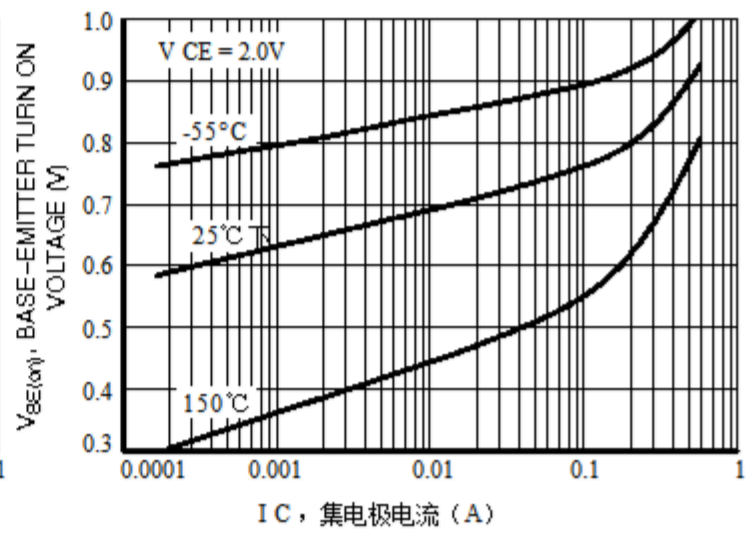
图8.基极发射极开通电压与 集电极电流
