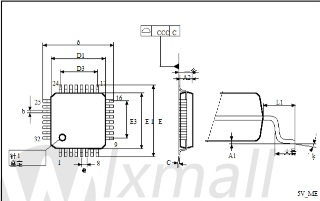
图45： 32引脚扁平扁平封装（7 x 7）
