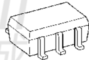
SSOP5-P-0.65A
