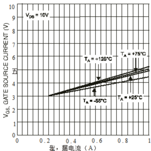
图5典型的传输特性
