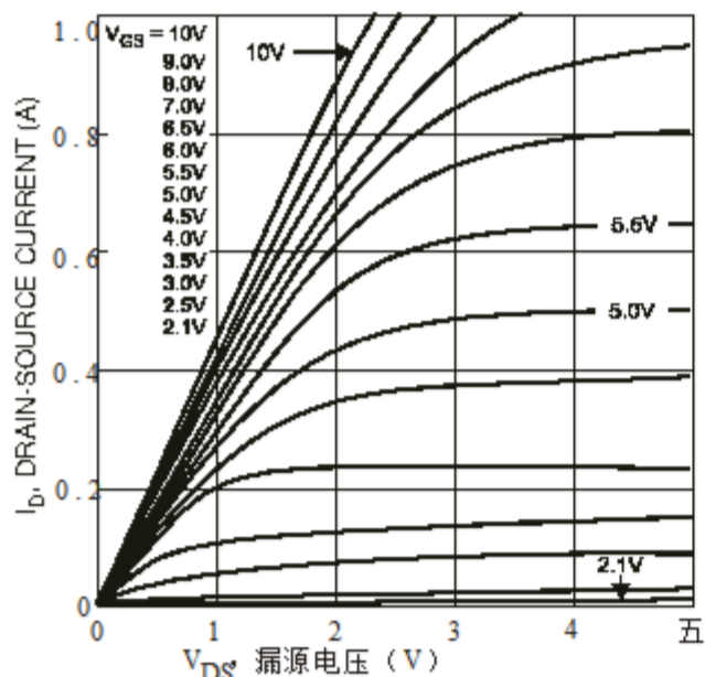
图1 On-Region特性
