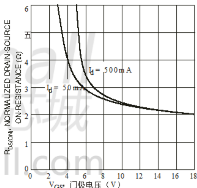
图4导通电阻与栅源电压的关系
