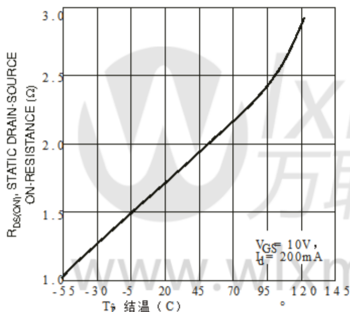
图3导通电阻与结温的关系
