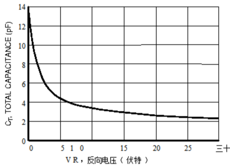
图4.总电容
