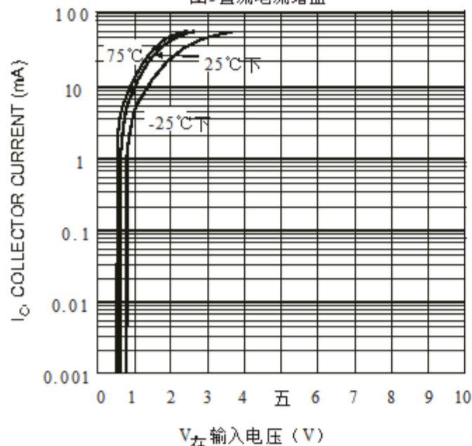
图5 集电极电流与 V_{in} 输入电压
