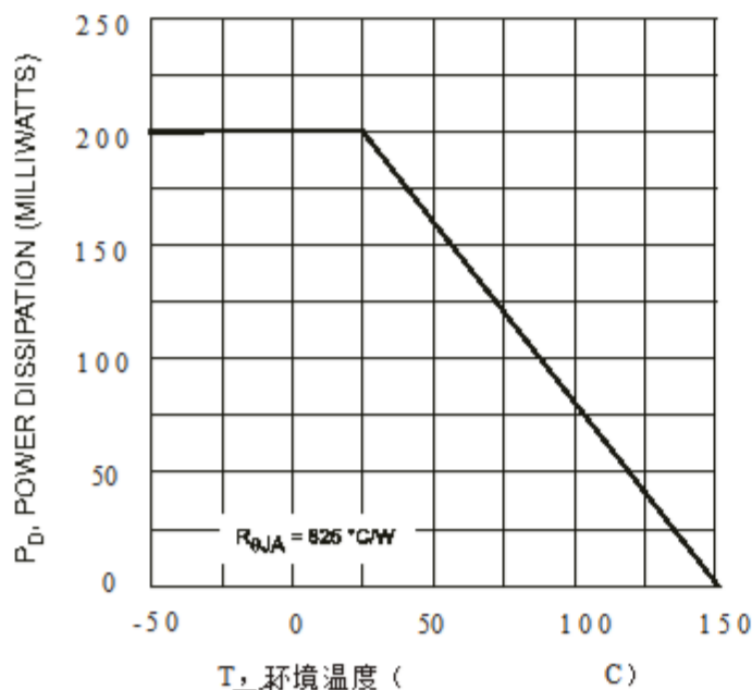
图1 降额曲线
