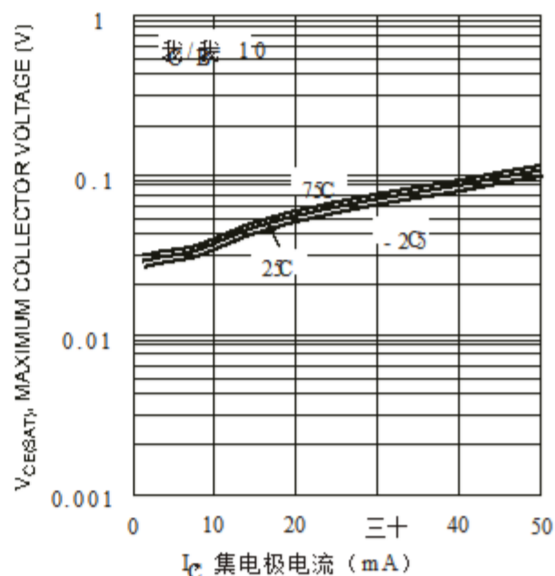
图2 V_{CE} (饱和) 与 I_C
