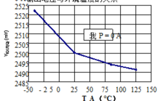
0 A输出电压与环境温度的关系
