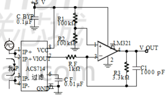
应用3. 此配置可将增益提高至610 mV/A (使用ACS714ELC-05A进行测试)。
