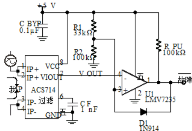
应用5. 10 A过流故障锁存器. 故障阈值由R1和R2. 该电路锁定过电流故障并保持到5 V电压断电.
