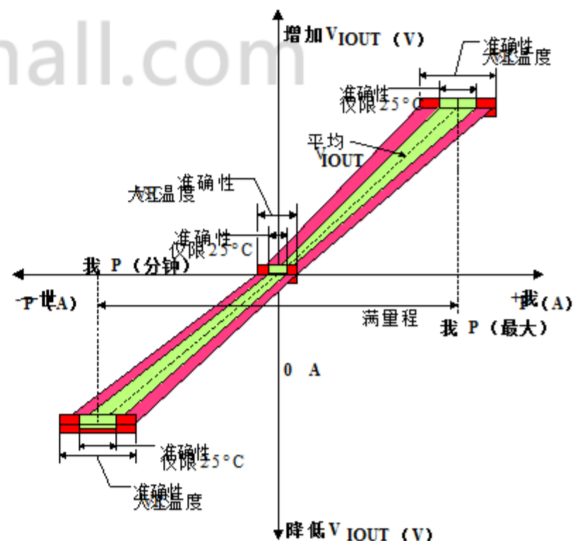
输出电压与感测电流的关系 在 0 A 和满量程电流时的精度
