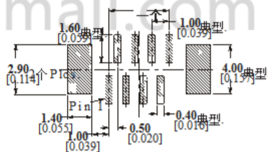
推荐的PCB布局
