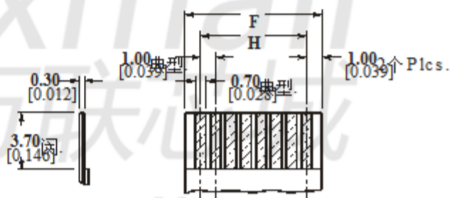
推荐FPC布局
