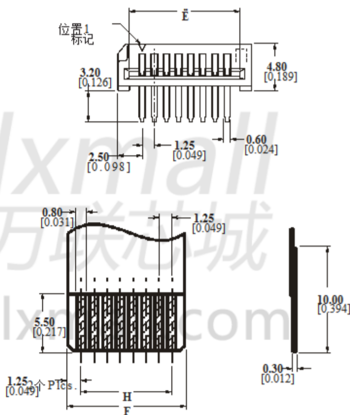
推荐的FFC布局
