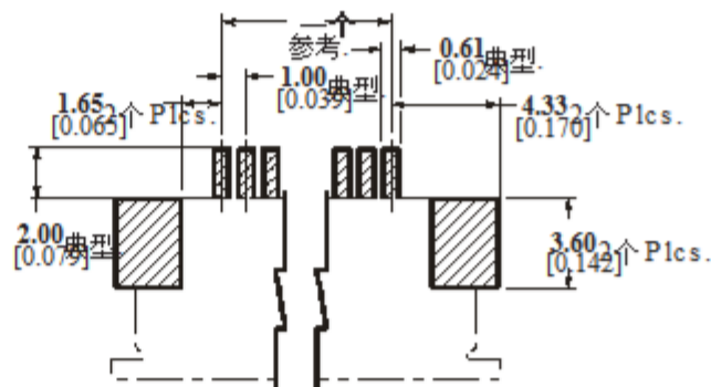
推荐的PCB布局
