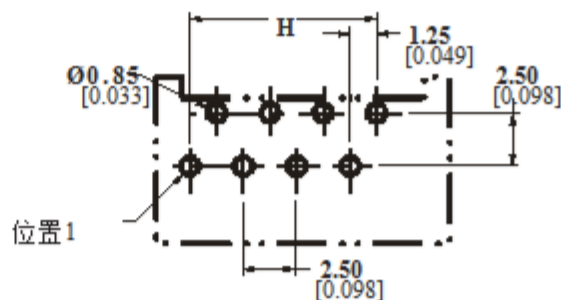
推荐的PCB布局
