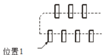
推荐的PCB布局 用于奇数位置连接器
