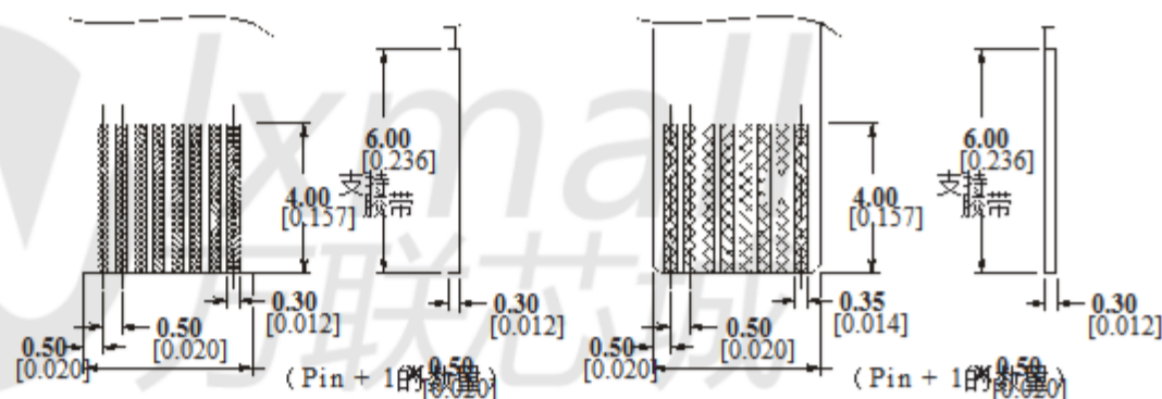
推荐的FFC布局
