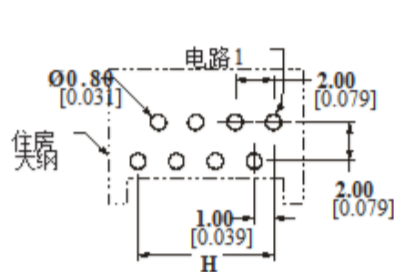
推荐的PCB布局 1.60 [0.063] 厚度 (对于偶数位置连接器)
