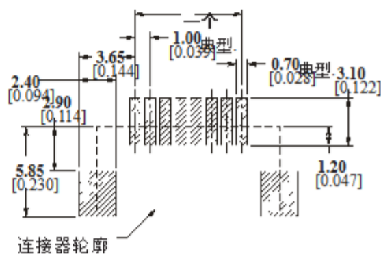
推荐的PCB布局
