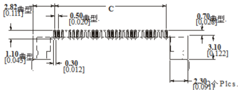
推荐的PCB布局
