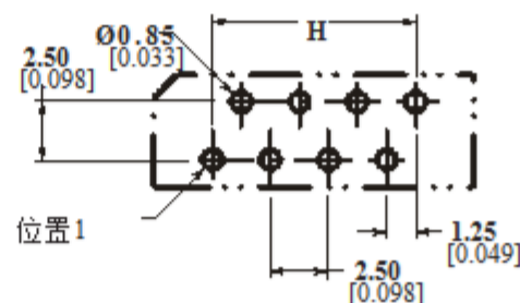
推荐的PCB布局
