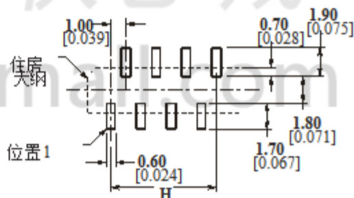
推荐的PCB布局 对于偶数位置连接器
