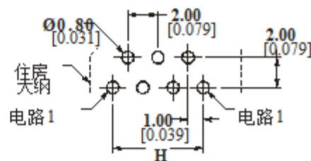
推荐的PCB布局 1.60 [0.063] 厚度 (对于奇数位置连接器)
