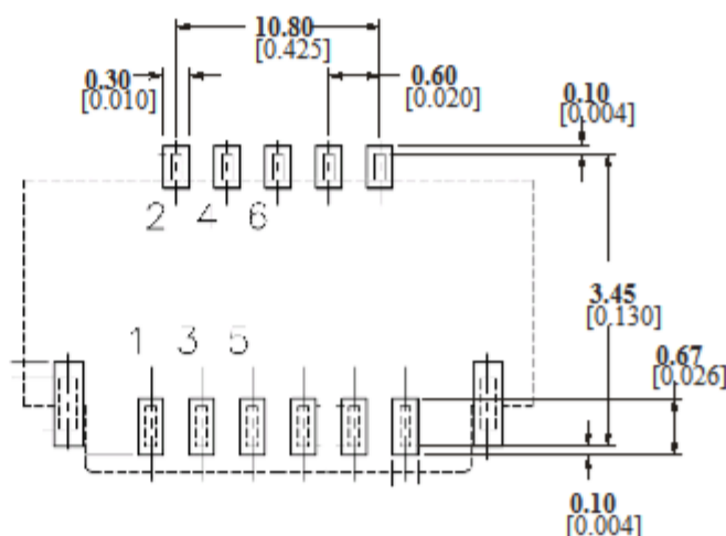
推荐的PCB布局
