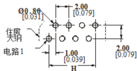
推荐的PCB布局 1.60 [0.063] 厚度 (对于偶数位置连接器)
