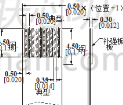
推荐的FPC布局
