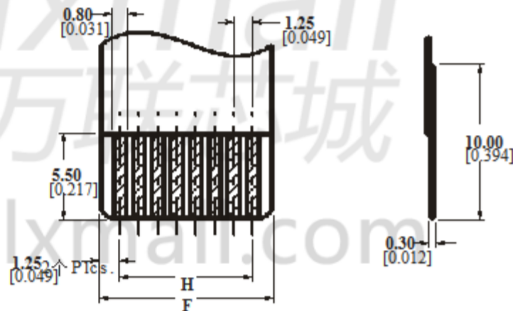
推荐的FFC布局
