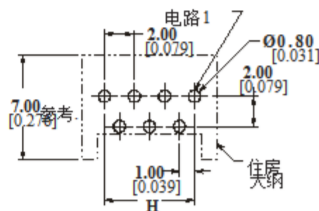
推荐的PCB布局 1.60 [0.063] 厚度 (对于奇数位置连接器)
