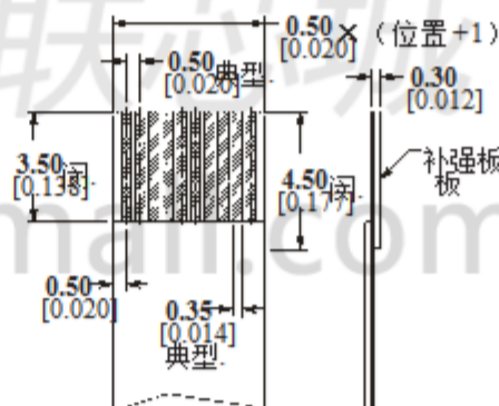
推荐的FPC布局
