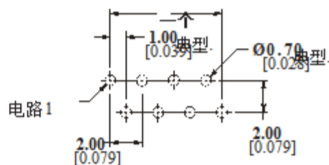
推荐的PCB布局
