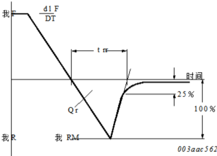
图5.反向恢复定义;拖尾恢复
