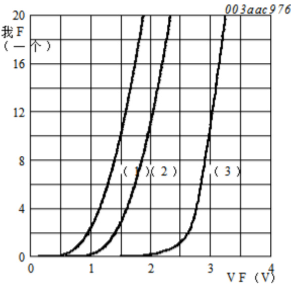
图4.正向电流与正向电压的关系
