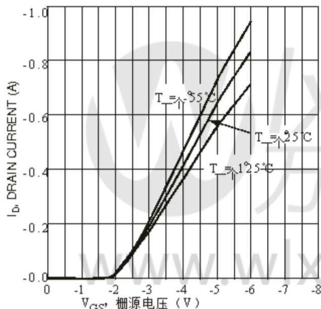
图3漏极电流与栅源电压的关系
