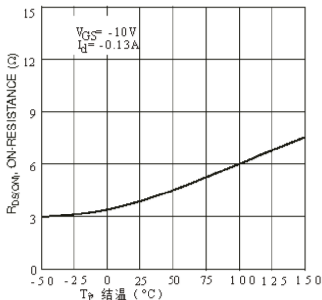
图5导通电阻与结温的关系
