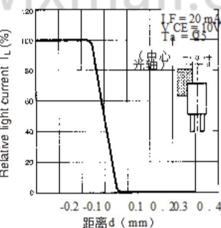
感应位置特征 (典型)
