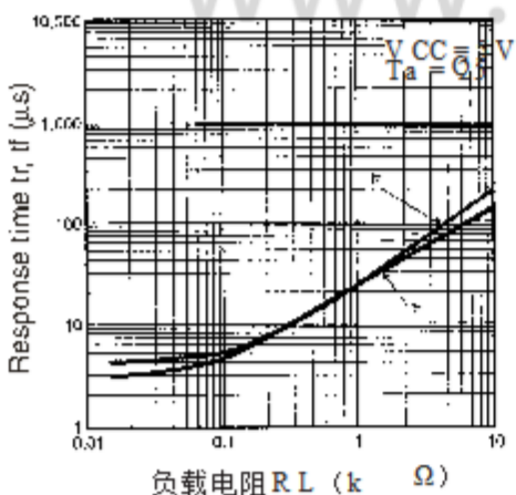
响应时间与负载抵抗 - 特点 (典型)
