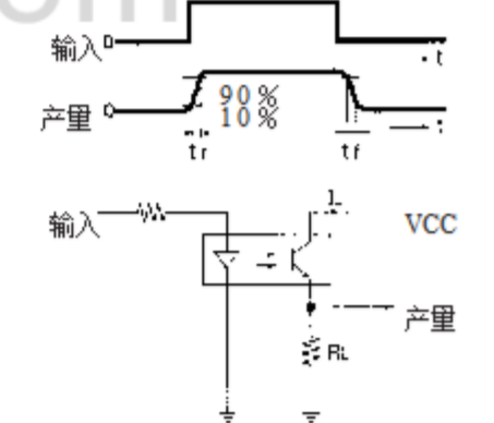
响应时间测量 电路
