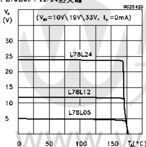
图6. L78L05 / 12/24热关断
