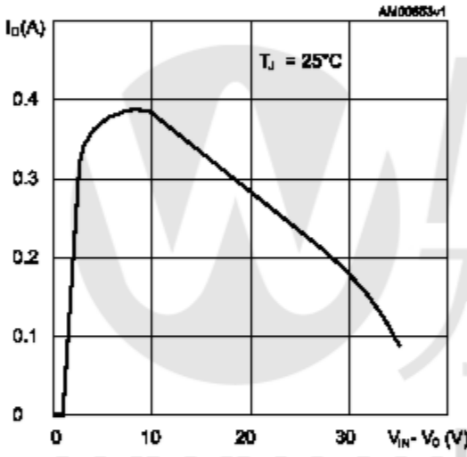
图12. L78L短路输出电流
