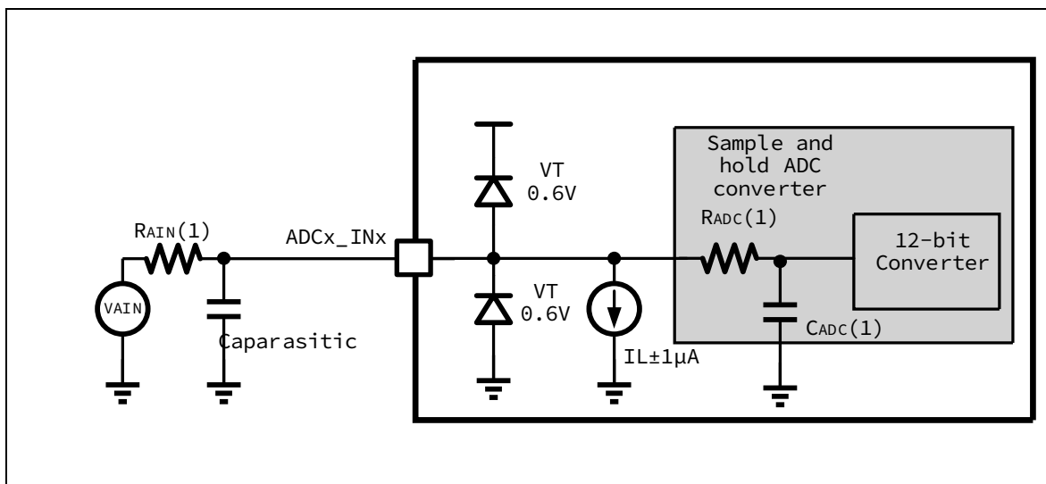
图 3-18 使用 ADC 的典型连接
