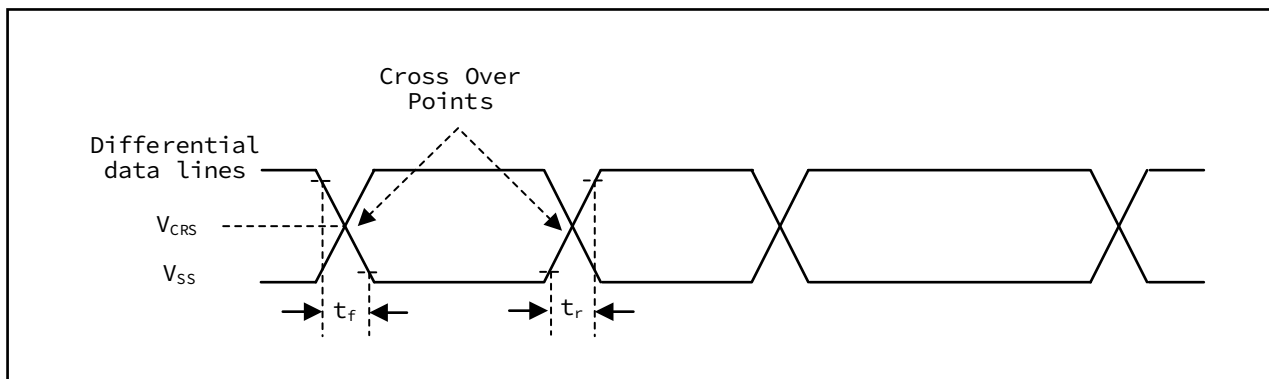
图 3-13 USB 上升/下降时间及 Cross Over 电压定义
