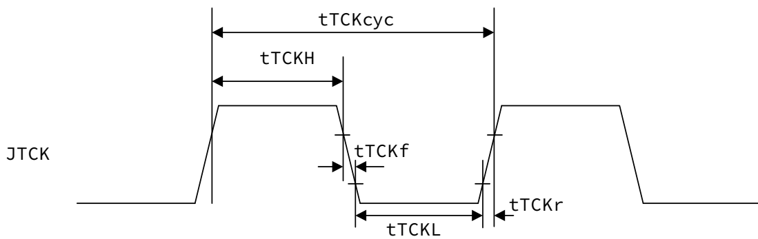
图 3-14 JTAG JTCK 时钟
