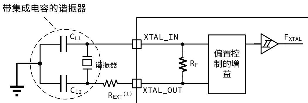
图 3-16 采用 8 MHz 晶振的典型应用
