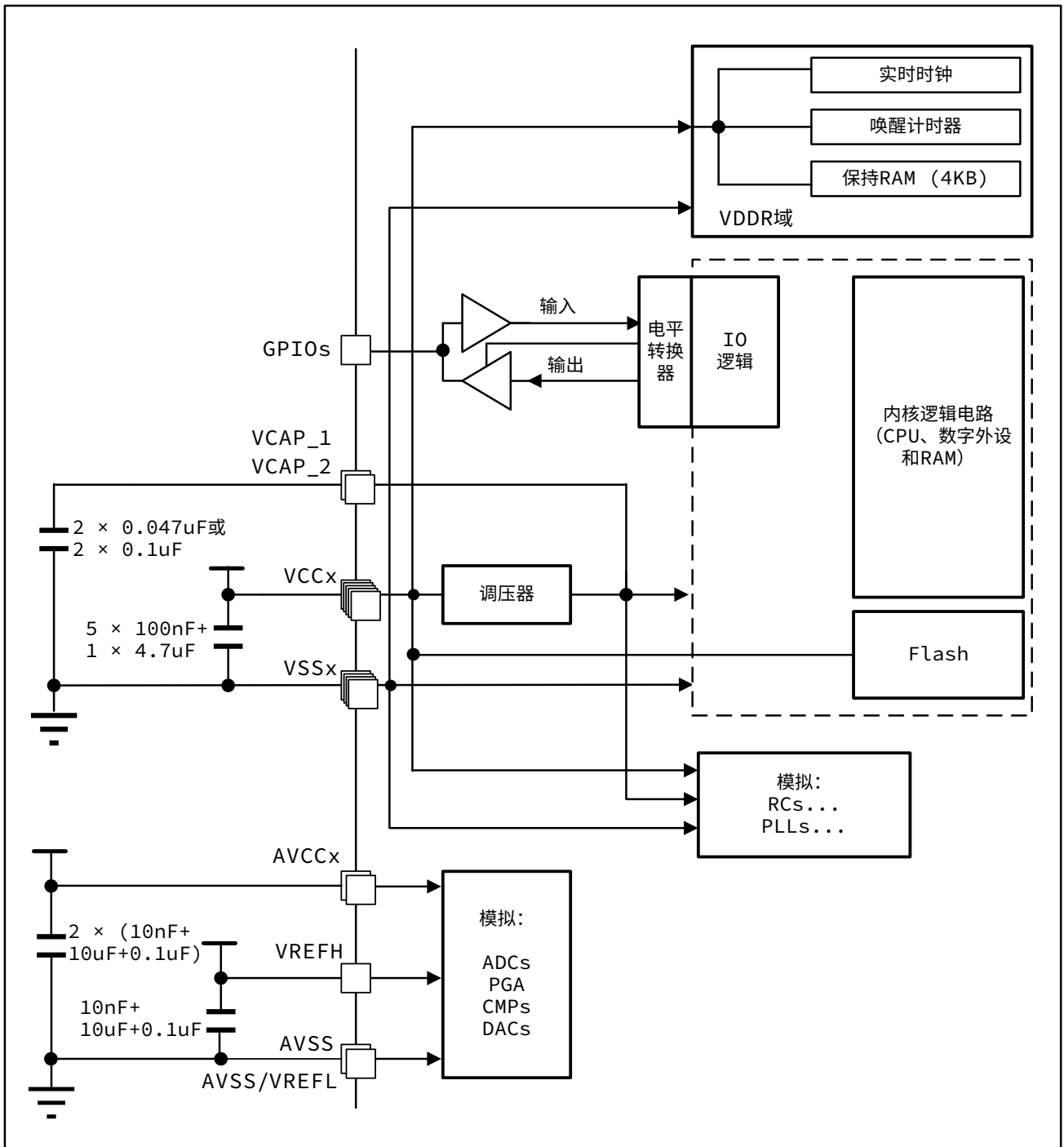
图 3-2 电源方案 (HC32A460PETB)
