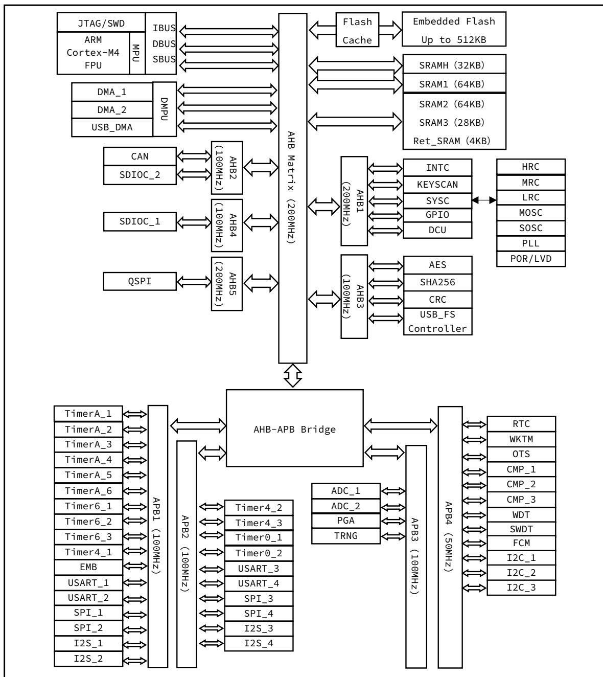
图 1-1 功能框图
