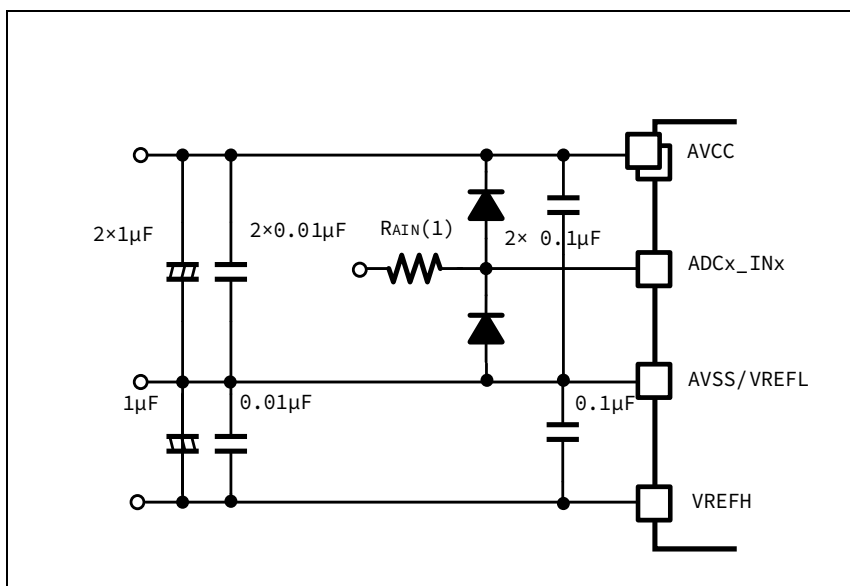
图 3-19 电源和参考电源去耦例
