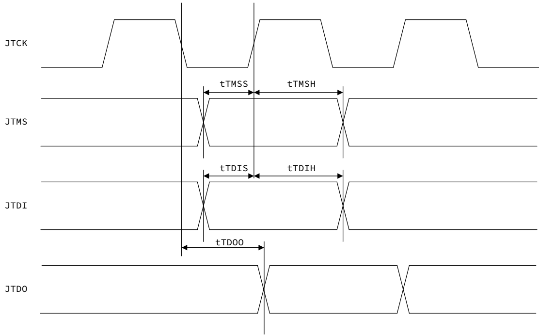
图 3-15 JTAG 输入输出
