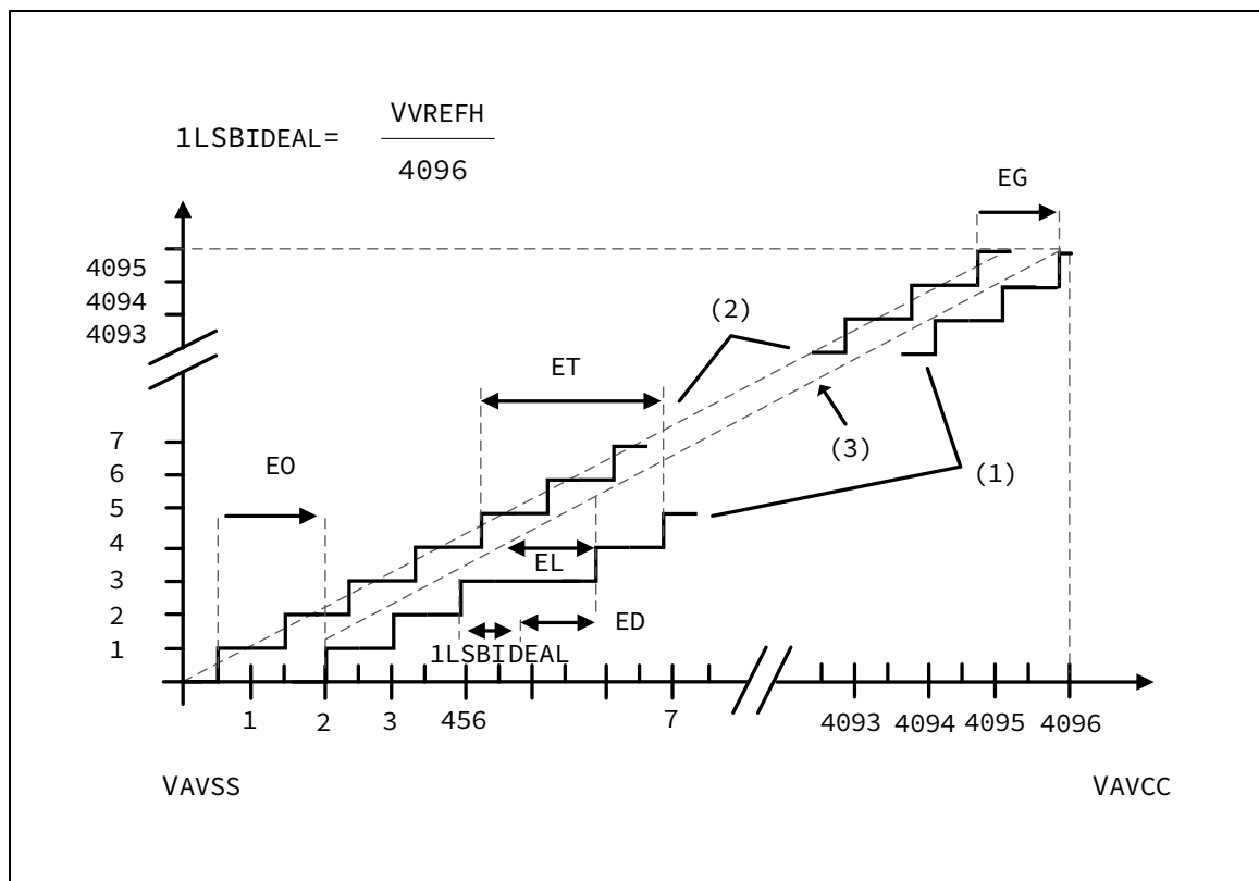
图 3-17 ADC 精度特性
