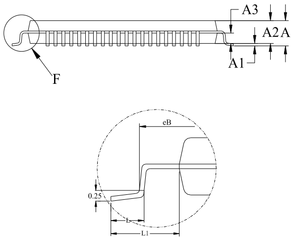
DETAIL: F
