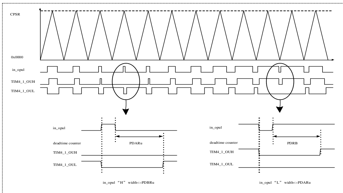
图 15-21 脉宽异常时的死区定时器模式下的波形输出
