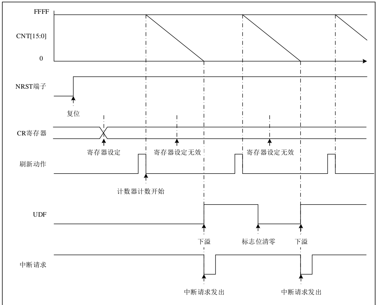
图 21-2 软件启动例
