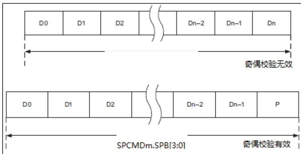
图 24-4 数据格式
