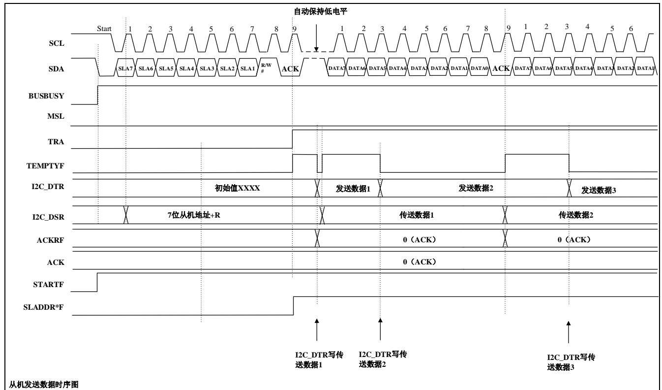
图 23-7 7 位地址格式的从机发送模式时序图（例）
