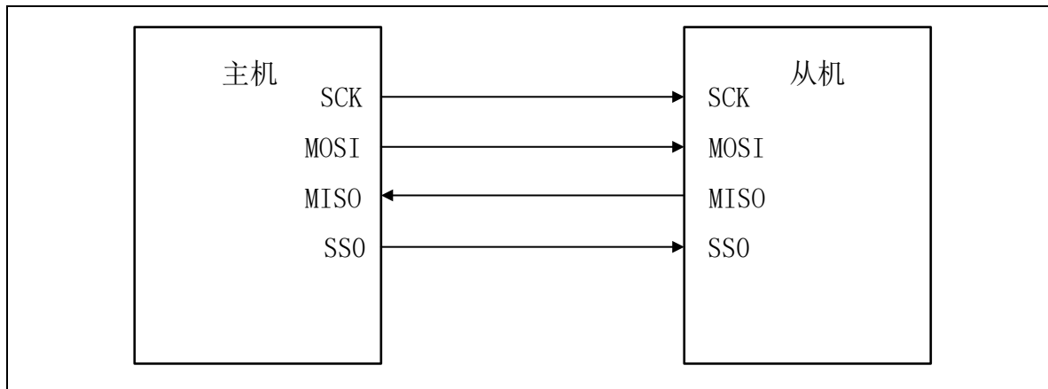
图 24-2 主机模式结构
