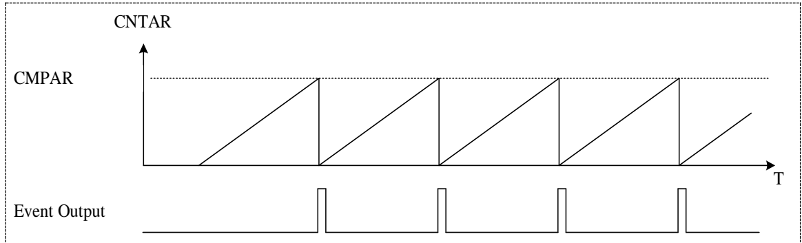
图 20-2 Timer0 计数时序图
