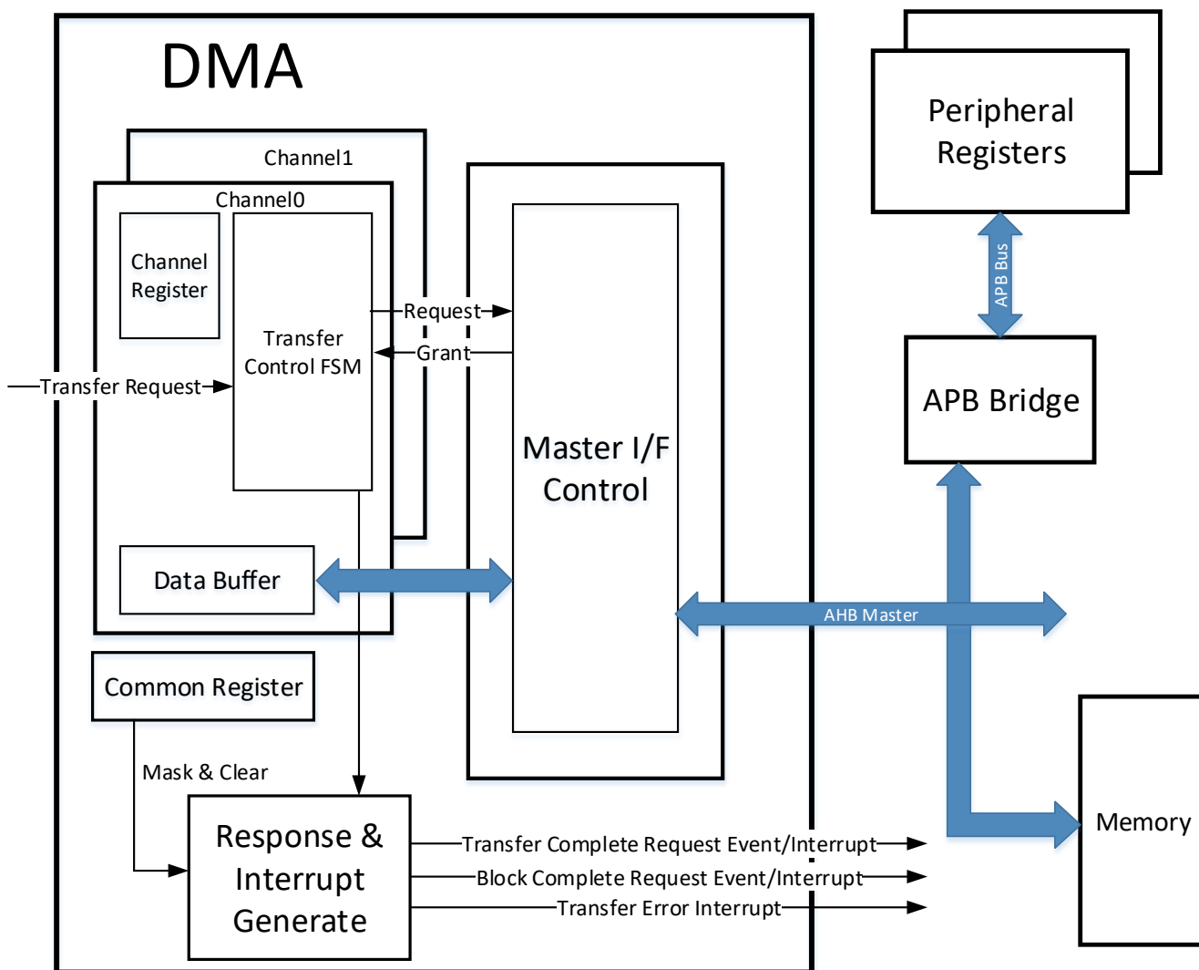
图 11-1 DMA 结构图
