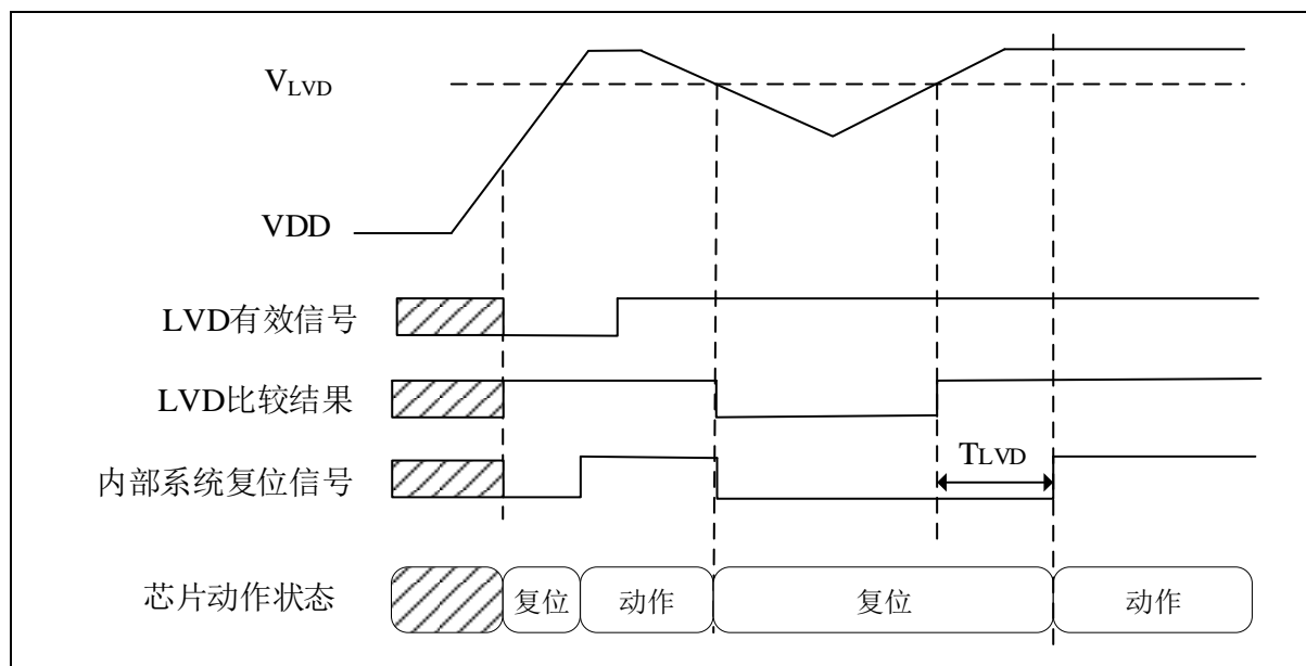
图 3-3 LVD 复位
