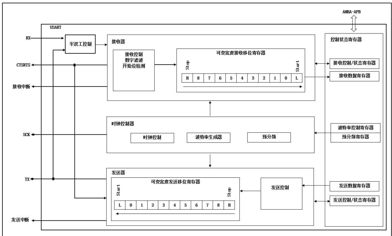
图 22-1 USART 系统框图
