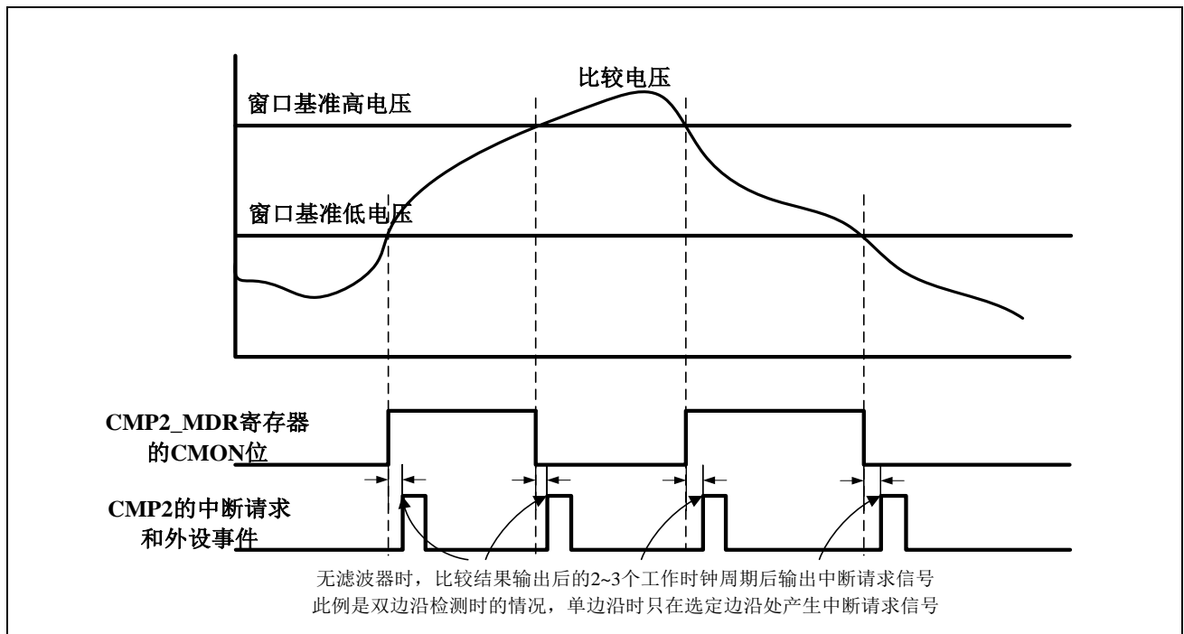
图 13-3 窗口比较模式工作示意图
