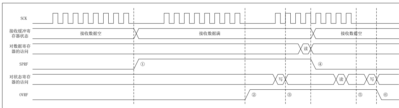
图 24-10 过载错误处理
