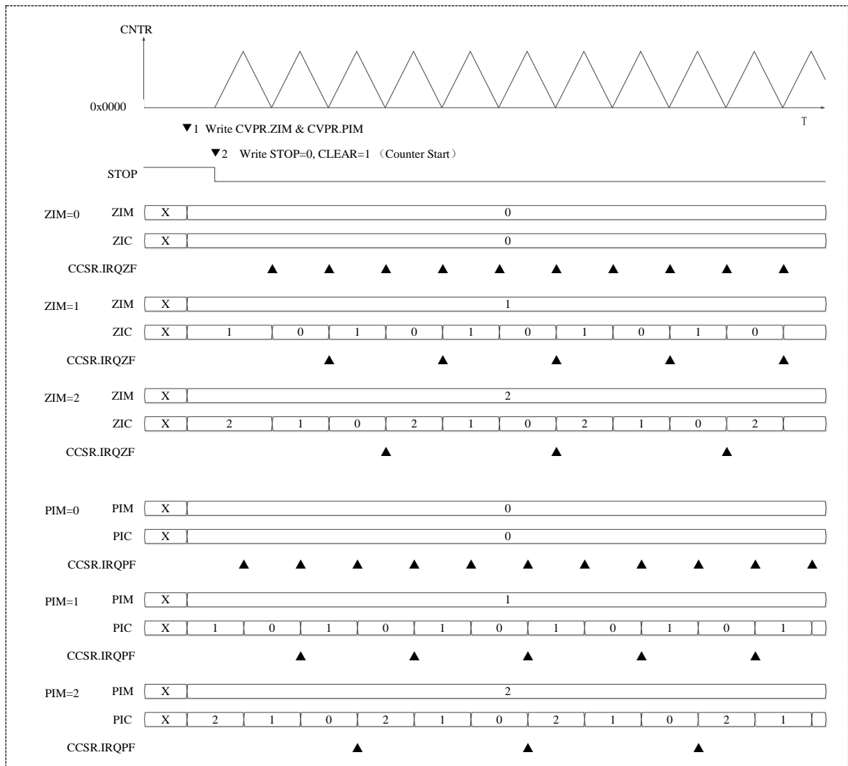
图 15-23 周期间隔响应时序图
