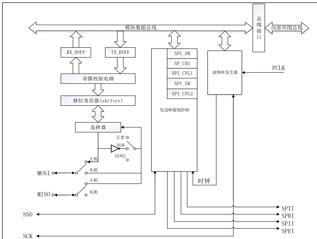
图 24-1 系统框图
