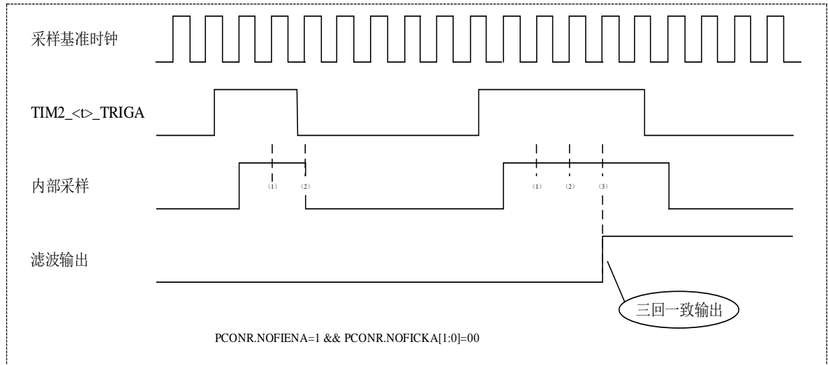
图 19-7 TRIG 输入端口的数字滤波
