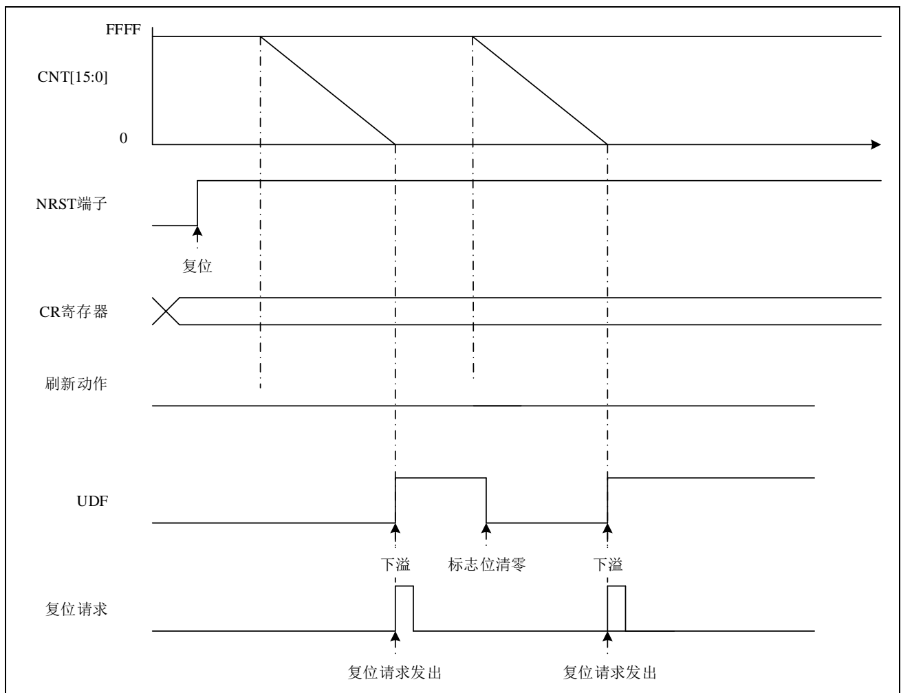
图 21-1 硬件启动例
