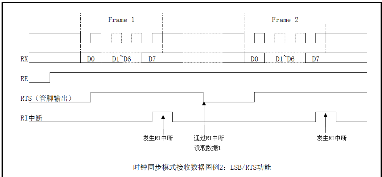
图 22-18 时钟同步模式接收数据图例 2
