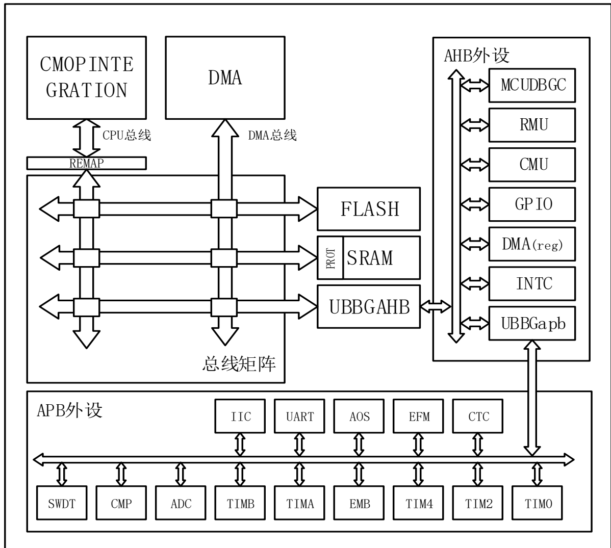
图 2-1 总线架构
