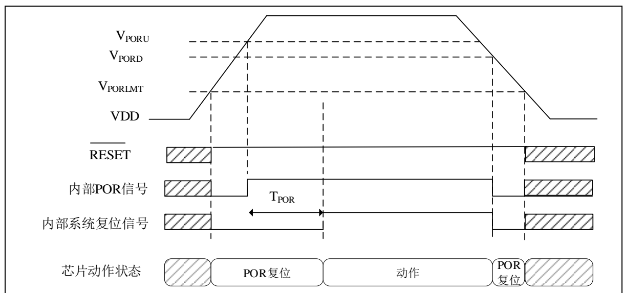
图 3-1 上电复位
