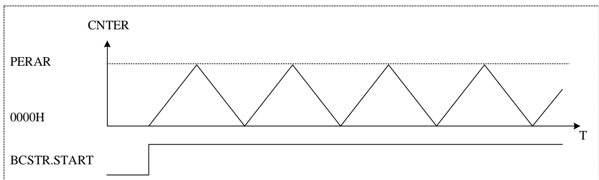
图 17-3 三角波波形
