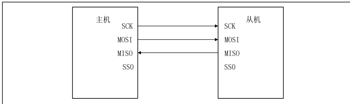
图 24-3 三线式时钟同步运行
