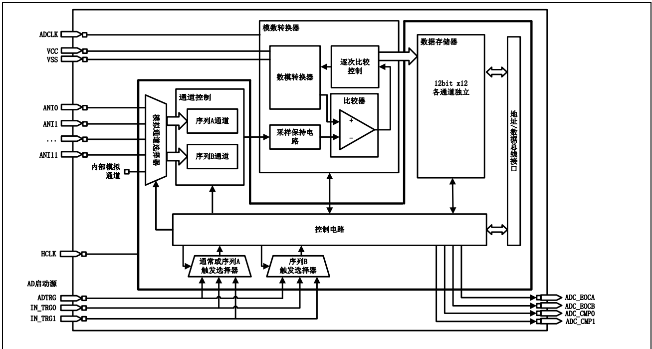
图 14-1 ADC 框图
