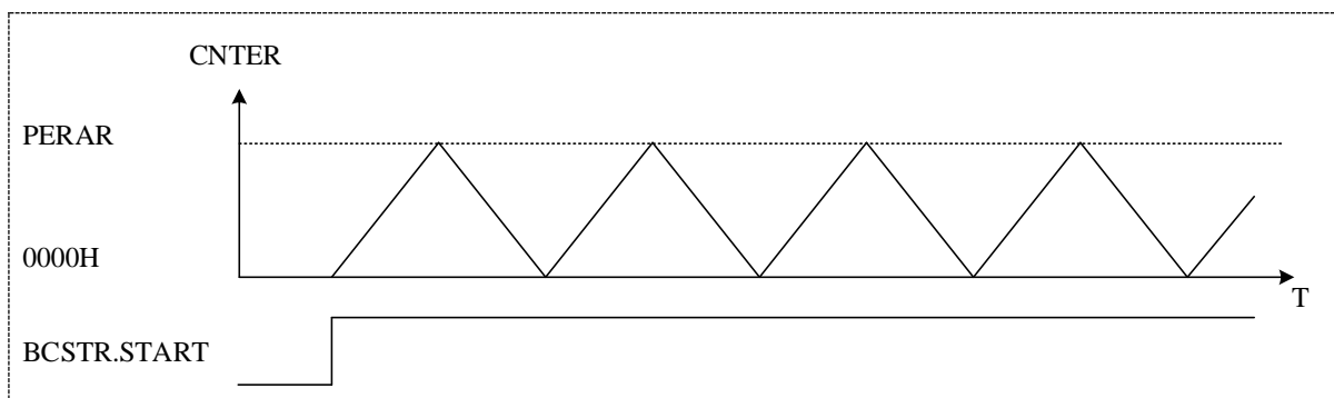
图 18-3 三角波波形
