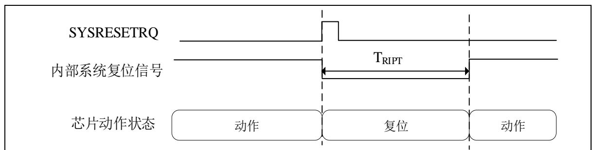
图 3-5 软件复位
