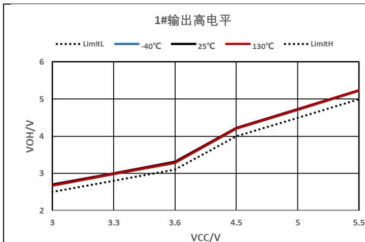
图 7-7 接收机输出高电平
