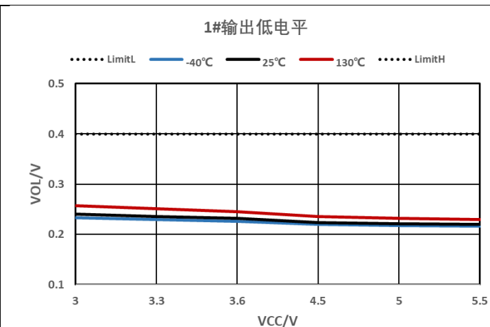
图 7-8 接收机输出低电平
