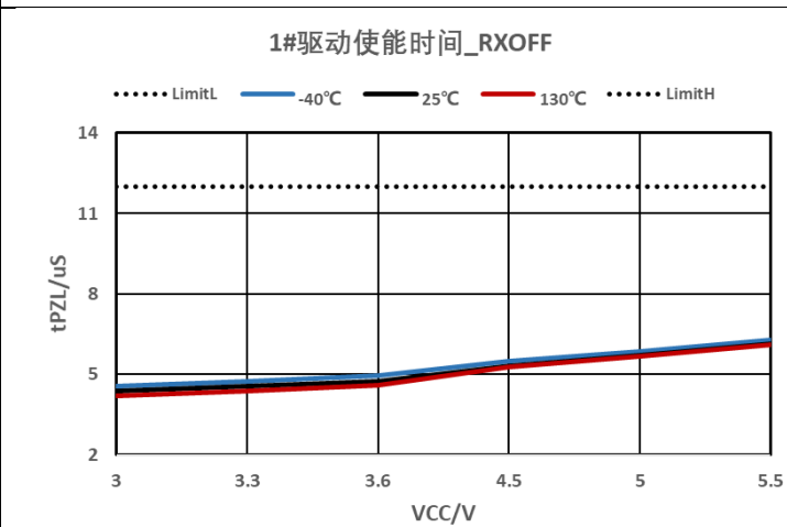
图 7-12 驱动使能时间
