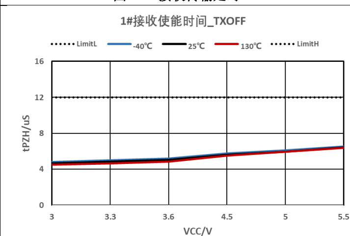
图 7-16 接收使能时间
