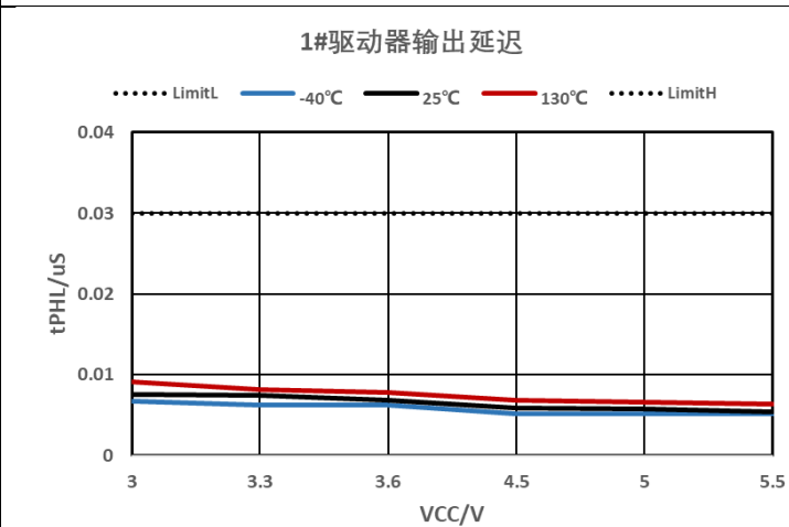
图 7-10 驱动器输出延迟
