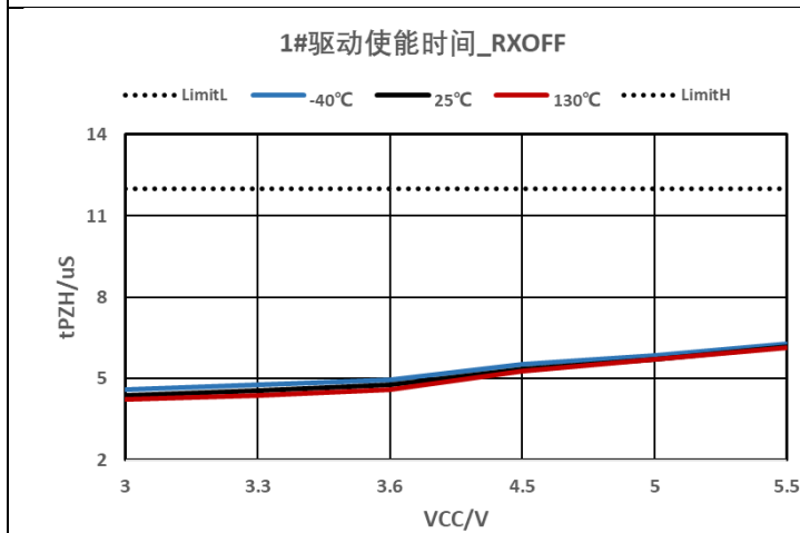
图 7-11 驱动使能时间
