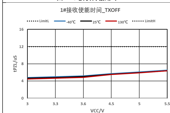
图 7-15 接收使能时间
