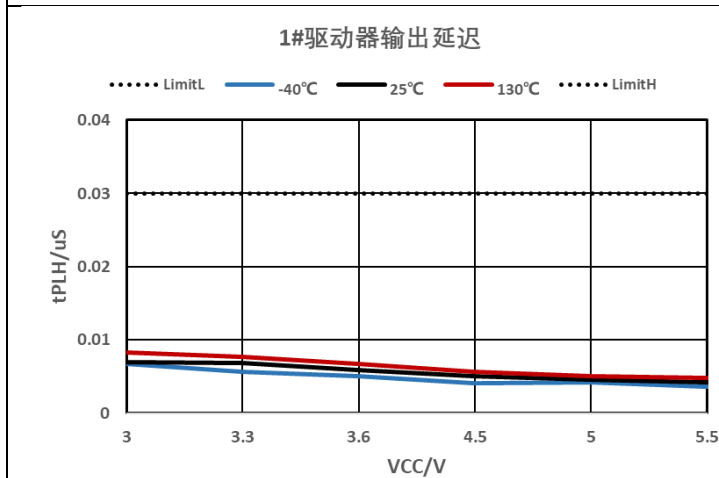
图 7-9 驱动器输出延迟
