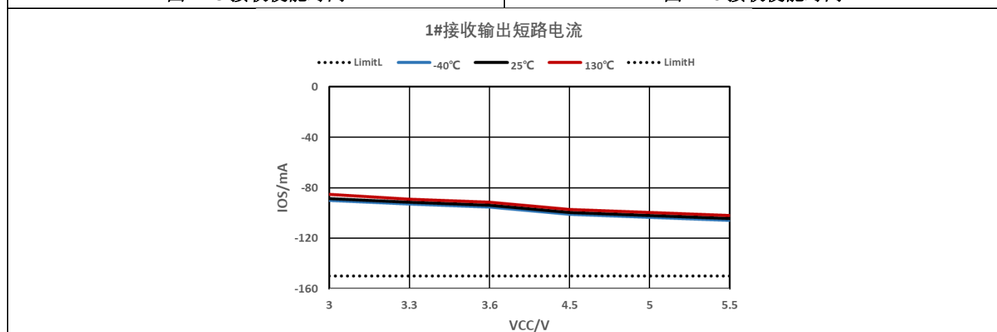
图 7-17 接收输出短路电流
