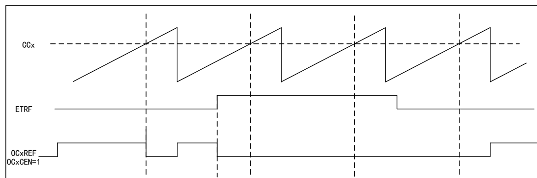
图 36 OCxREF 时序图
