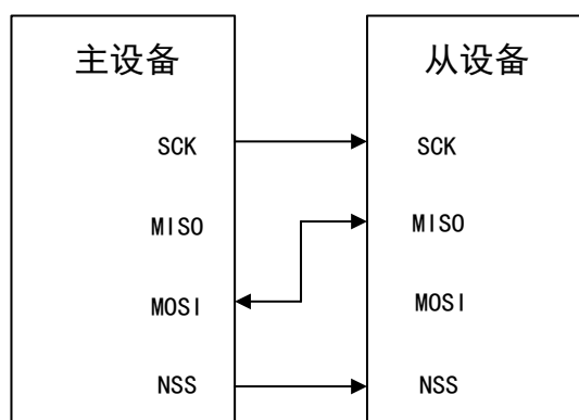
图 90 双向线连接
