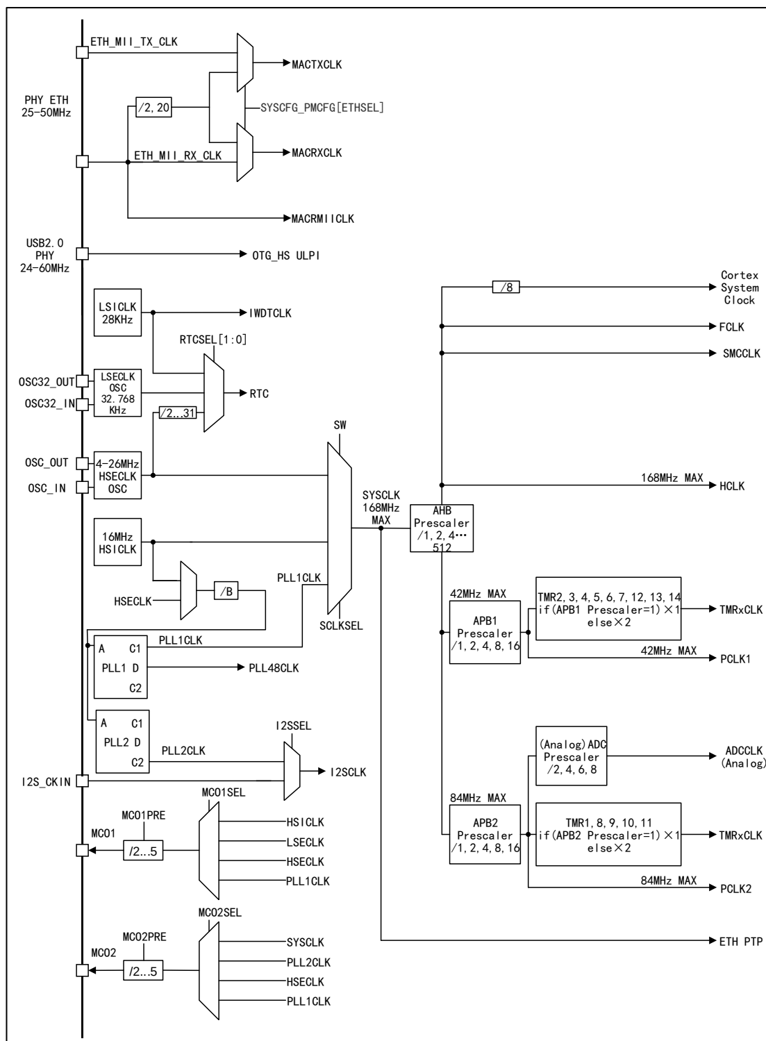
图 5 APM32A407xGT7 时钟树
