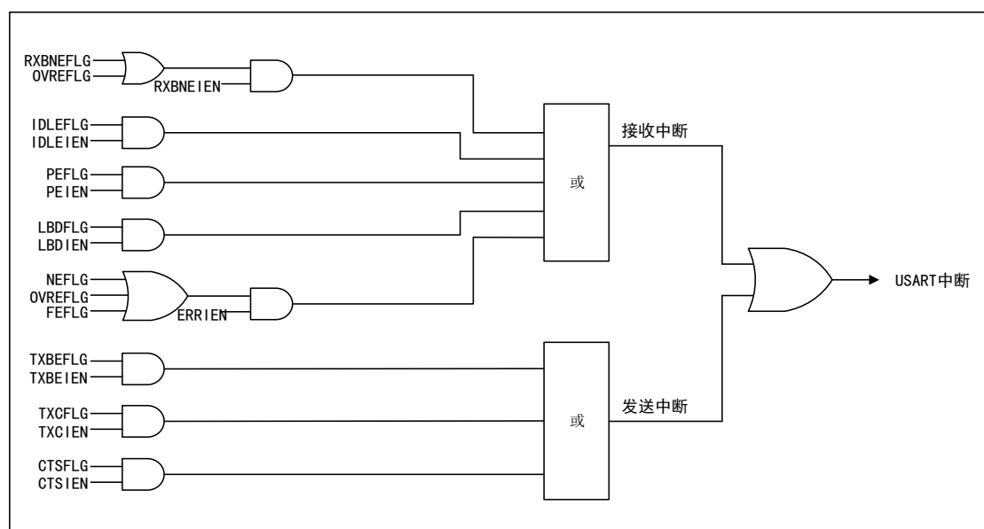
图 78 USART 中断映射
