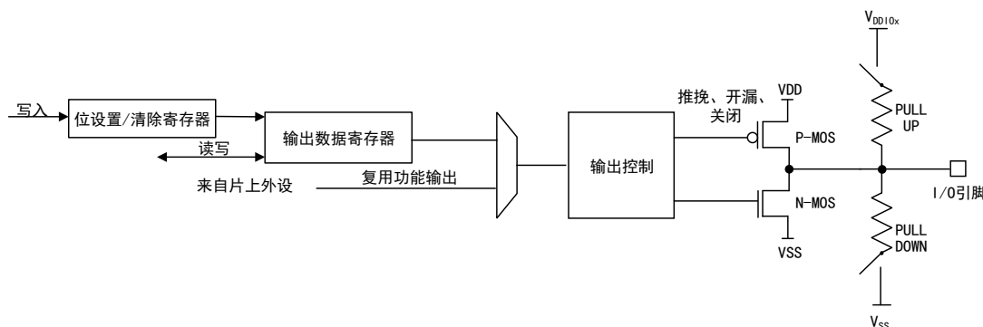
图 14 输出模式 I/O 结构
