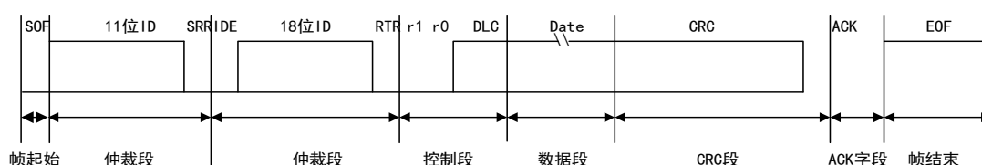
图 103 扩展数据帧
