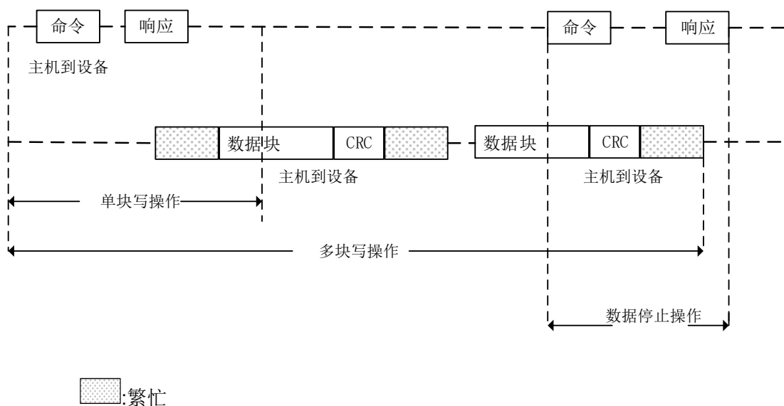
图 114 SDIO（多）数据块写操作
