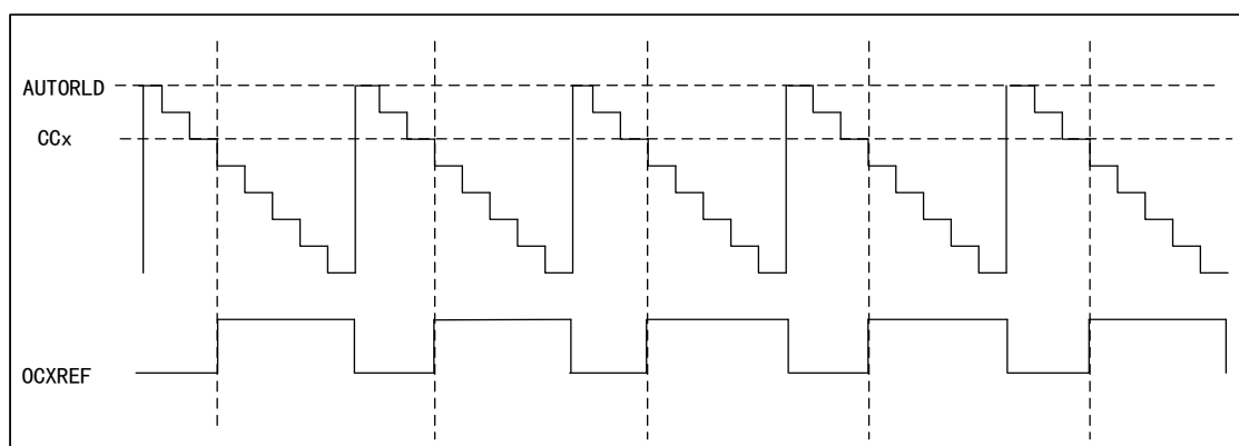
图 22 PWM1 向下计数模式的时序图
