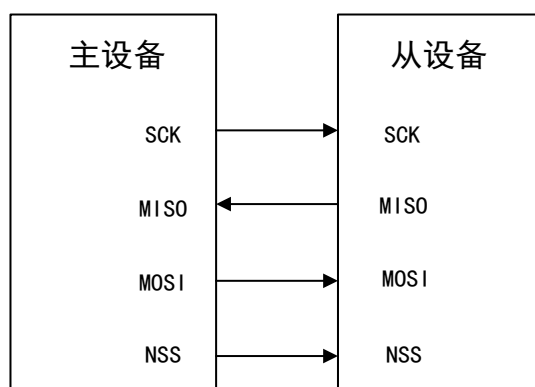
图 87 全双工模式连接
