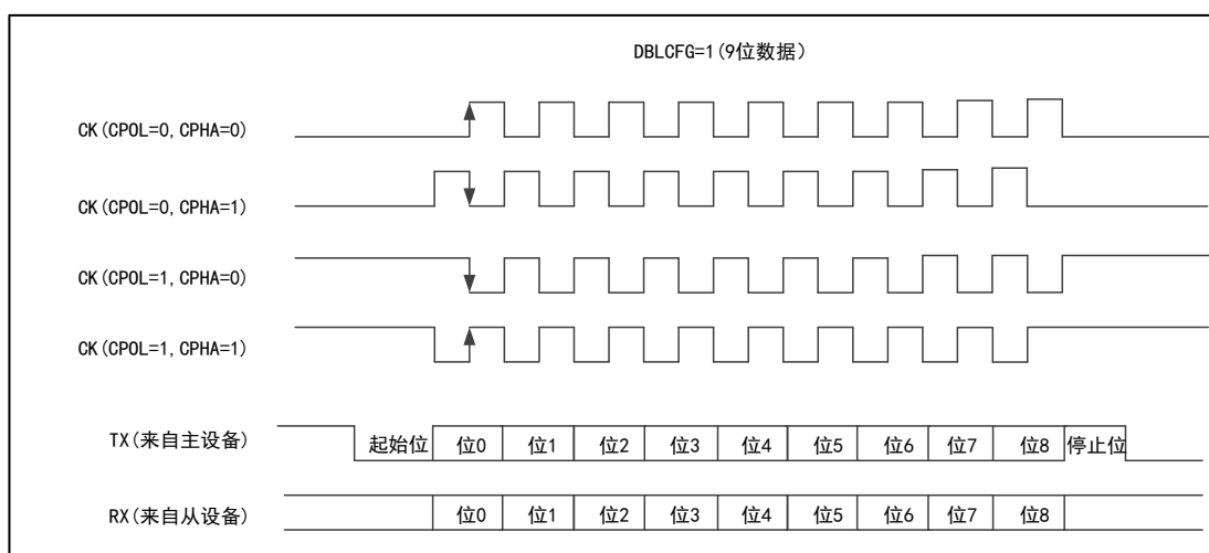
图 72 USART 同步发送时序图 (DBLCFG=1)
