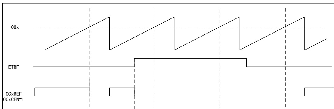
图 52 OCxREF 时序图
