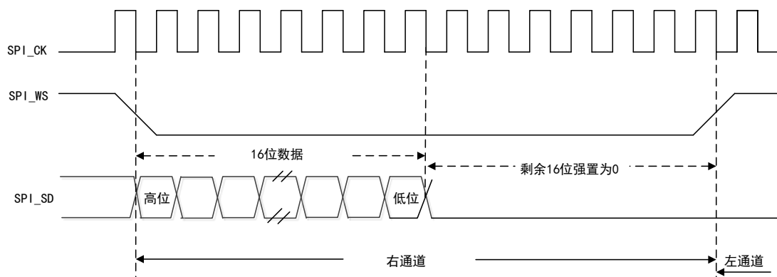
图 96 MSB 对齐标准波形（16 位扩展至 32 位）
