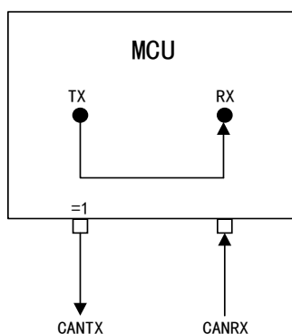
图 106 CAN 工作在静默环回模式
