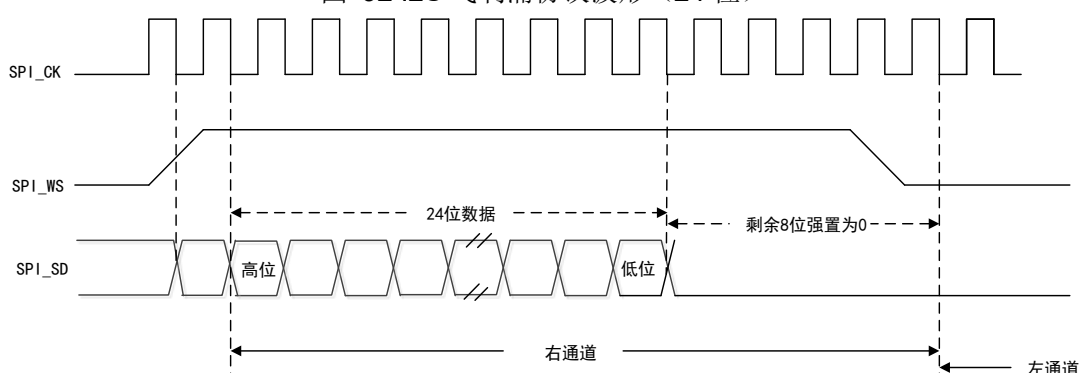
图 92 I2S 飞利浦协议波形（24 位）
