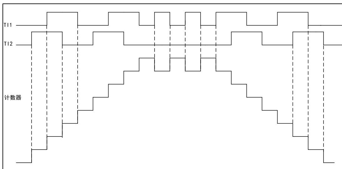
图 32 编码器模式下的计数器操作实例
