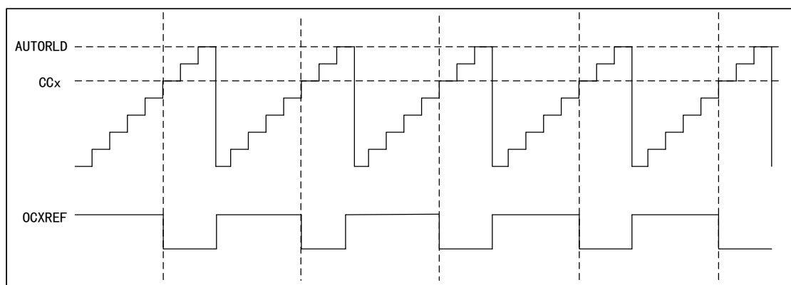
图 21 PWM1 向上计数模式的时序图
