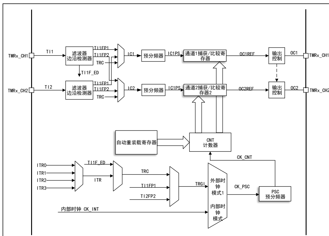
图 53 通用定时器 TMR9/12 结构框图
