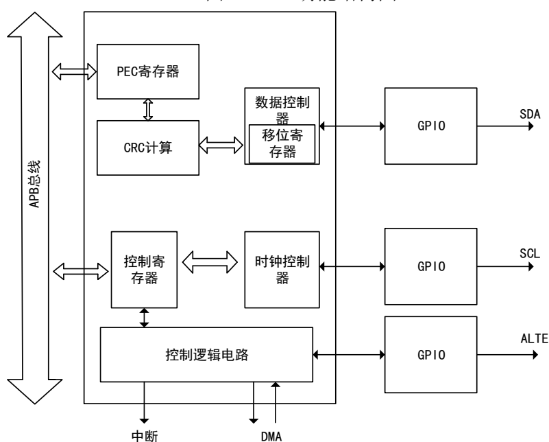
图 79 I2C 功能结构图
