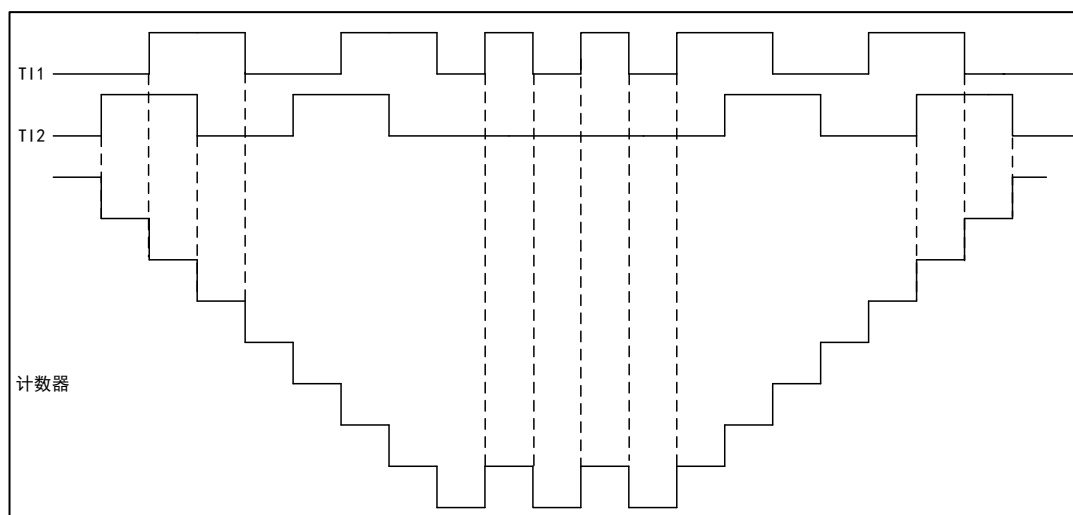
图 33 IC1FP1 反相的编码器接口模式实例
