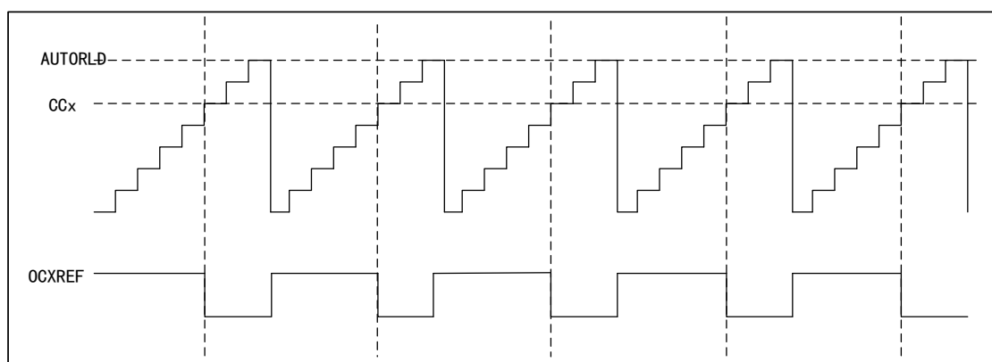
图 57 PWM1 向上模式的时序图
