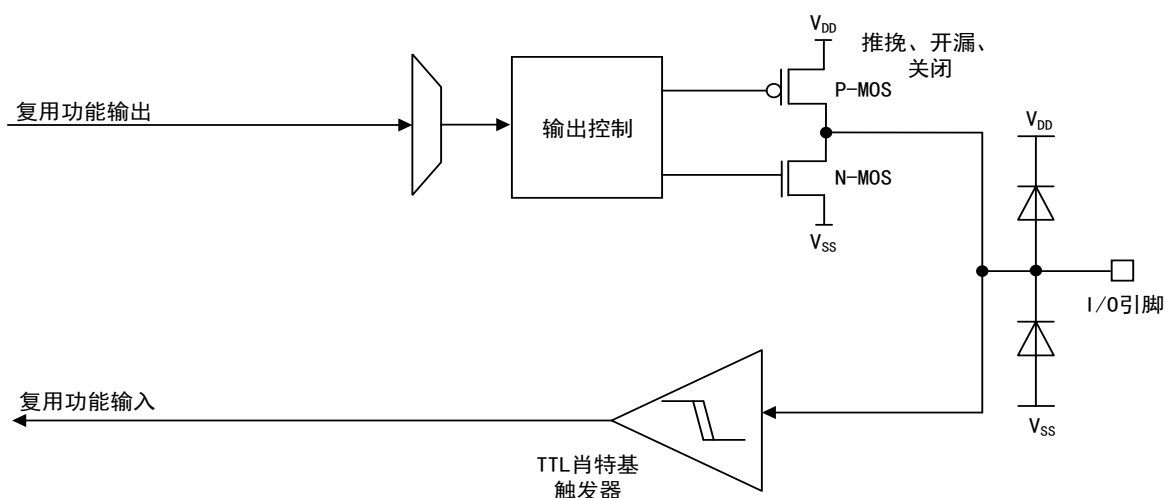
图 15 复用模式 I/O 结构
