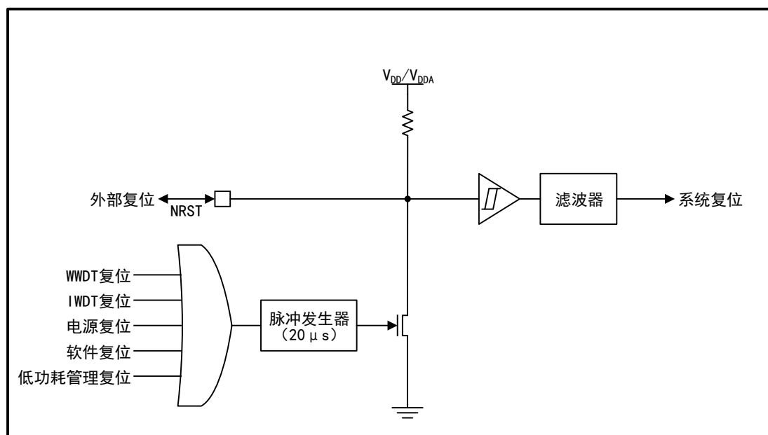
图 3 “系统复位”复位电路
