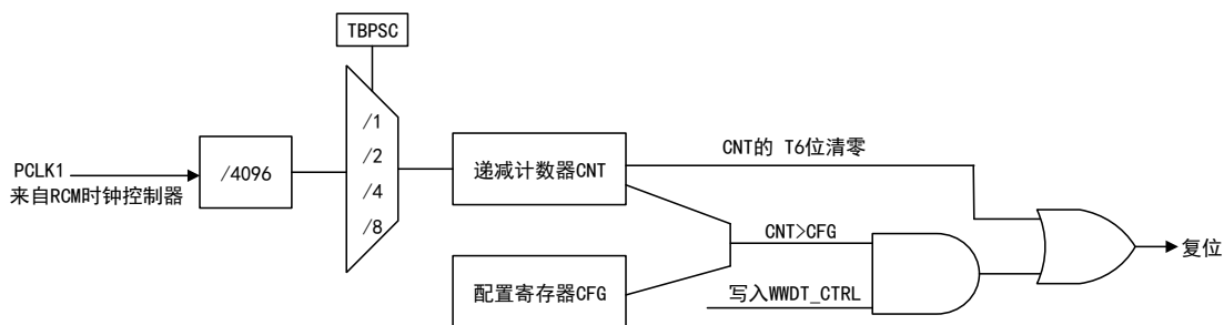
图 63 窗口看门狗结构框图
