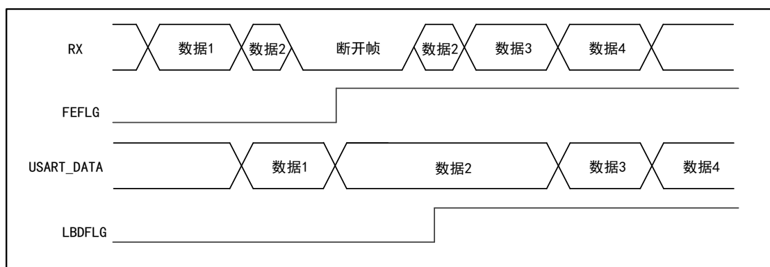
图 74 数据发送状态检测断开帧
