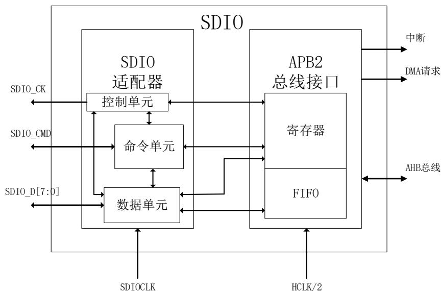
图 111 SDIO 结构框图如图
