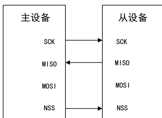
图 88 半双工模式连接（主机用来接收，从机用来发送）
