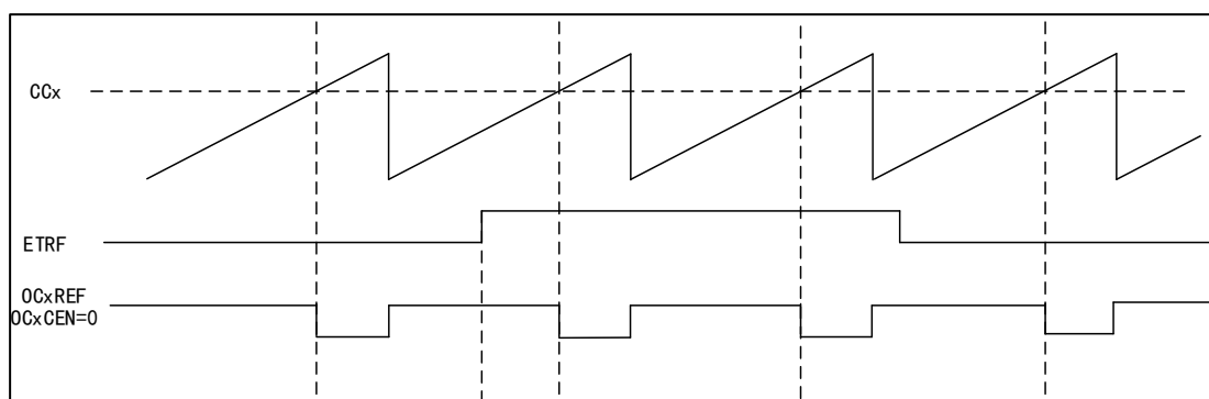
图 35 OCxREF 时序图
