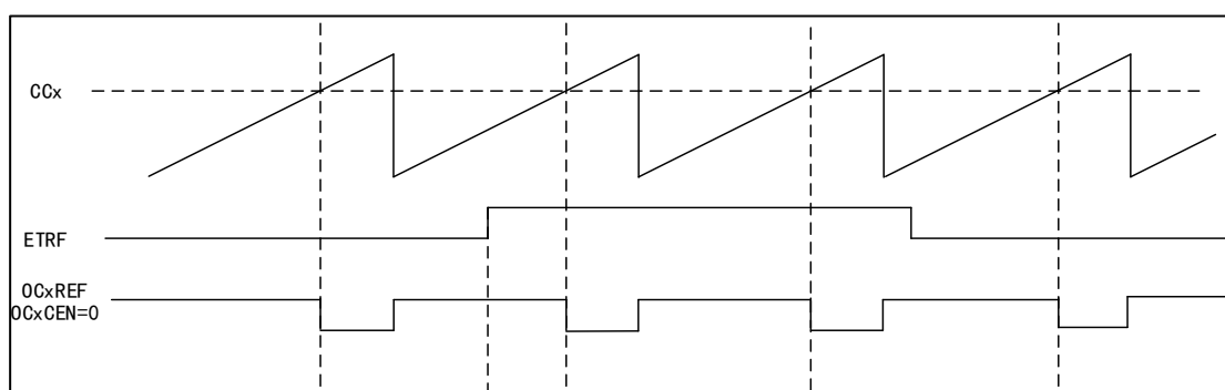
图 51 OCxREF 时序图
