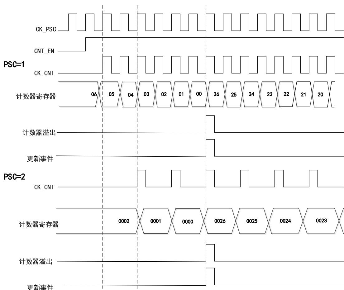
图 18 向下计数模式下，分频因子为 1 或 2 的时序图
