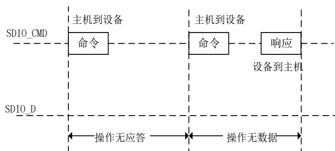
图 112 SDIO “无响应”和“无数据”操作
