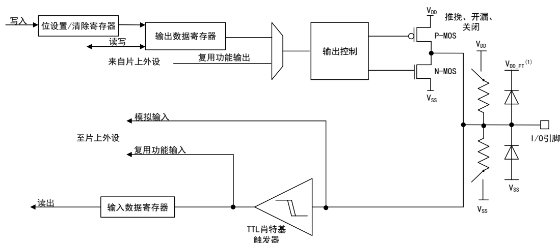
图 12 5 伏兼容 GPIO 结构框图
