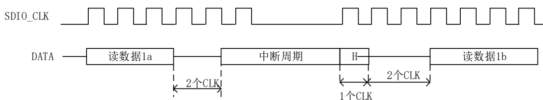
图 118 通过停止 SDIO_CLK 的读等待操作
