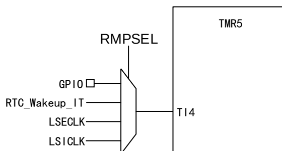
图 6 TMR5 测量时钟频率电路图
