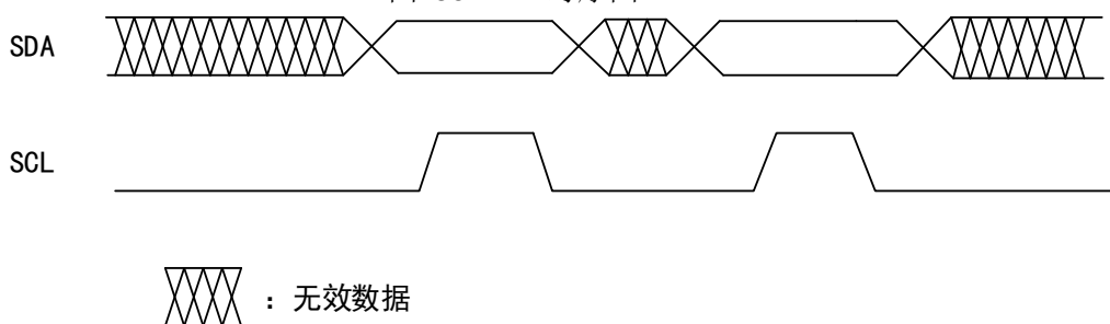
图 83 SDA 时序图
