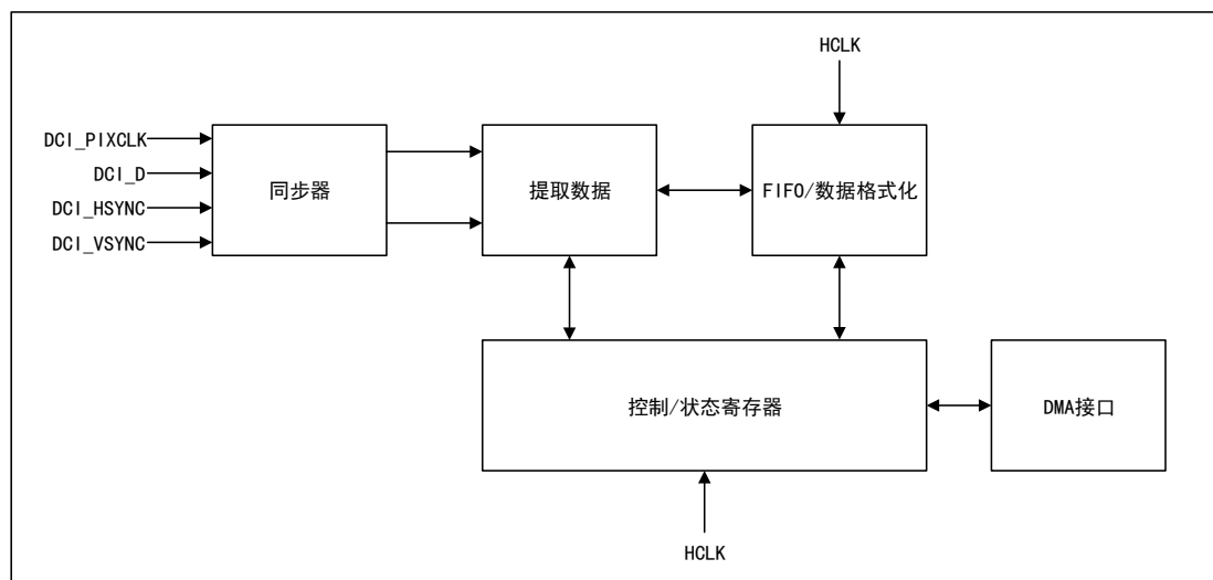
图 66DCI 结构框图
