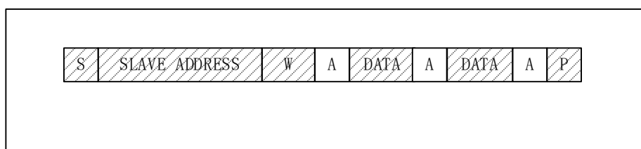
图 82 主机写数据到从机
