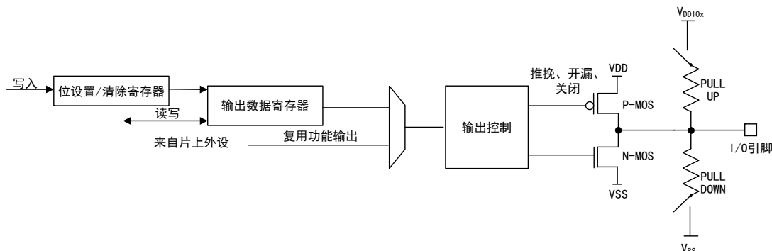
图 15 输出模式 I/O 结构
