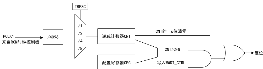
图 64 窗口看门狗结构框图
