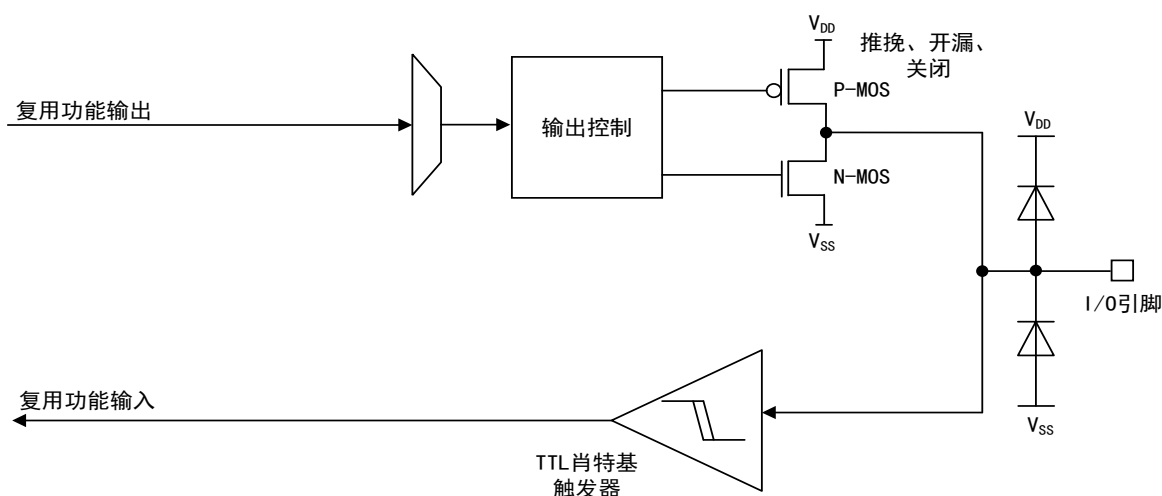
图 16 复用模式 I/O 结构
