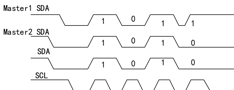
图 87 SDA 时序图
