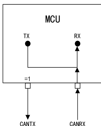
图 105 CAN 工作在静默模式
