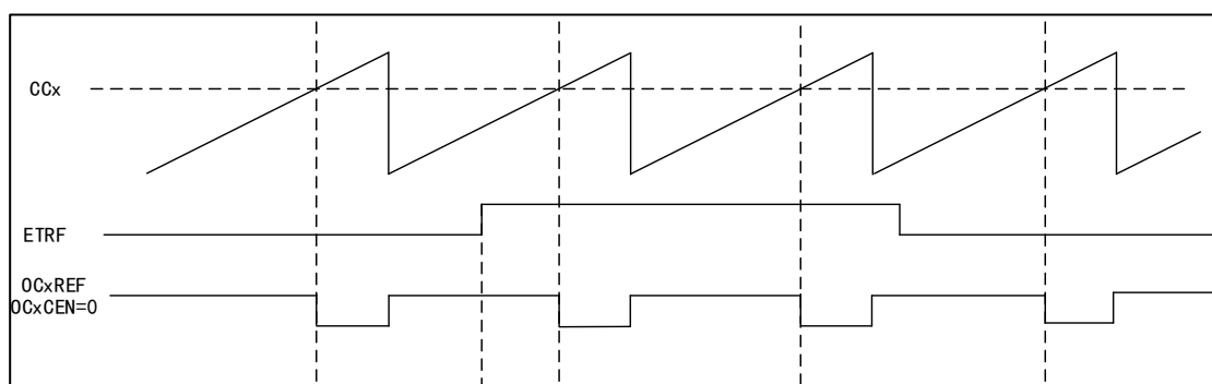
图 52 OCxREF 时序图
