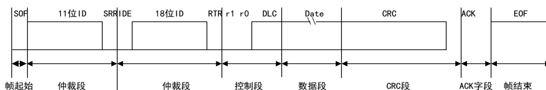
图 104 扩展数据帧
