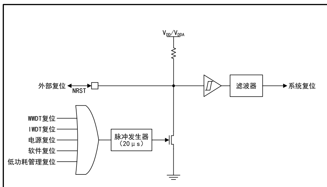
图 4 “系统复位”复位电路
