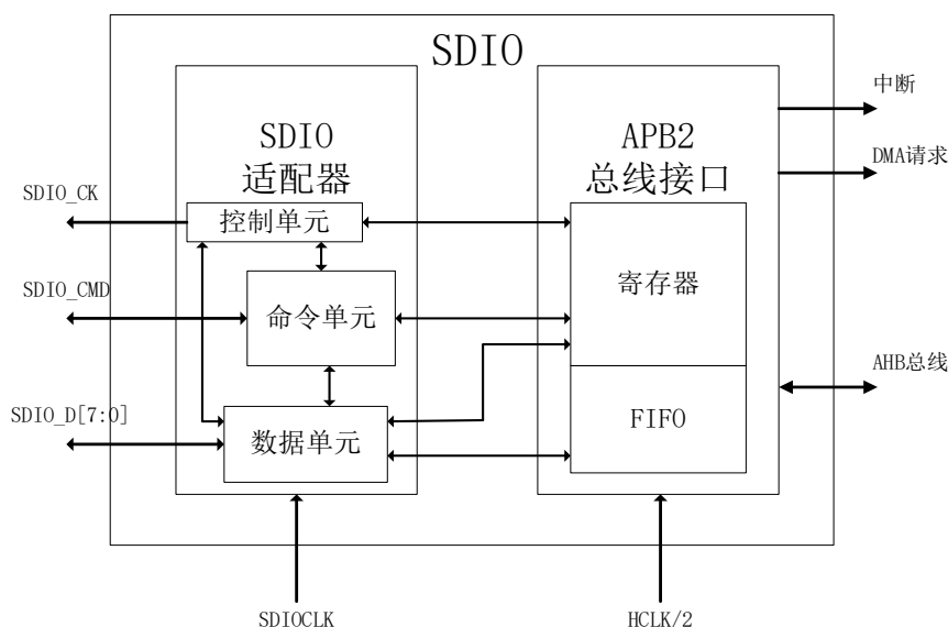
图 112 SDIO 结构框图如图
