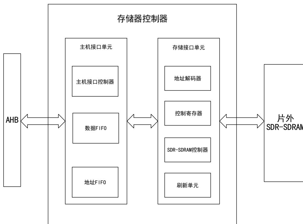
图 3 DMC 结构框图
