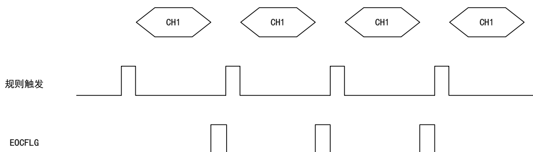
图 120 单次转换模式时序图
