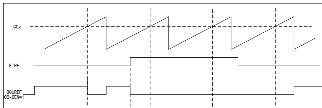
图 37 OCxREF 时序图
