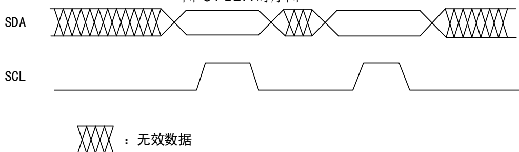
图 84 SDA 时序图
