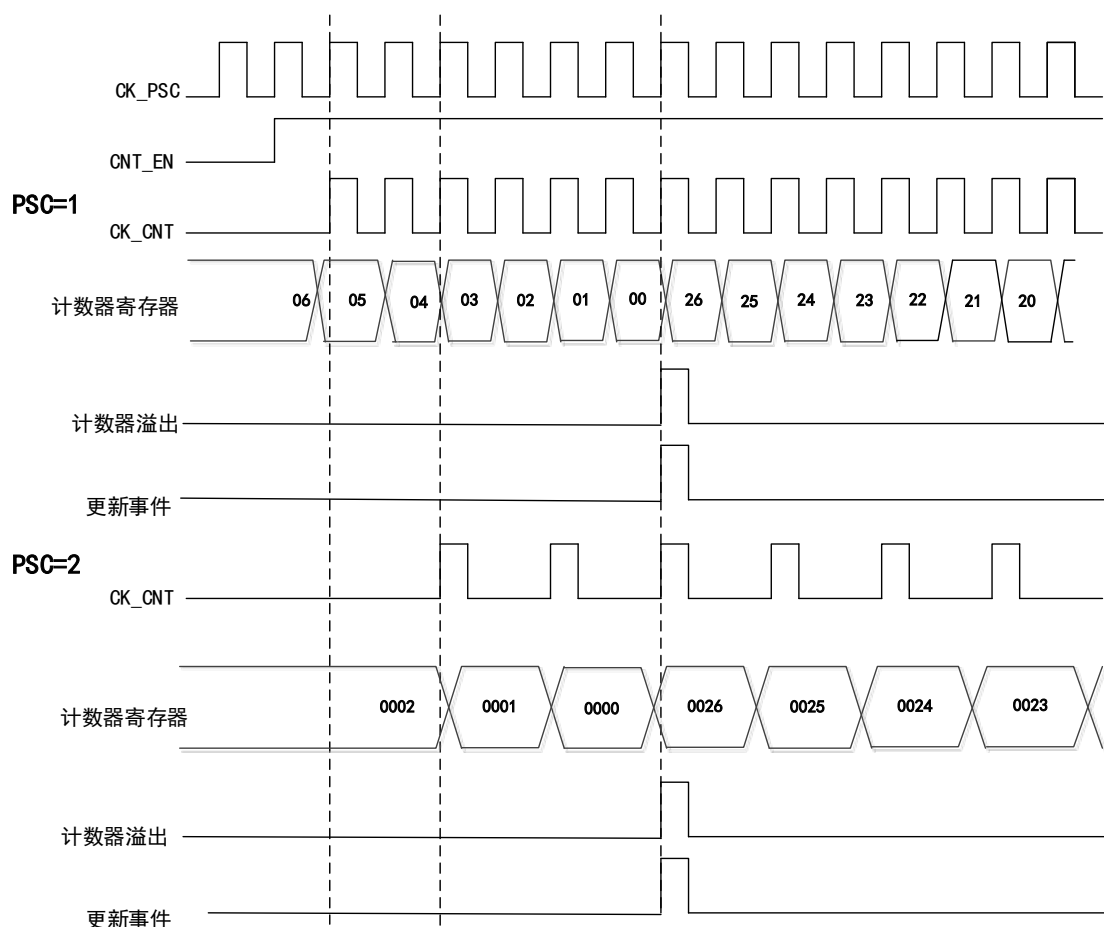
图 40 向下计数模式下，分频因子为 1 或 2 的时序图
