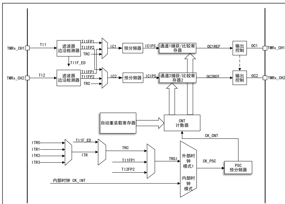
图 54 通用定时器 TMR9/12 结构框图
