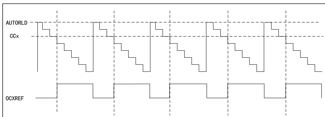
图 23 PWM1 向下计数模式的时序图
