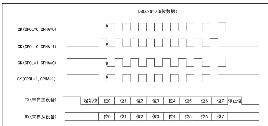
图 72 USART 同步发送时序图 (DBLCFG=0)
