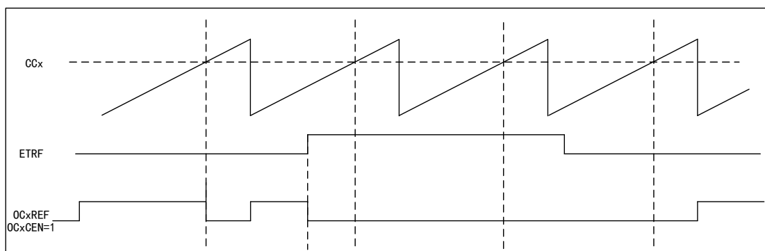
图 53 OCxREF 时序图
