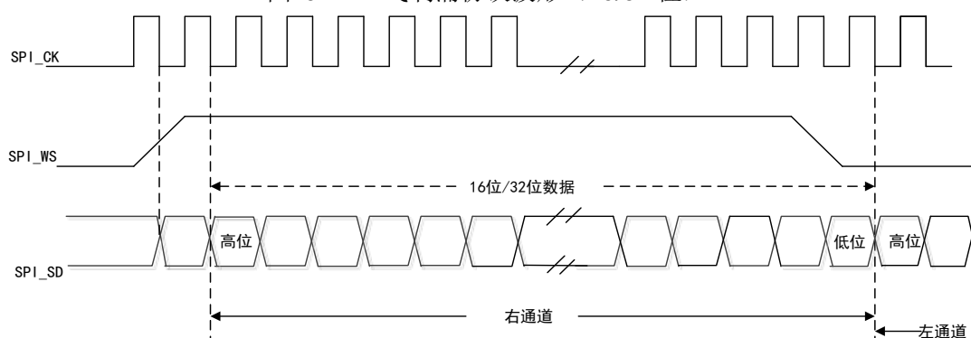
图 92 I2S 飞利浦协议波形（16/32 位）
