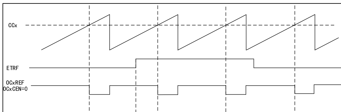
图 36 OCxREF 时序图
