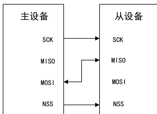
图 91 双向线连接
