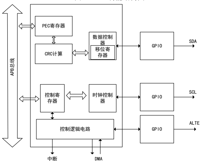
图 80 I2C 功能结构图
