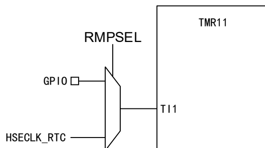
图 8 TMR11 测量时钟频率电路图
