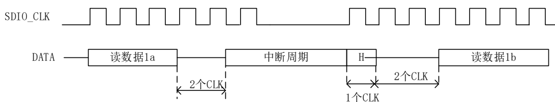
图 119 通过停止 SDIO_CLK 的读等待操作
