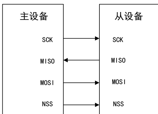
图 88 全双工模式连接
