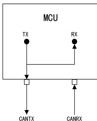
图 106 CAN 工作在环回模式
