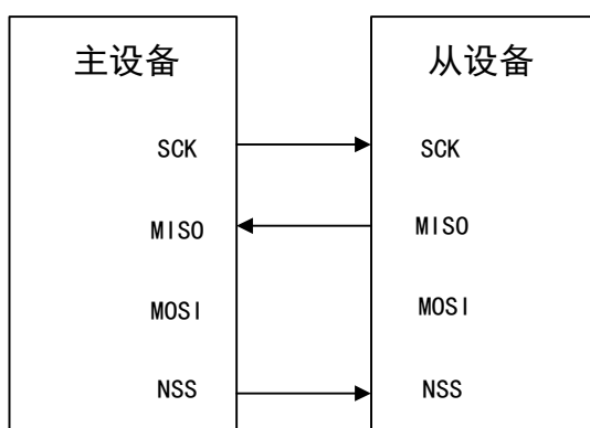
图 89 半双工模式连接（主机用来接收，从机用来发送）
