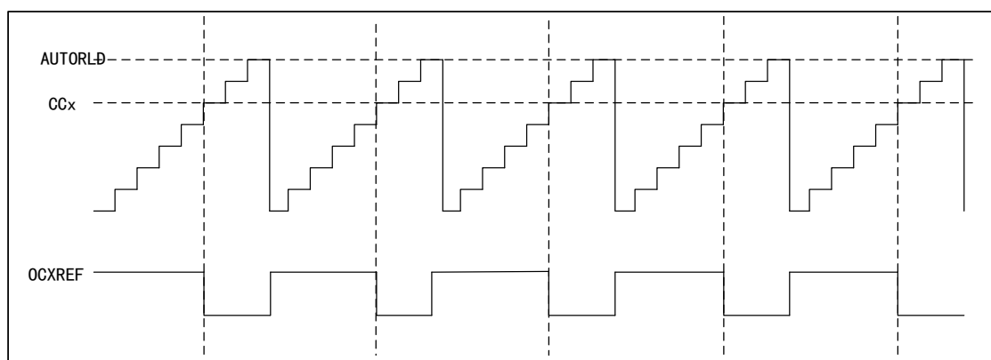
图 42 PWM1 向上计数模式的时序图
