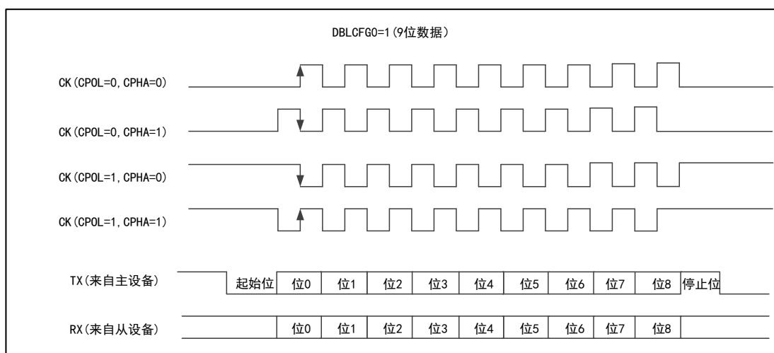
图 89 USART 同步传输时序图 (DBLCFG0=1)
