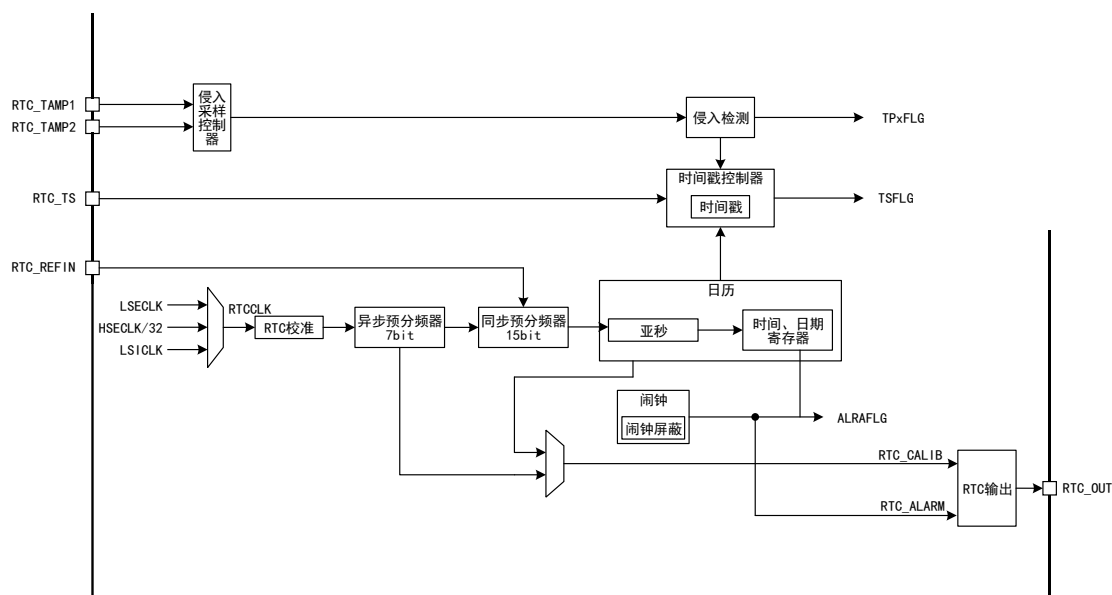
图 82 APM32F030x4x6x8 RTC 结构框图
