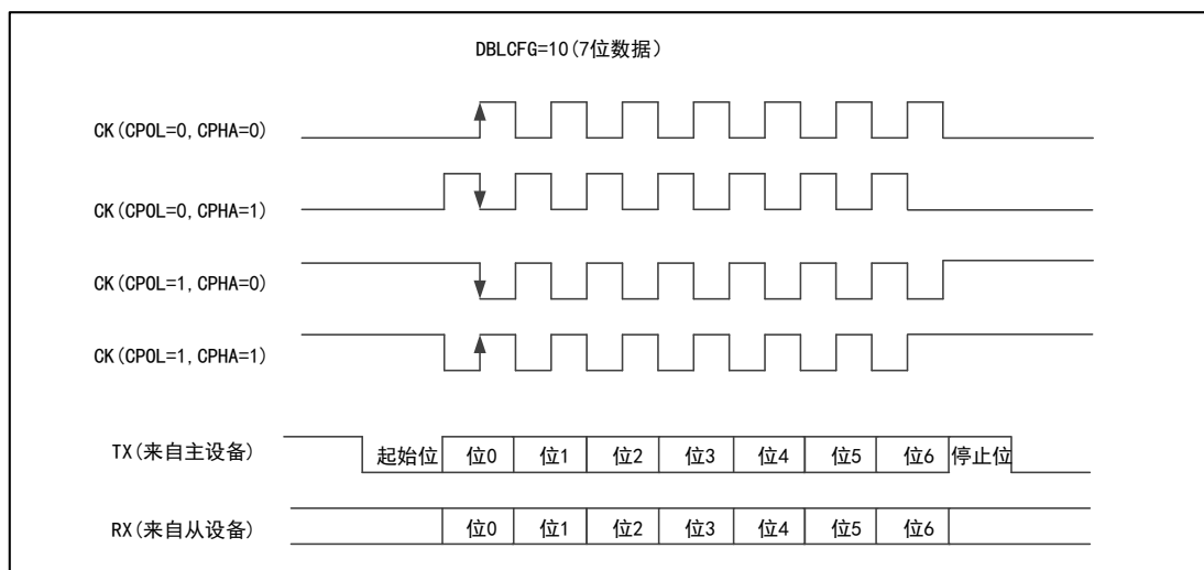
图 87 USART 同步传输时序图 (DBLCFG=10)
