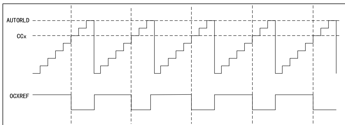
图 62 PWM1 向上计数模式的时序图
