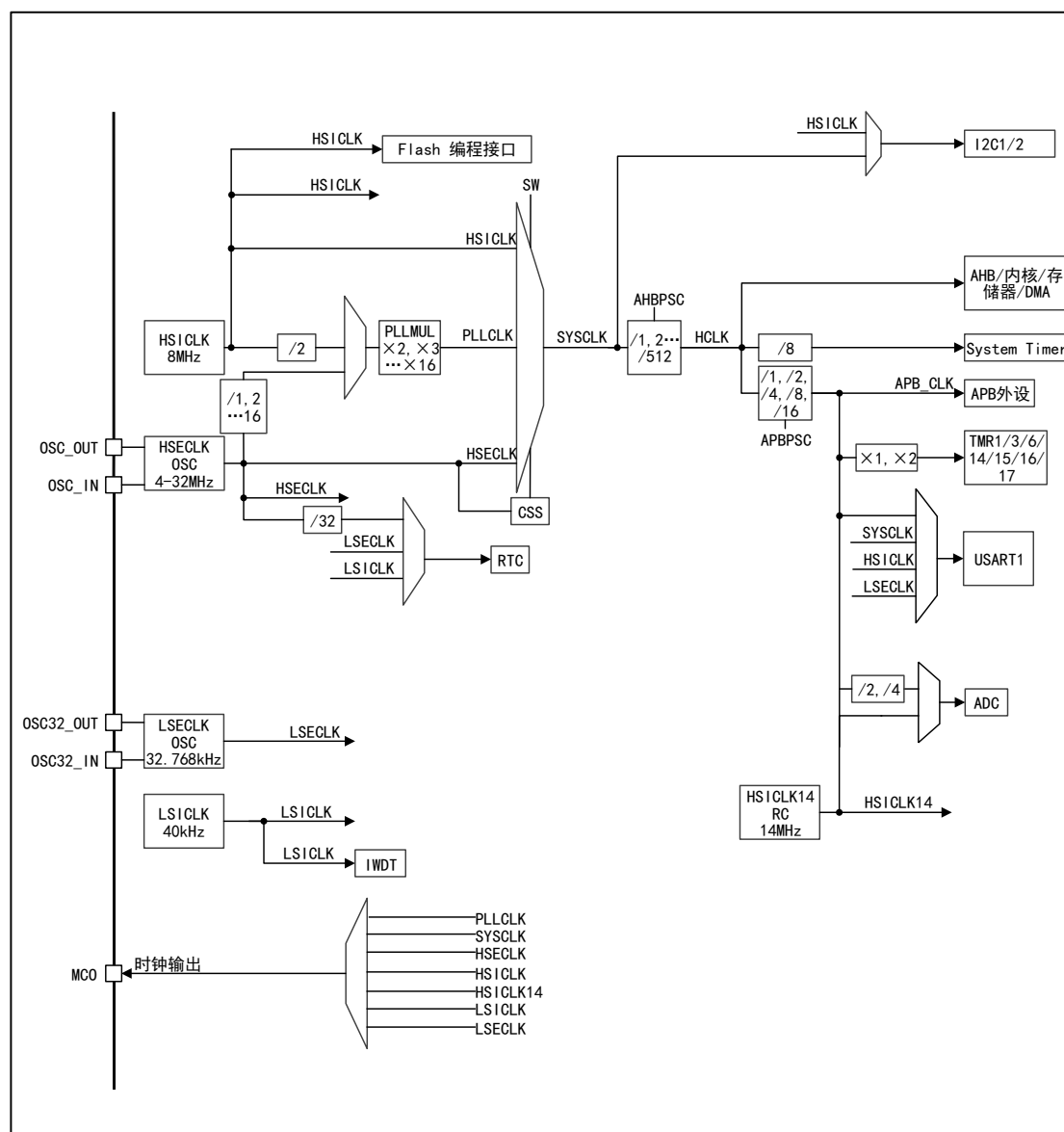
图 4 APM32F030x4x6x8xC 时钟树
