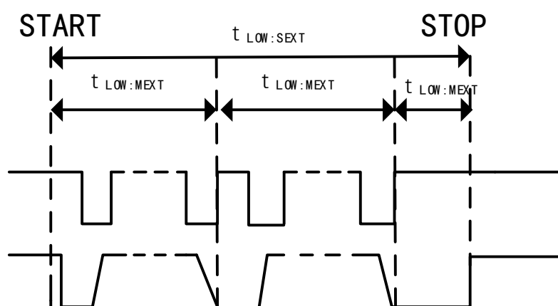
图 97 t_{\text{LOW:SEXT}} 与 t_{\text{LOW:MEXT}} 时间
