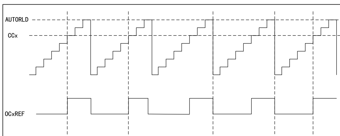
图 63 PWM2 向上计数模式的时序图
