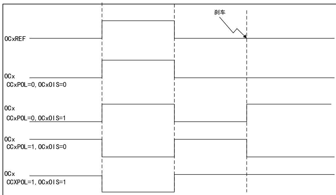
图 73 发生刹车事件的时序图
