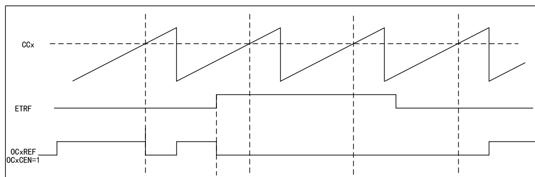
图 42 OCxREF 时序图
