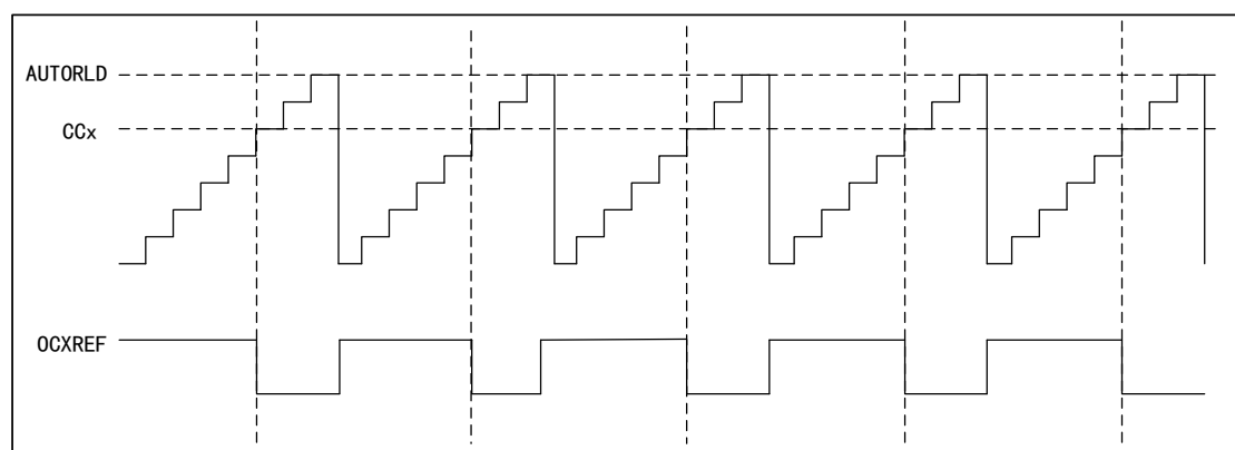
图 68 PWM1 向上计数模式的时序图
