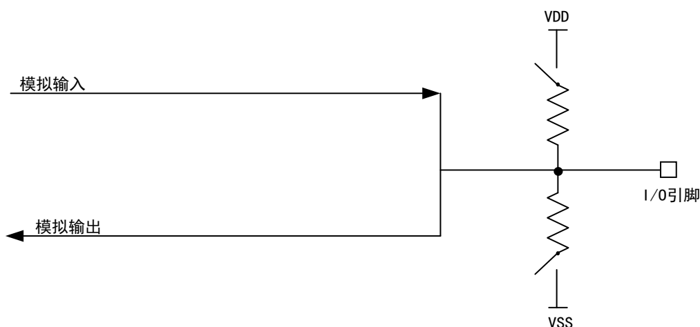
图 20 模拟功能 I/O 结构
