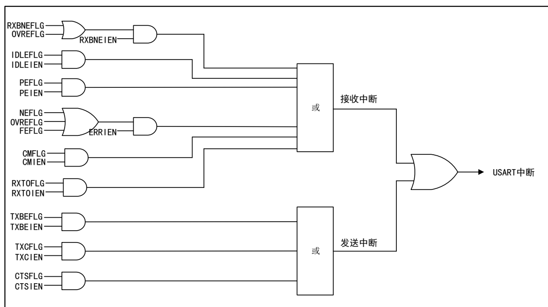
图 91 USART 中断映射
