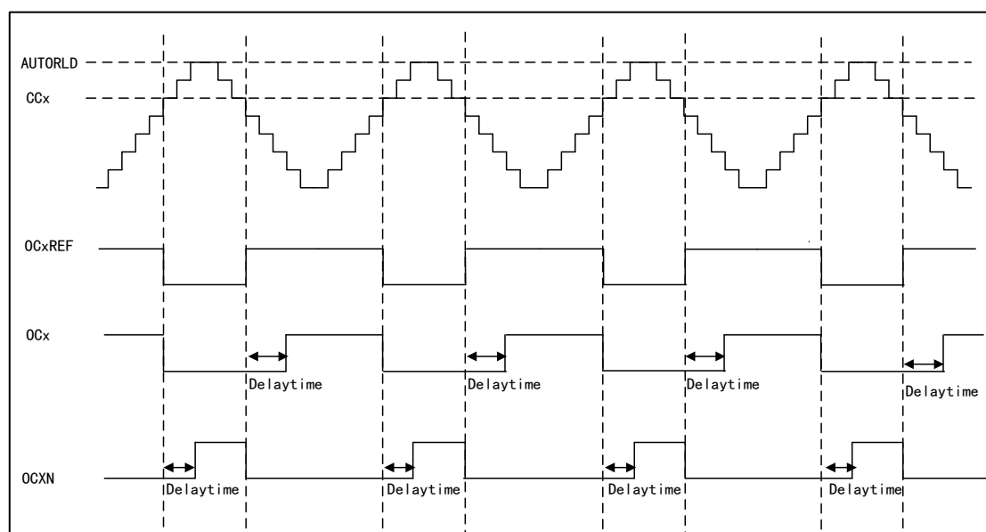
图 37 带死区插入的互补输出
