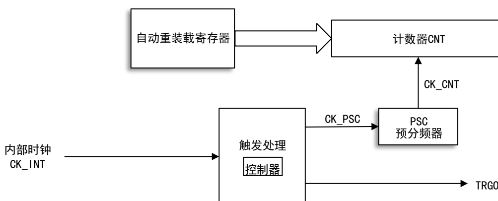
图 76 基本定时器结构框图
