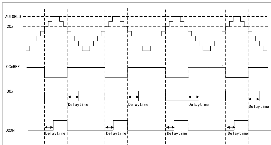
图 36 带死区插入的互补输出
