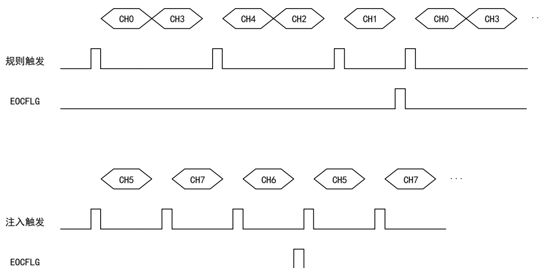
图 113 间断模式时序图
