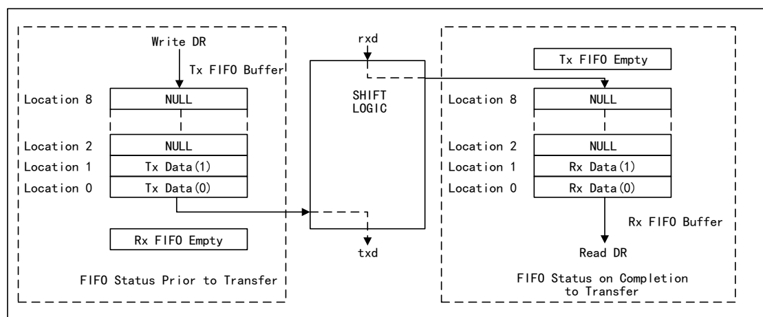
图 94 发送和接收状态下的 QSPI 传送 FIFO 状态
