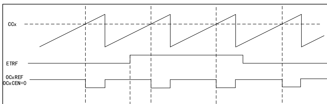
图 40 OCxREF 时序图
