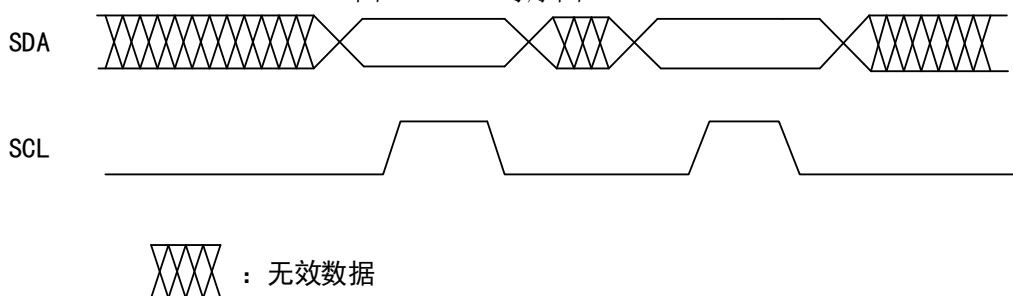
图 77 SDA 时序图
