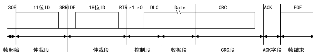
图 102 扩展数据帧
