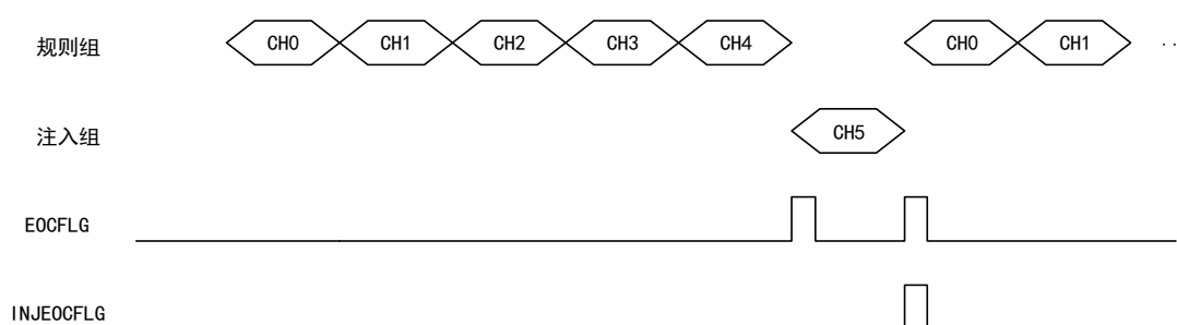
图 115 自动注入时序图
