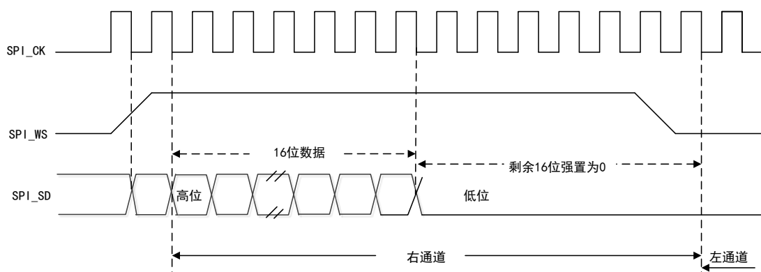
图 111 I2S 飞利浦协议波形（16 位扩展至 32 位）
