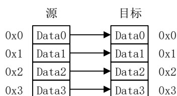
图 9 源为 8bits 目标为 8bits 的传输宽度
