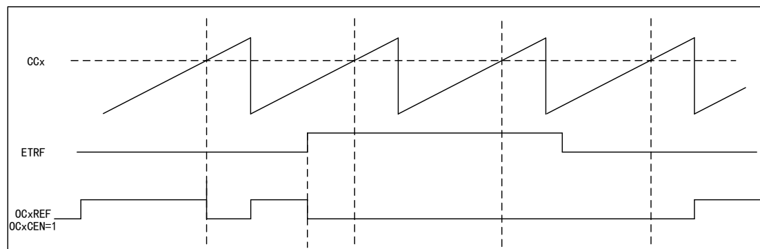
图 40 OCxREF 时序图
