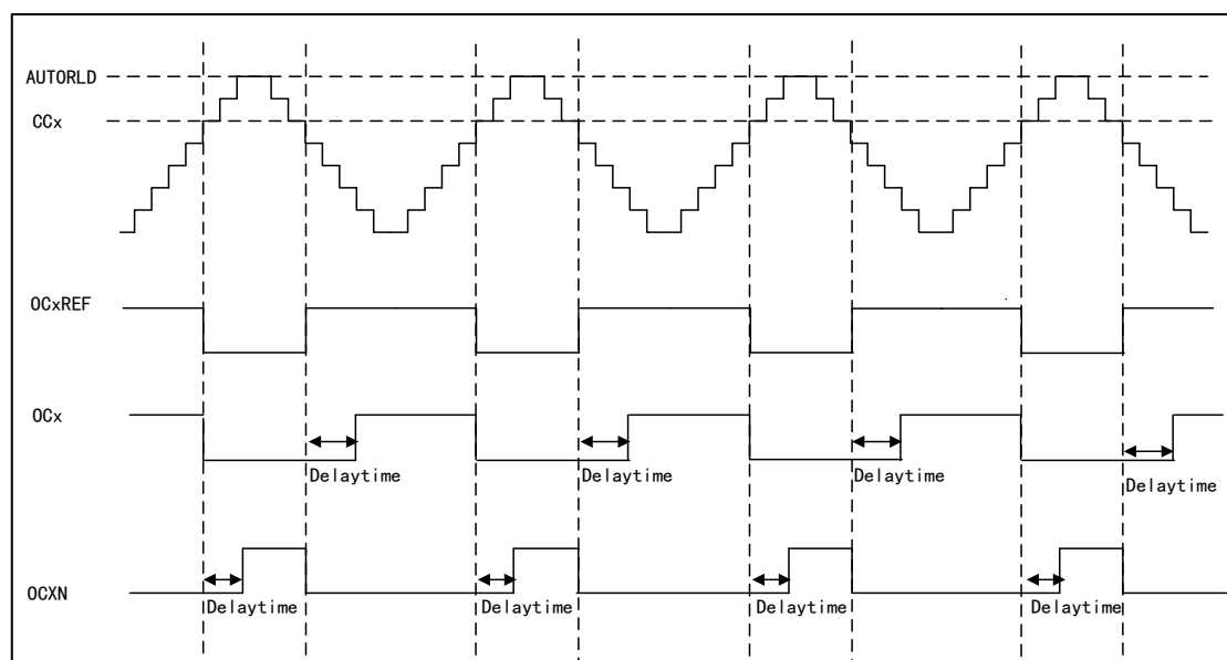
图 76 带死区插入的互补输出
