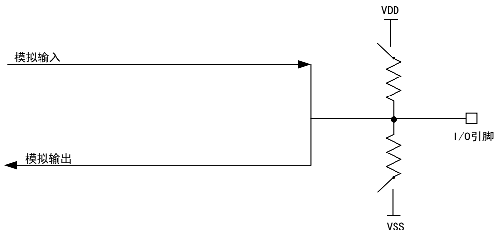
图 21 模拟功能 I/O 结构
