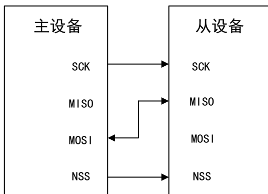
图 107 单工模式连接（主机用来接收，从机用来发送）
