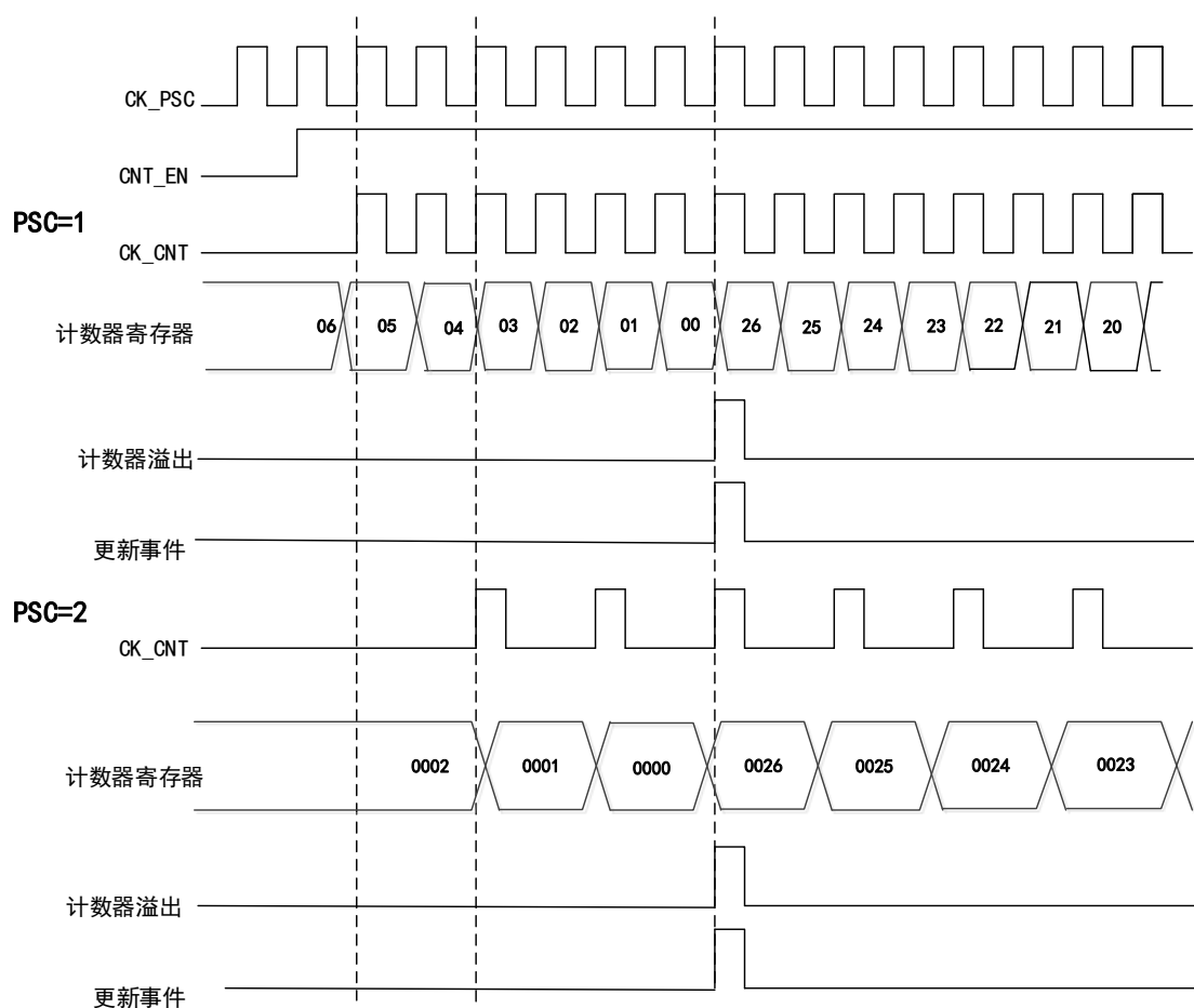
图 63 向下计数模式下，分频因子为 1 或 2 的时序图
