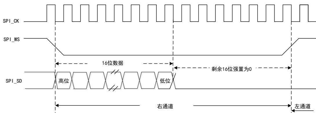
图 114 MSB 对齐标准波形（16 位扩展至 32 位）
