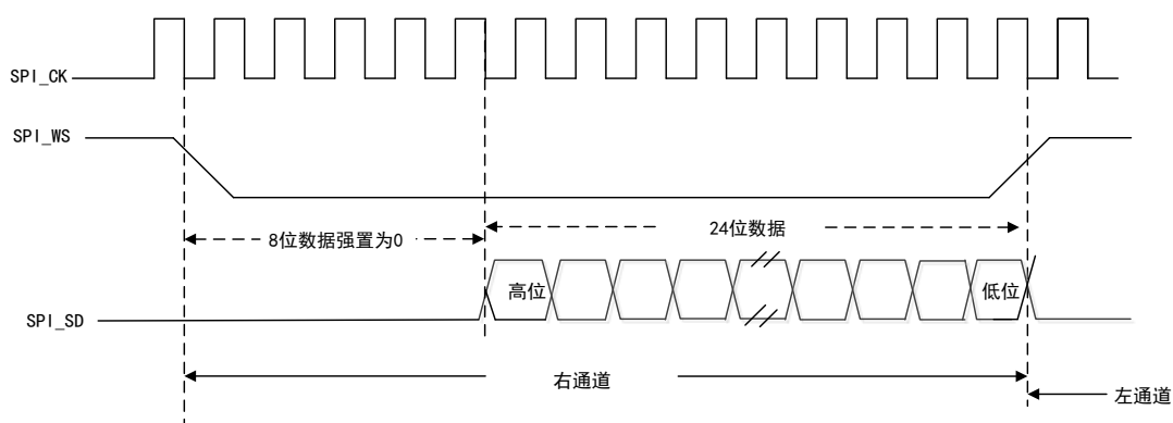
图 116 LSB 对齐标准波形（24 位数据）
