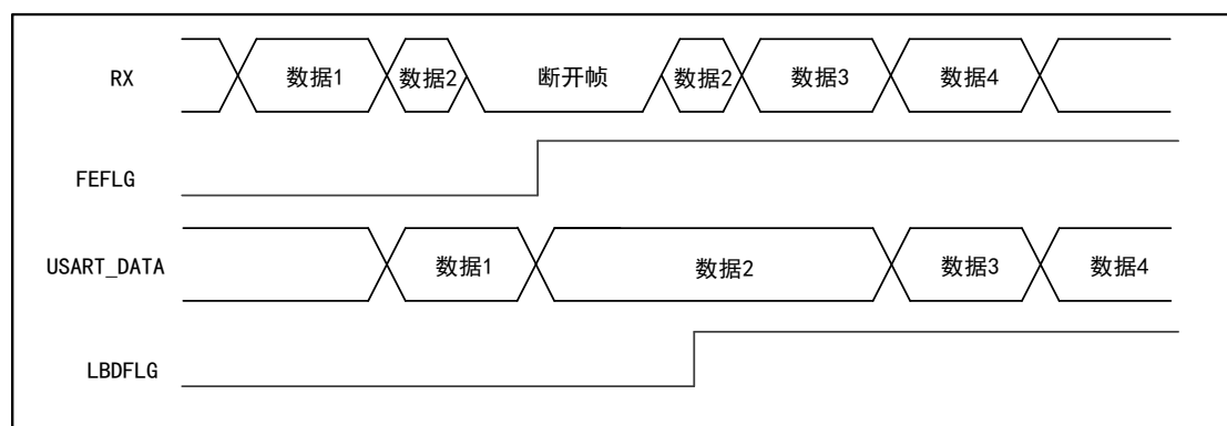
图 94 数据传输状态检测断开帧
