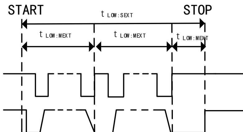
图 104 t_{\text{LOW:SEXT}} 与 t_{\text{LOW:MEXT}} 时间
