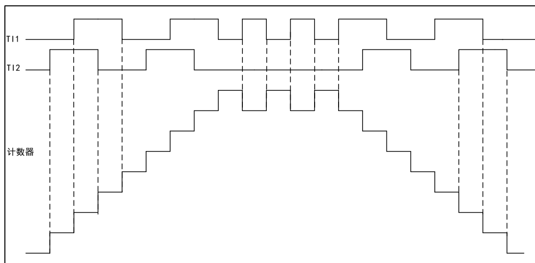
图 77 编码器模式下的计数器操作实例
