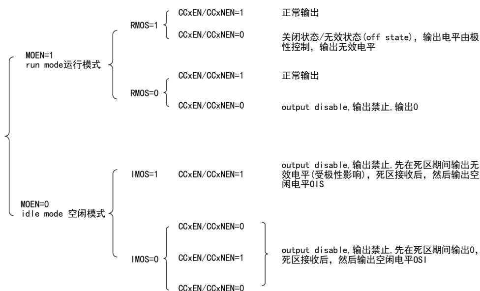
图 57 影响输出波形的寄存器结构关系
