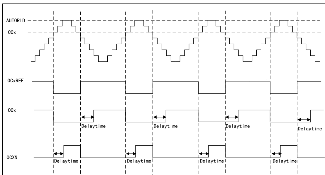
图 59 带死区插入的互补输出
