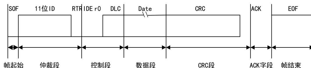
图 120 标准数据帧
