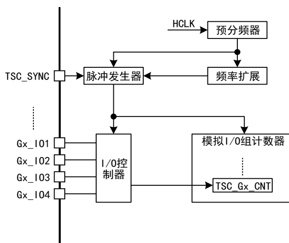
图 133 结构框图
