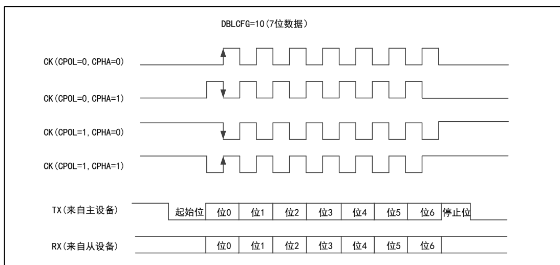
图 90 USART 同步传输时序图（DBLCFG=10）
