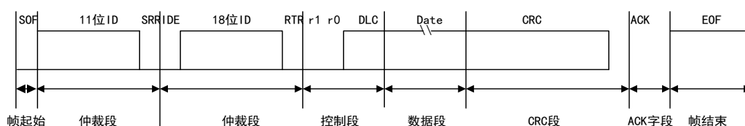
图 121 扩展数据帧
