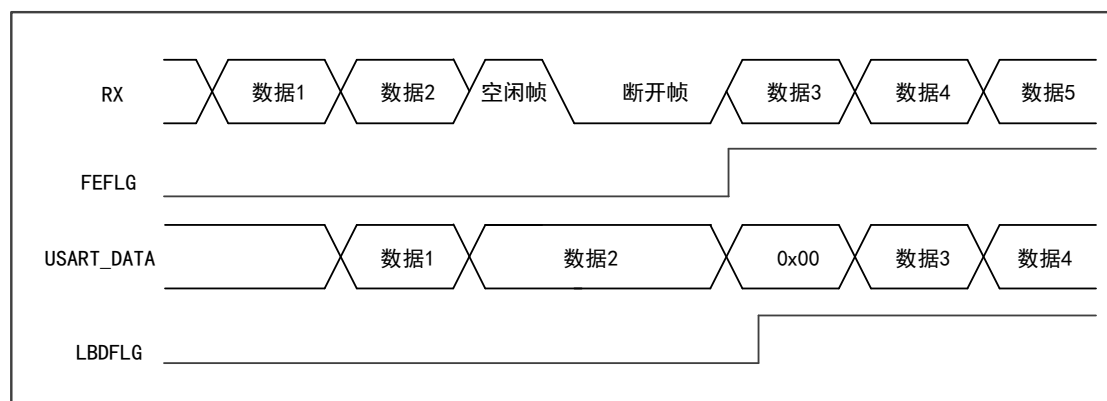
图 93 空闲状态检测断开帧
