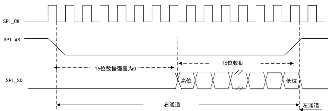
图 117 LSB 对齐标准下（16 位扩展至 32 位）
