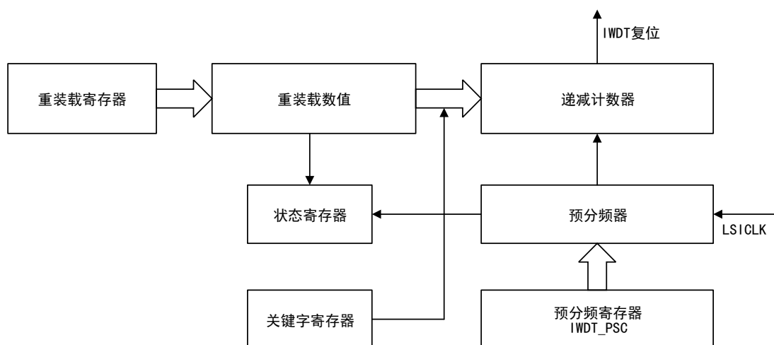
图 83 独立看门狗框图
