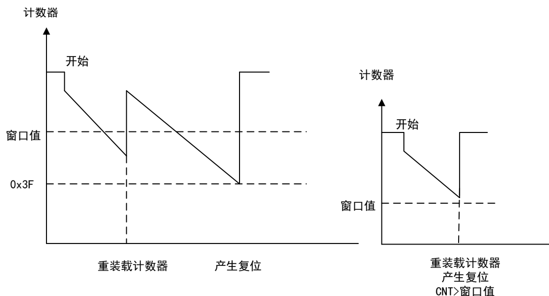
图 85 窗口看门狗时序图
