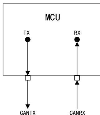
图 125 CAN 工作在正常模式
