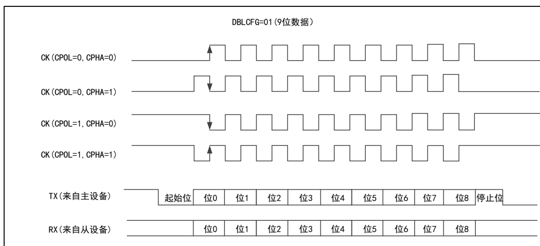
图 92 USART 同步传输时序图 (DBLCFG=01)
