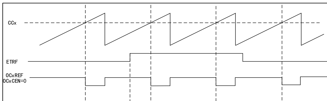
图 80 OCxREF 时序图
