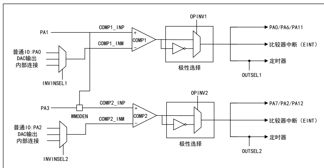
图 134 COMP 结构框图
