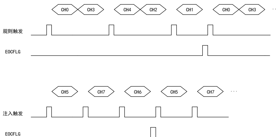
图 106 间断模式时序图
