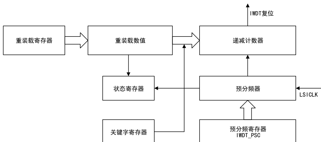
图 88 独立看门狗结构框图
