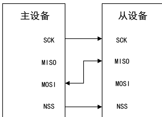
图 111 单工模式连接（主机用来接收，从机用来发送）
