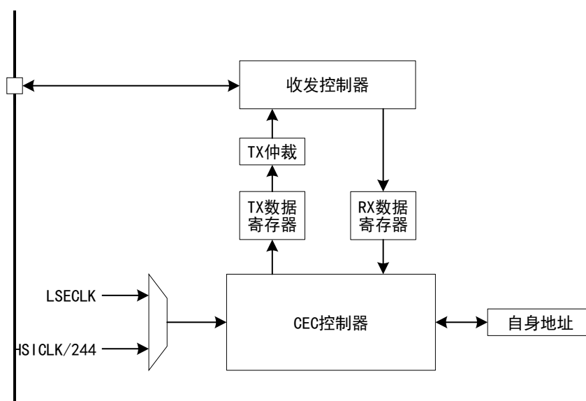
图 124 CEC 结构框图
