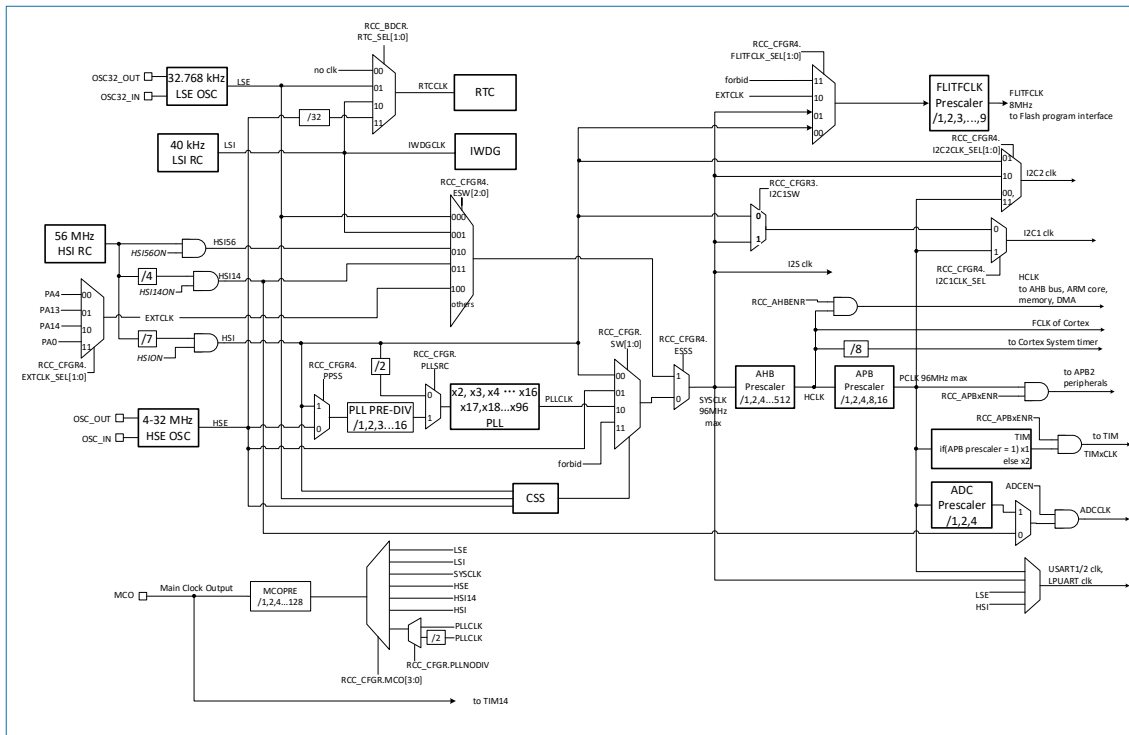
图 3-4 HK32F072x8xB 时钟树
