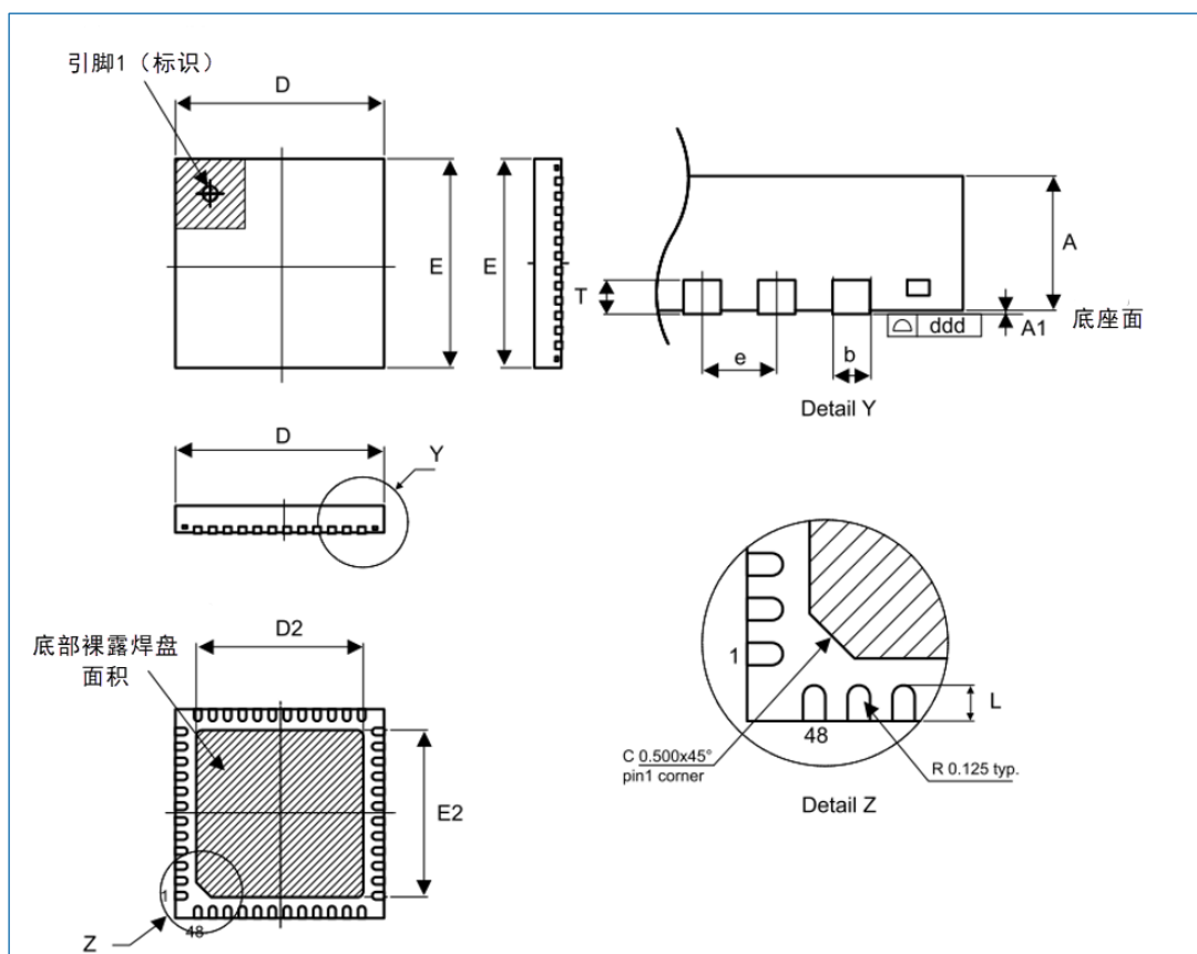
图 7-3 QFN48 封装尺寸图
