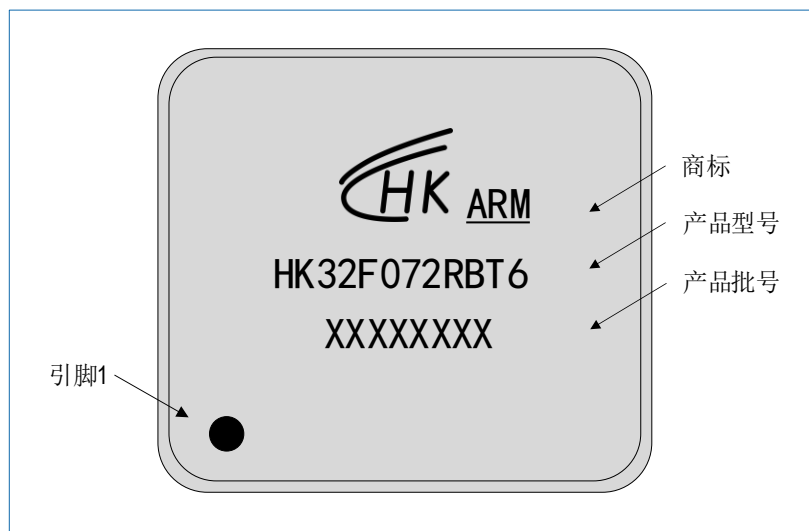
图 7-4 LQFP64 HK32F072RBT6 丝印示例
