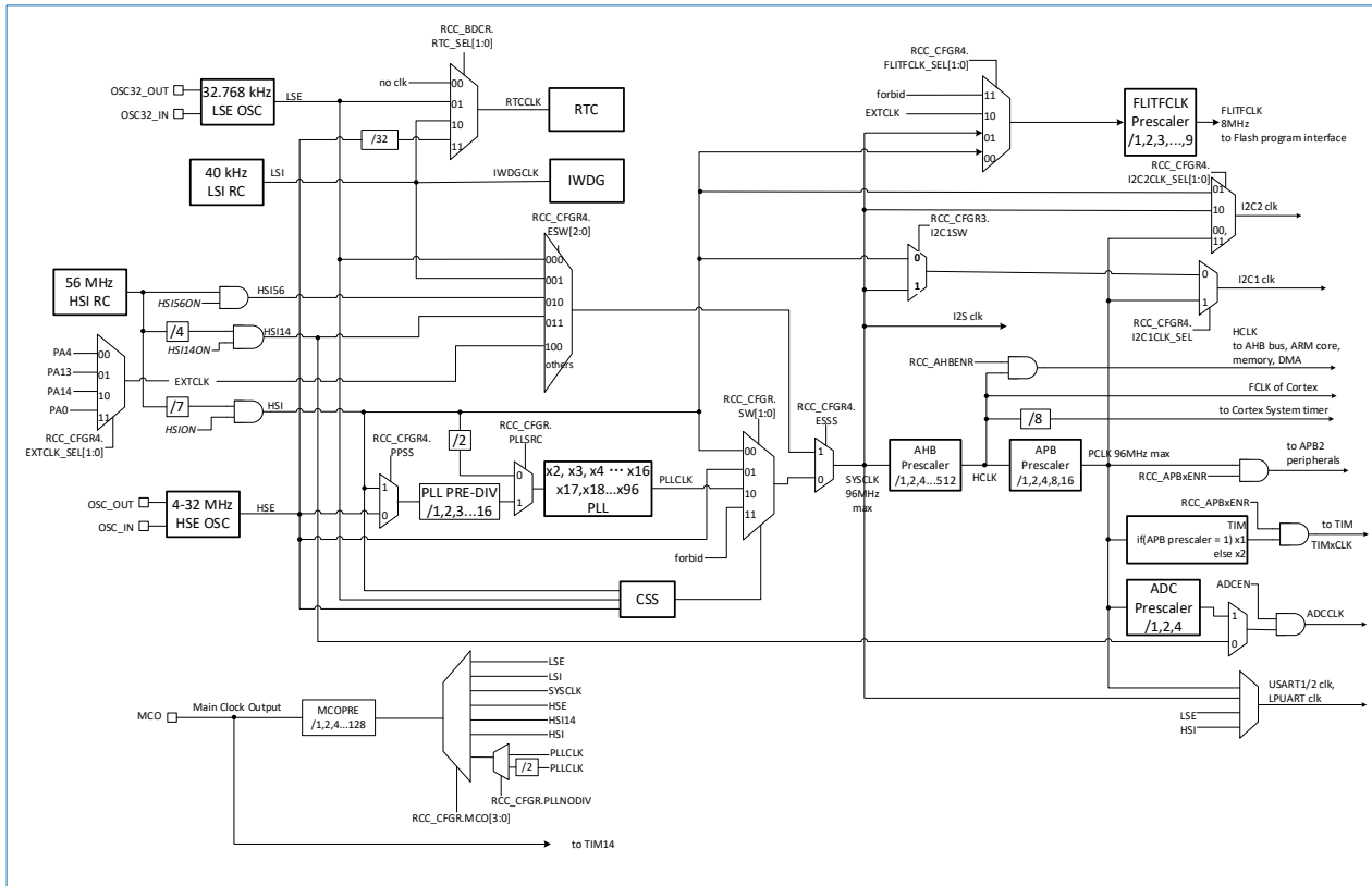
图 3-4 HK32F04AxxxxA 时钟树
