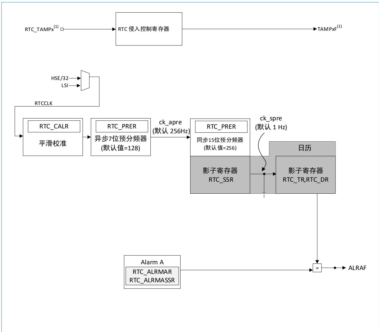
图 25-1 RTC 框图
