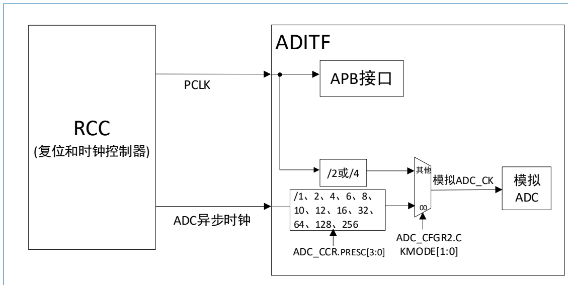
图 11-5 ADC 时钟图
