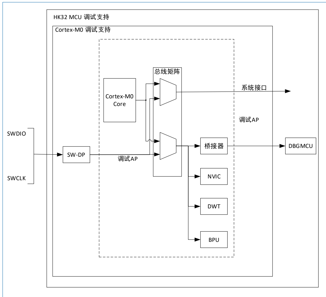
图 27-1 HK32C105 MCU 和 Cortex®-M0 级调试支持框图
