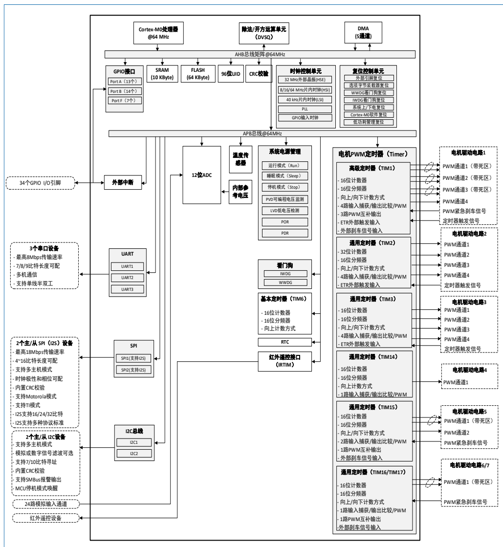
图 2-1 HK32C105S8T7 功能框图
