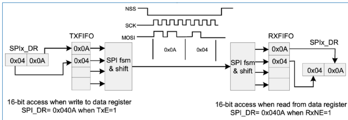
图 24-9 发送和接收 FIFO 中的数据组包
