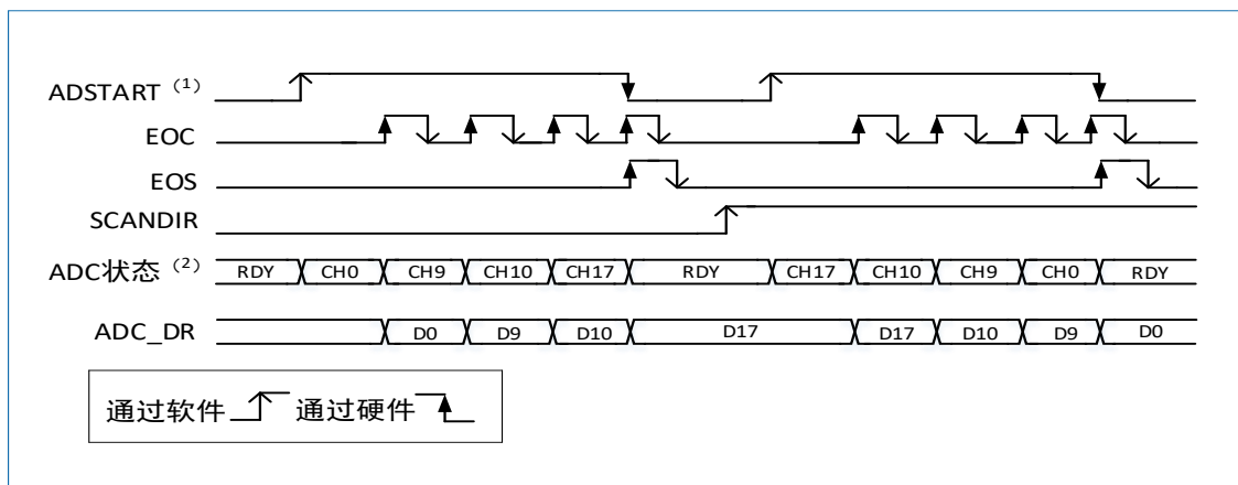
图 11-9 单序列转换, 软件触发
