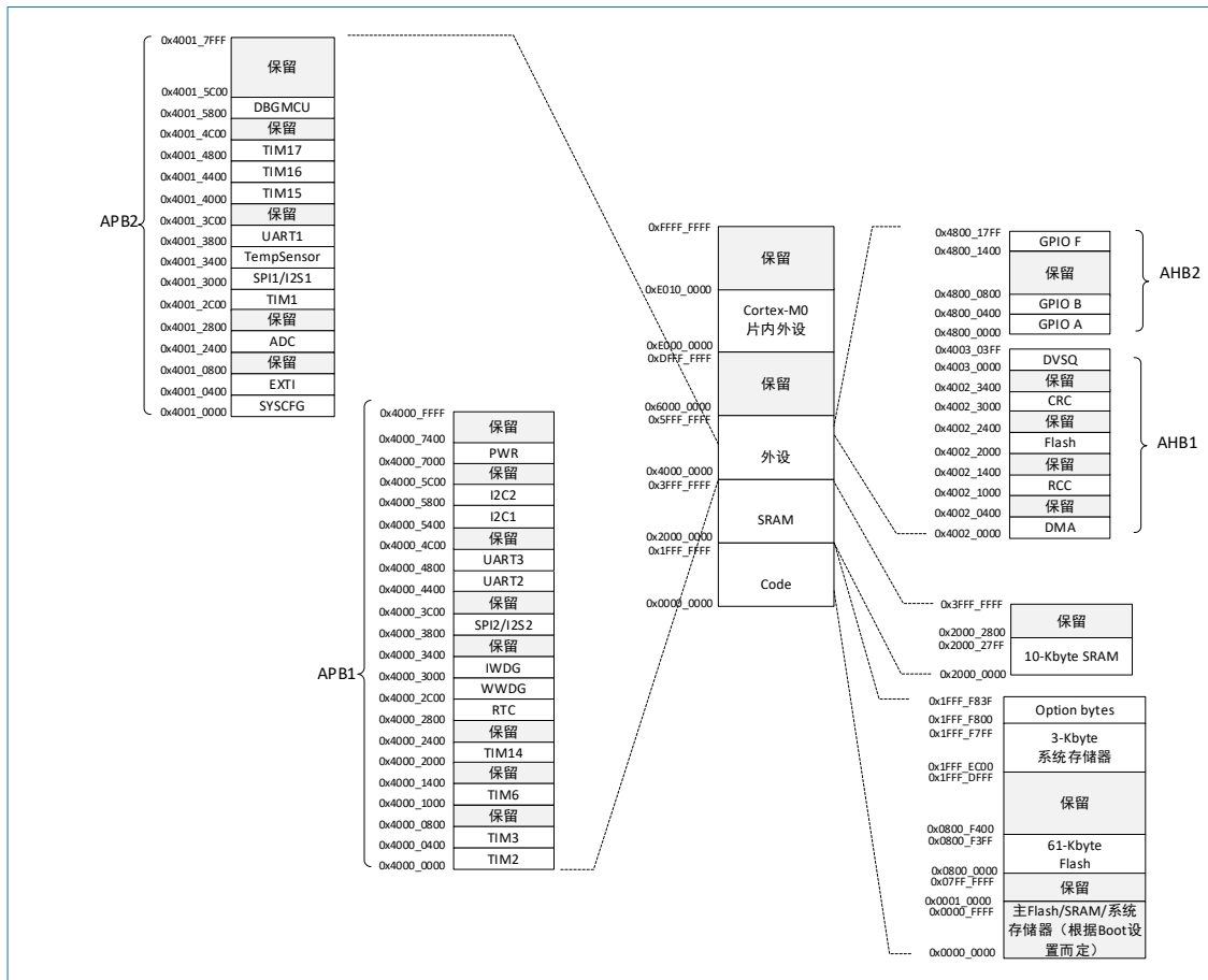
图 2-2 HK32C105S8T7 存储器映射
