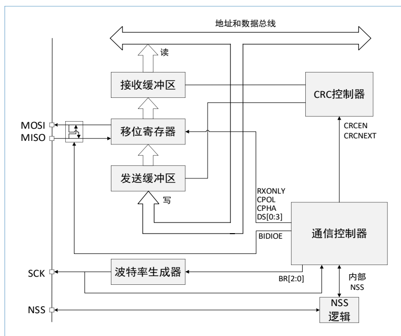
图 24-1 SPI 框图
