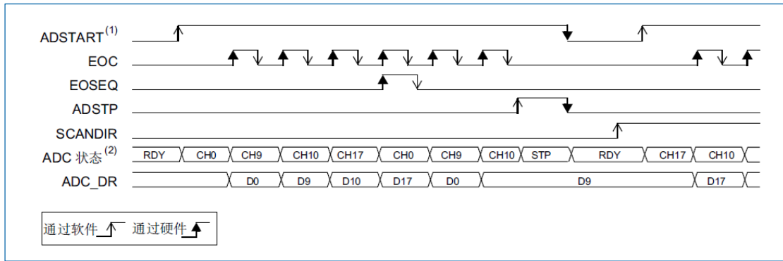
图 11-10 连续序列转换，软件触发
