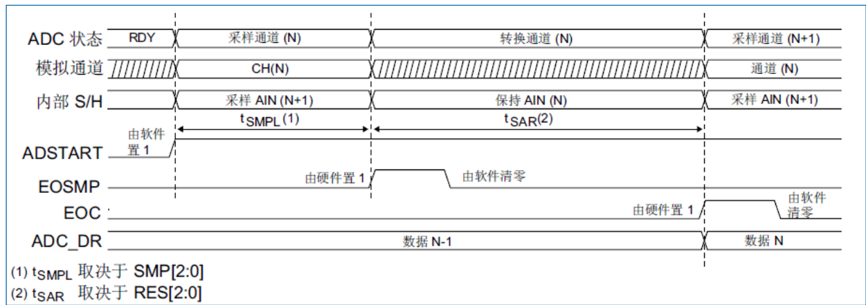
图 11-6 模数转换时间
