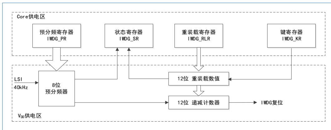
图 20-1 IWDG 框图
