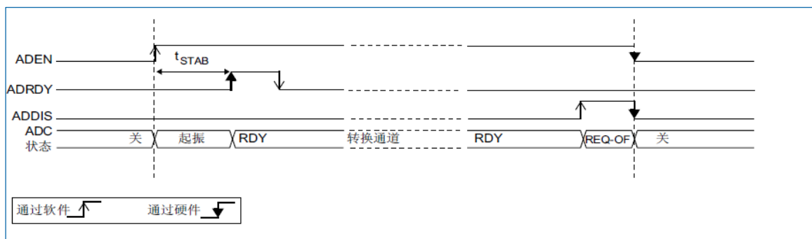
图 11-4 使能/禁用 ADC
