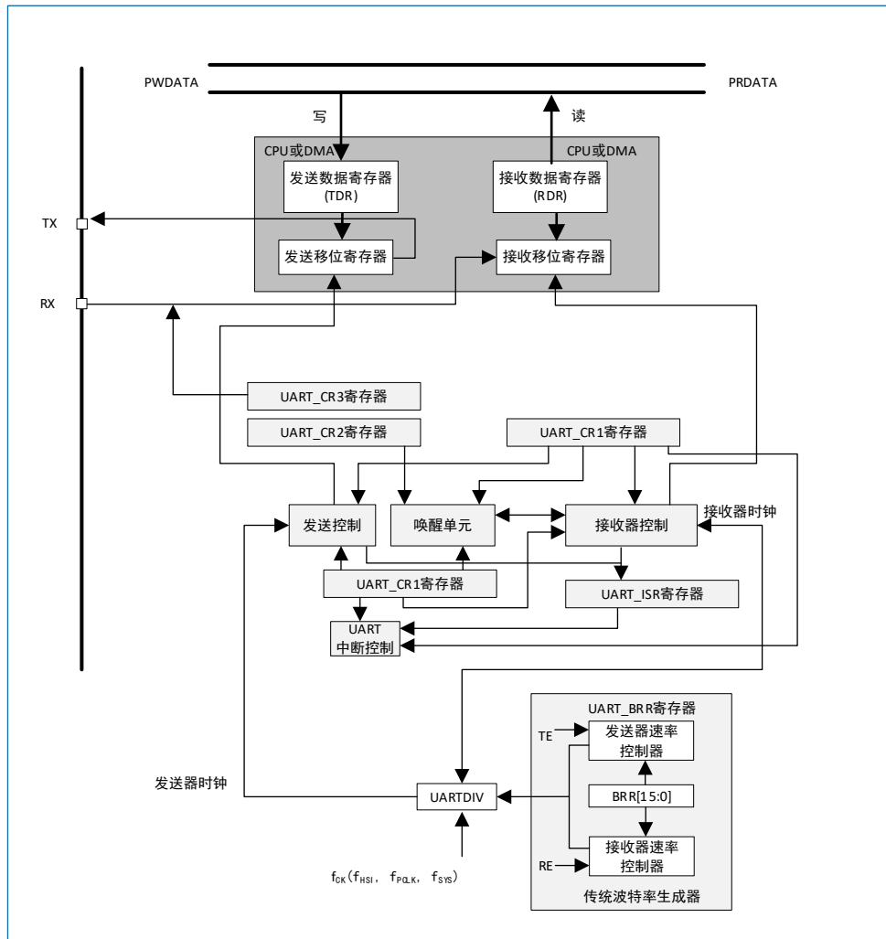
图 23-1 UART 框图
