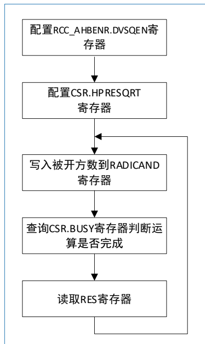
图 13-3 开方运算流程图
