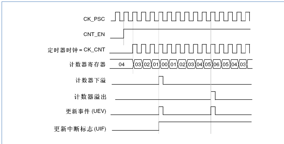
图 14-15 计数器时序图，内部时钟分频因子为 1，TIM1_ARR=0x6（这里使用了中央对齐模式 1）
