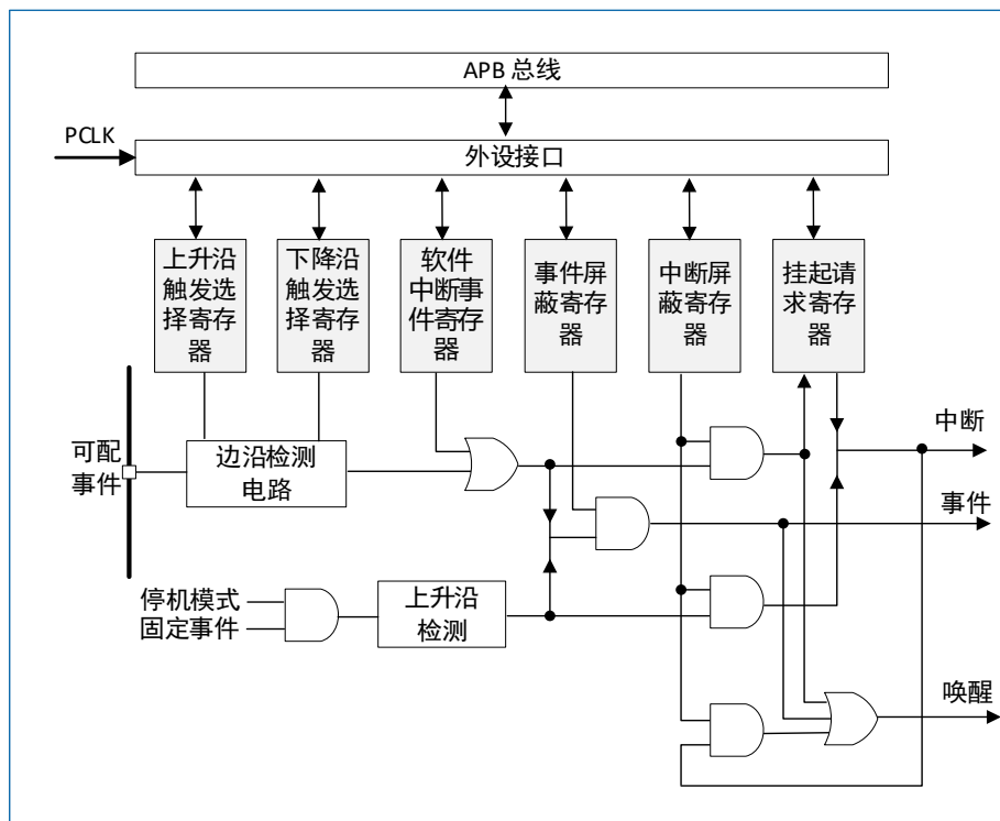
图 10-1 EXTI 框图
