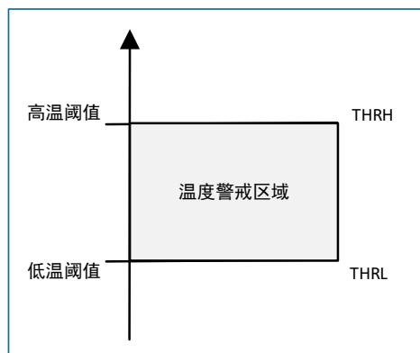
图 12-2 温度传感器的保护区域
