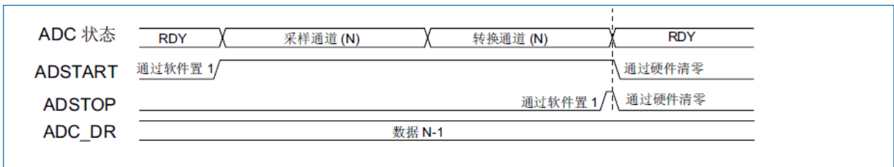
图 11-8 停止正在进行的转换
