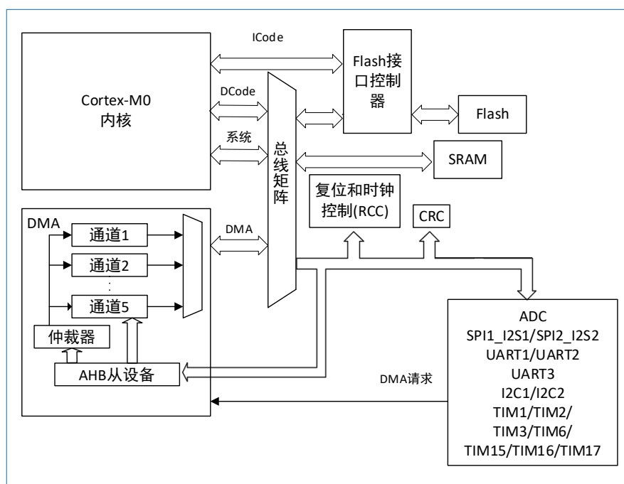
图 9-1 DMA 结构图
