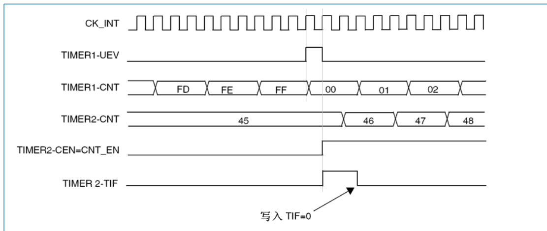
图 15-44 使用定时器 1 的更新触发定时器 2
