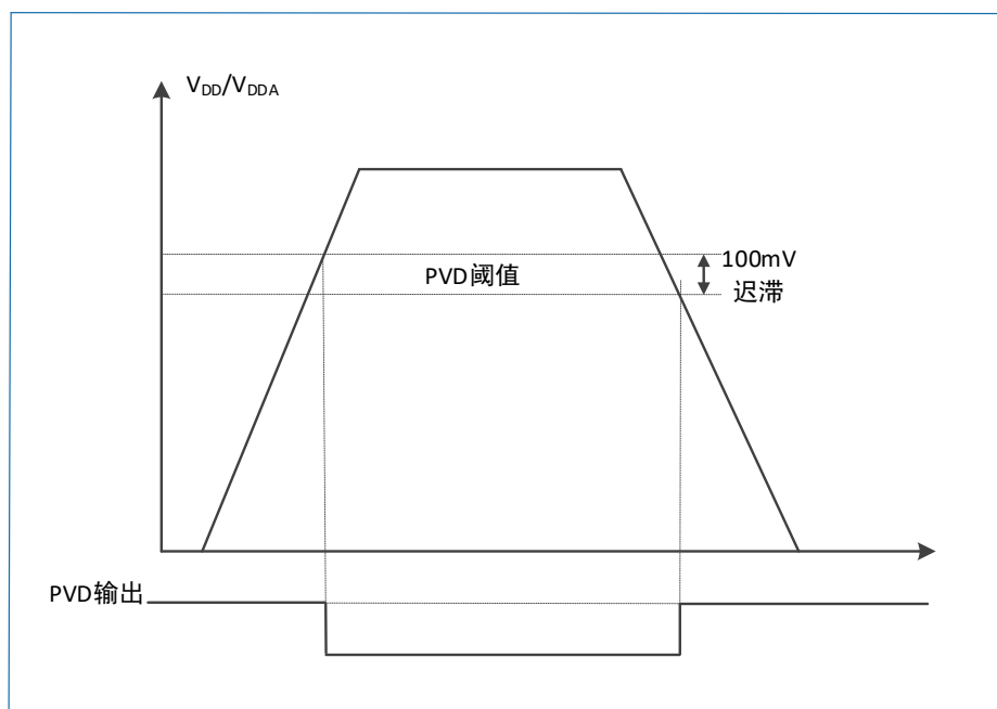
图 5-3 PVD 的门限
