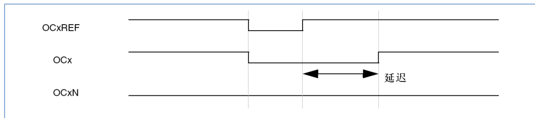
图 14-37 死区波形延迟大于负脉冲
