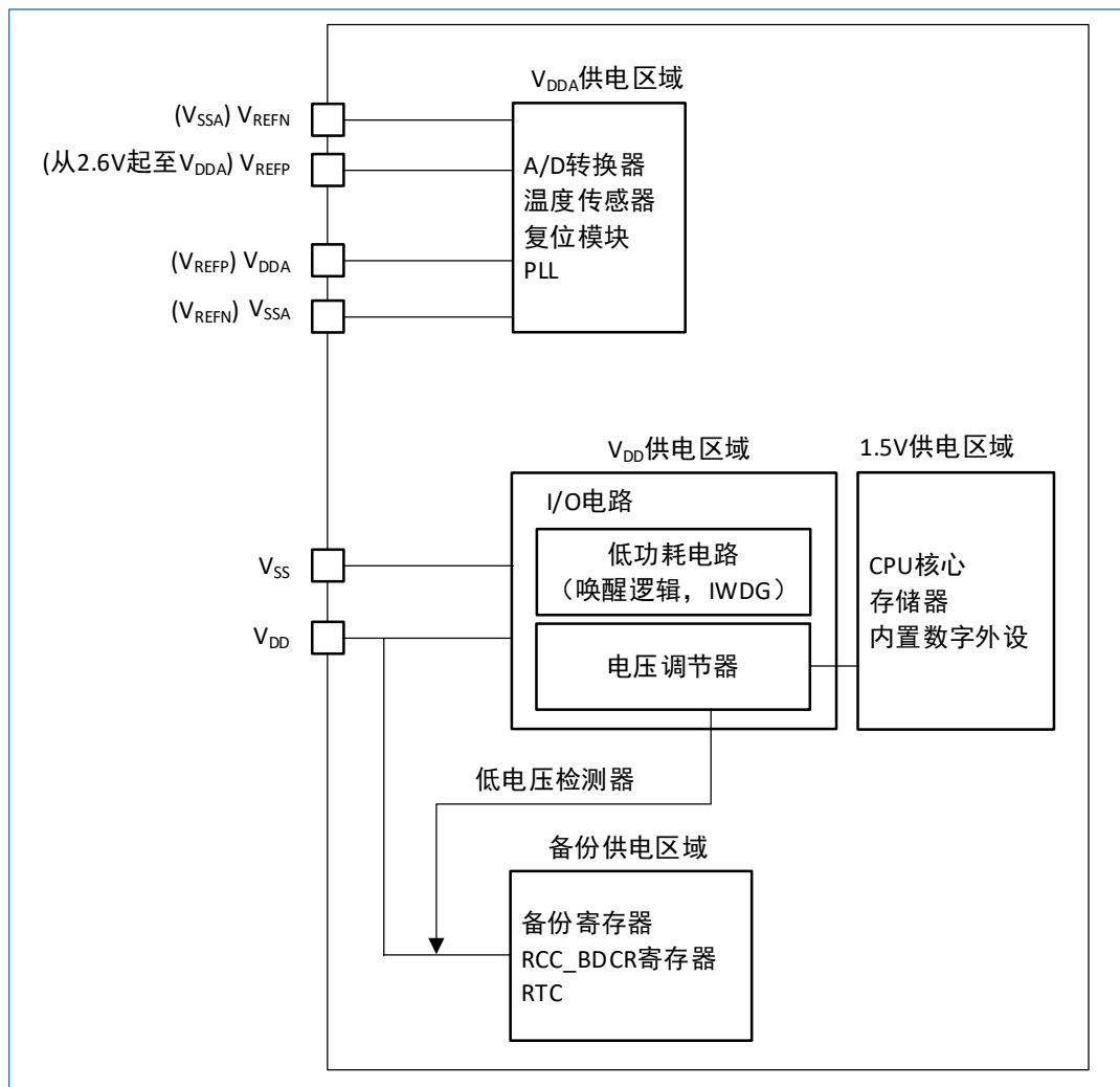
图 5-1 电源框图
