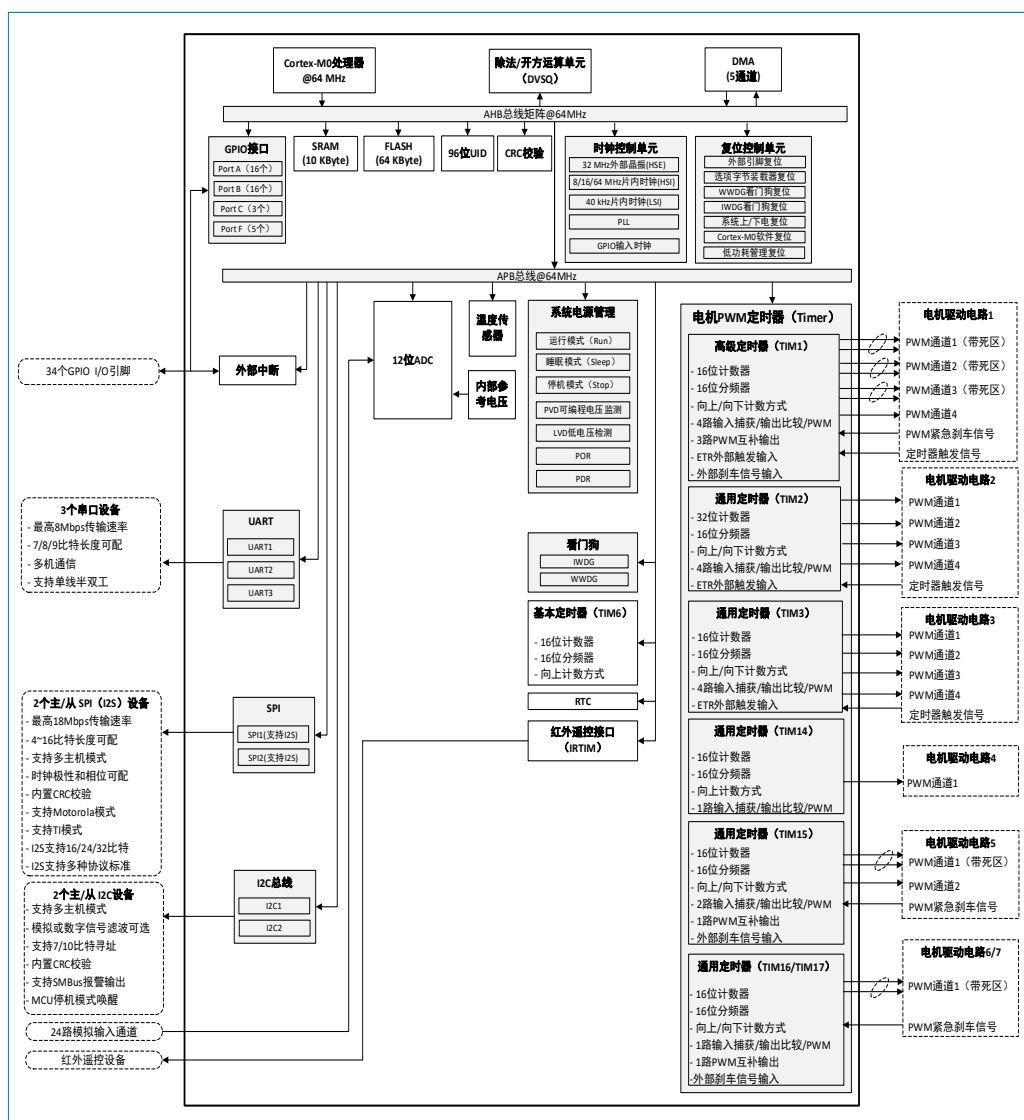
图 2-1 HK32C207S8T7 功能框图
