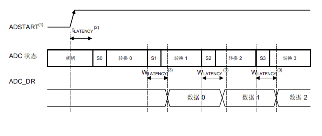
图 11-7 模数转换时序
