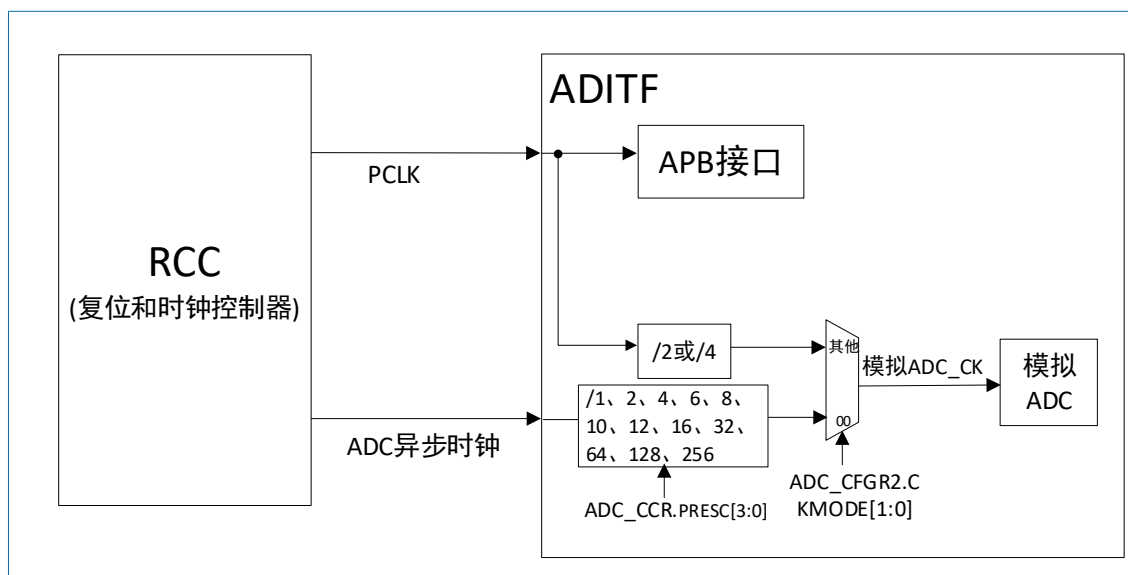
图 11-5 ADC 时钟图
