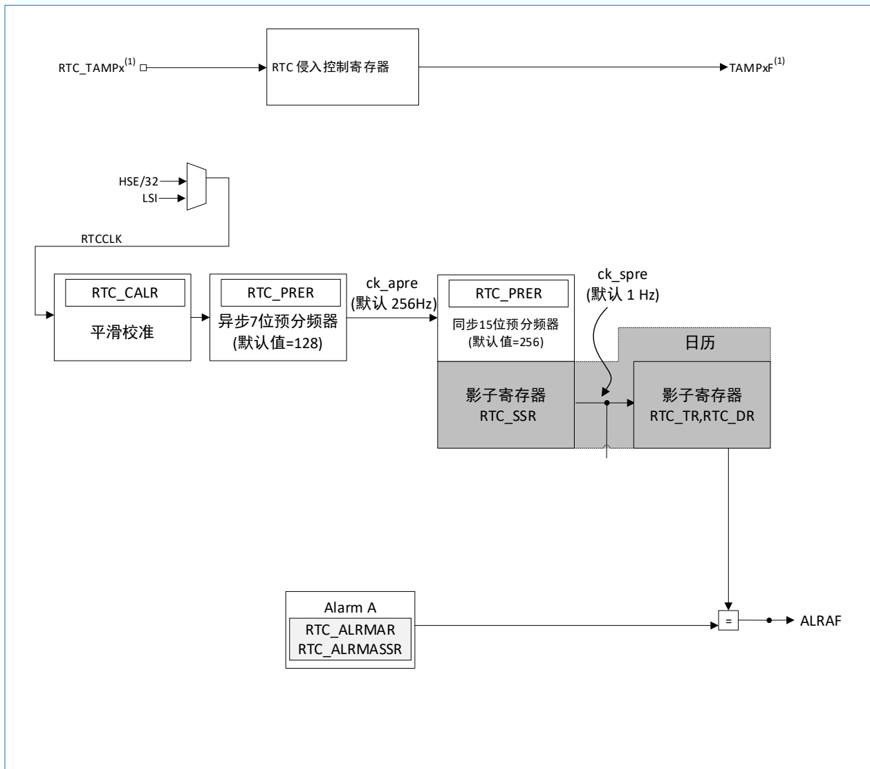
图 25-1 RTC 框图
