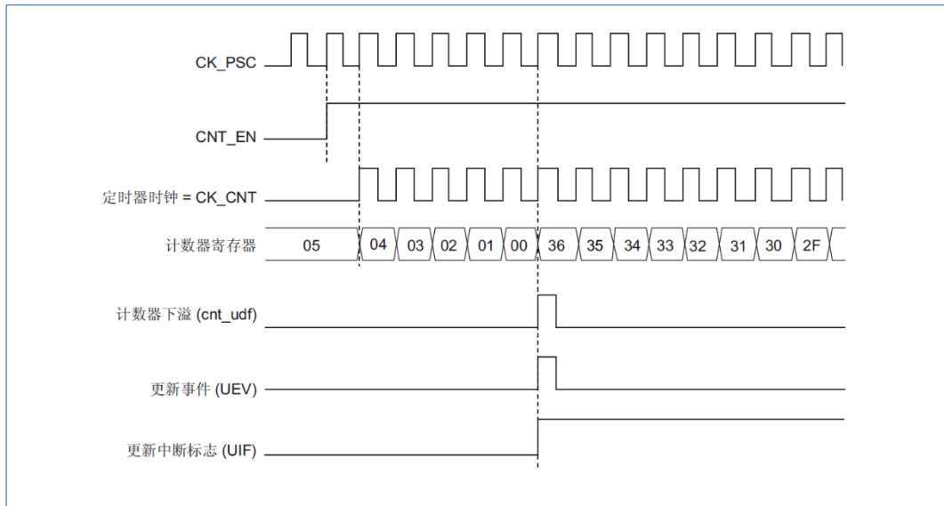
图 15-10 计数器时序图，内部时钟分频因子为 1
