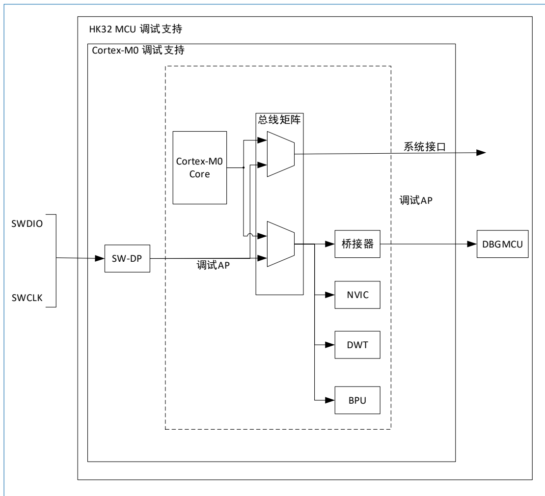
图 27-1 HK32C207 MCU 和 Cortex®-M0 级调试支持框图
