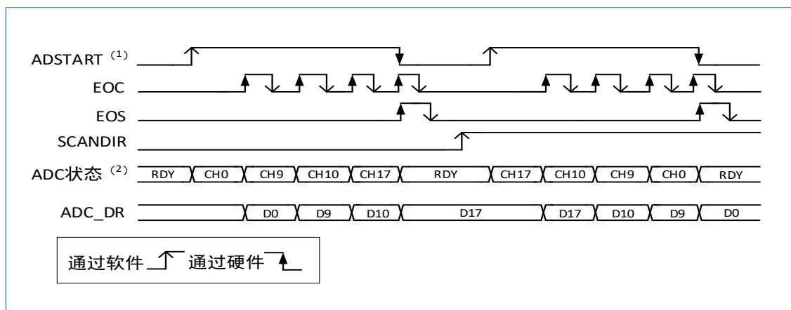
图 11-9 单次序列转换, 软件触发
