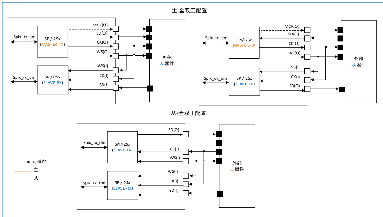
图 24-17 全双工通信
