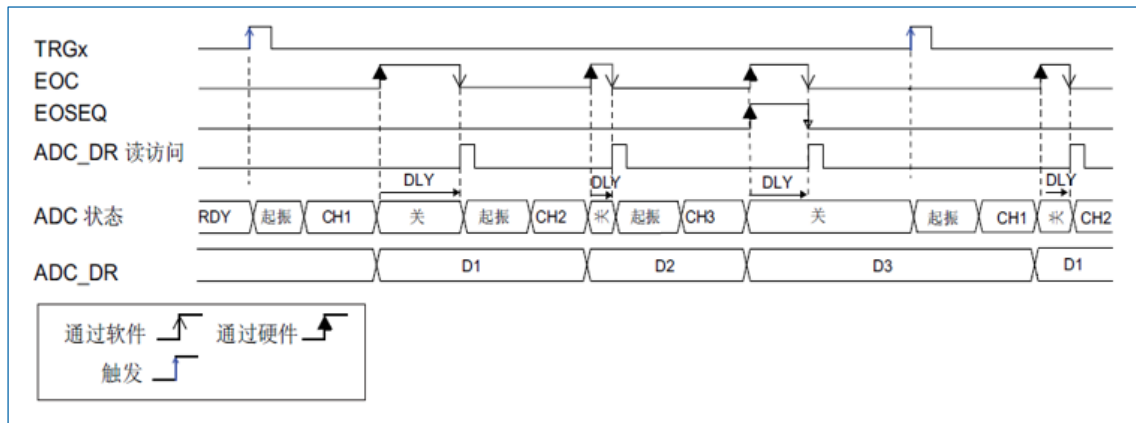
图 11-17 WAIT=1、AUTOFF=1 时的行为
