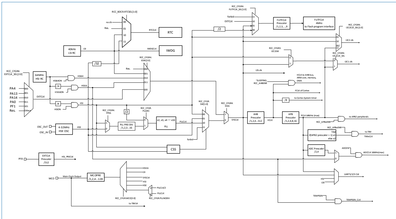
图 6-2 时钟树
