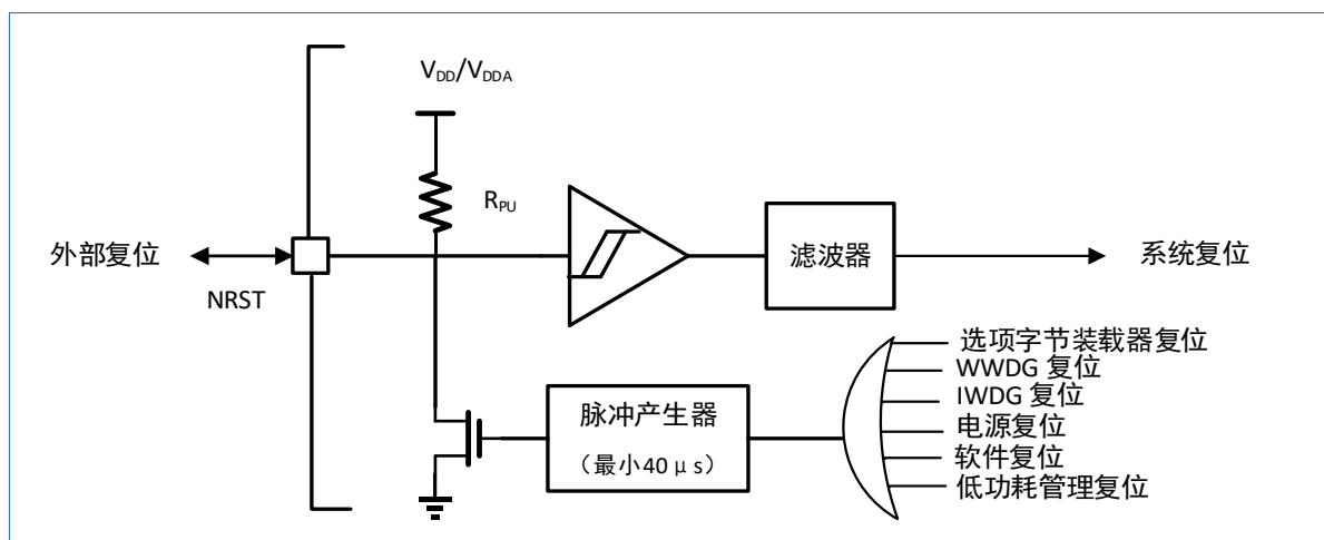
图 6-1 复位电路
