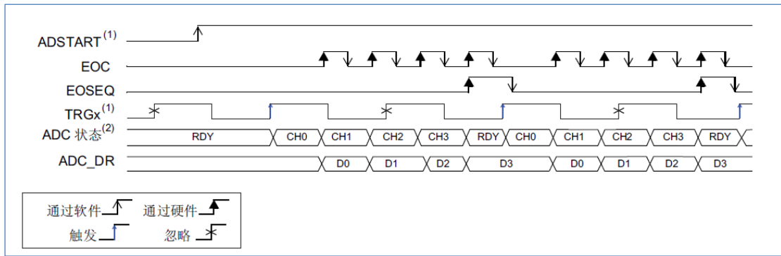
图 11-11 单序列转换，硬件触发
