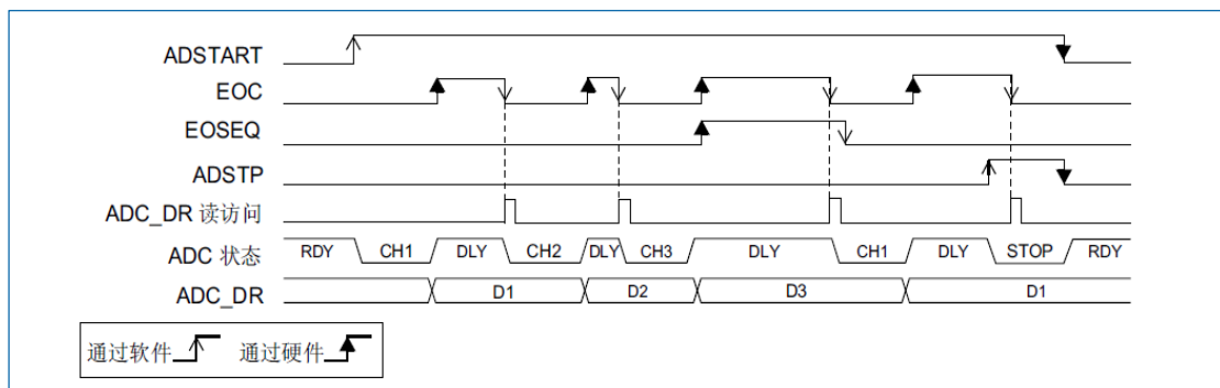
图 11-15 等待模式转换（连续模式，软件触发）
