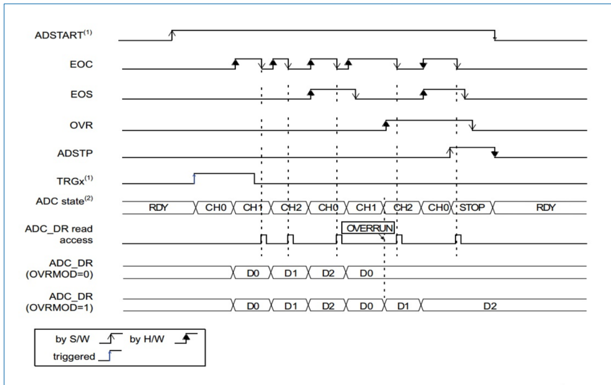
图 11-14 溢出示例 (OVR)
