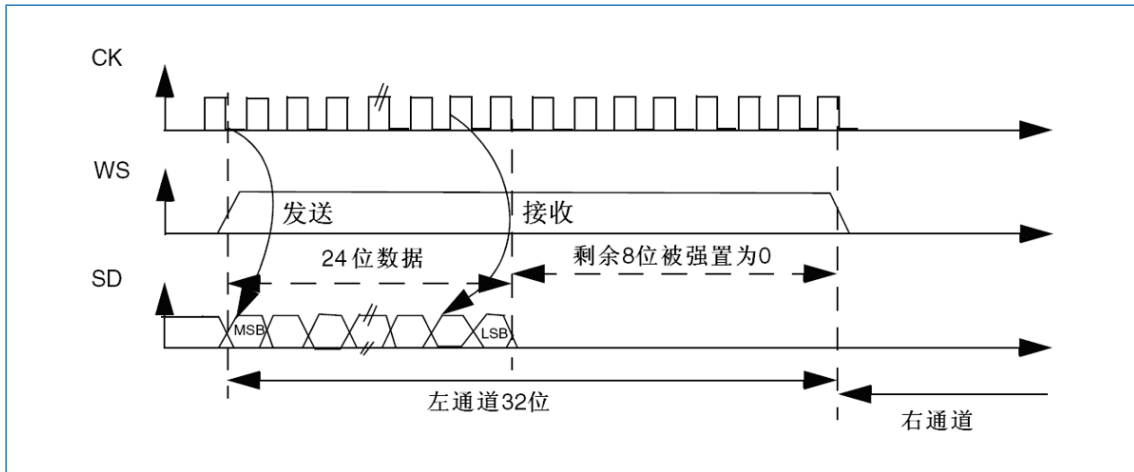
图 24-26 MSB 对齐 16 位数据扩展到 32 位数据包帧, CPOL=0
