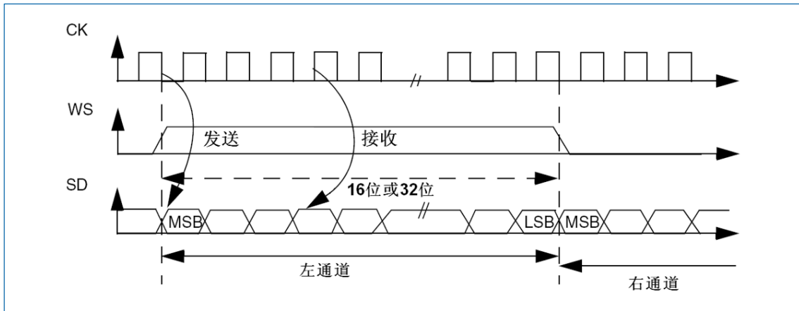
图 24-27 LSB 对齐的 16 位或 32 位全精度, CPOL=0
