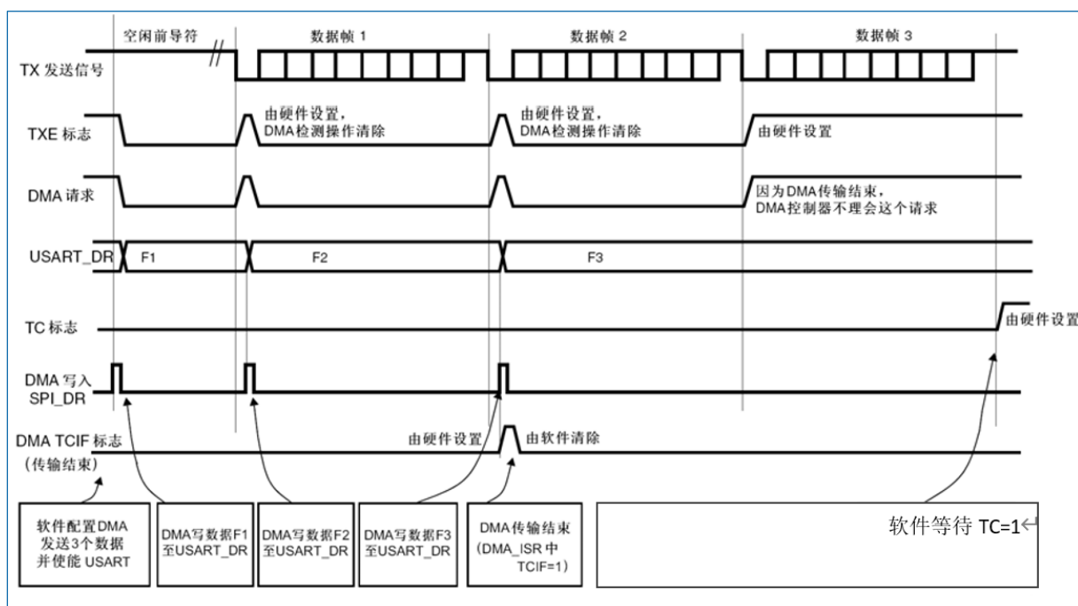
图 21-19 利用 DMA 发送
