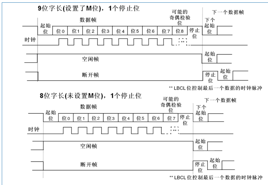
图 21-2 字长设置
