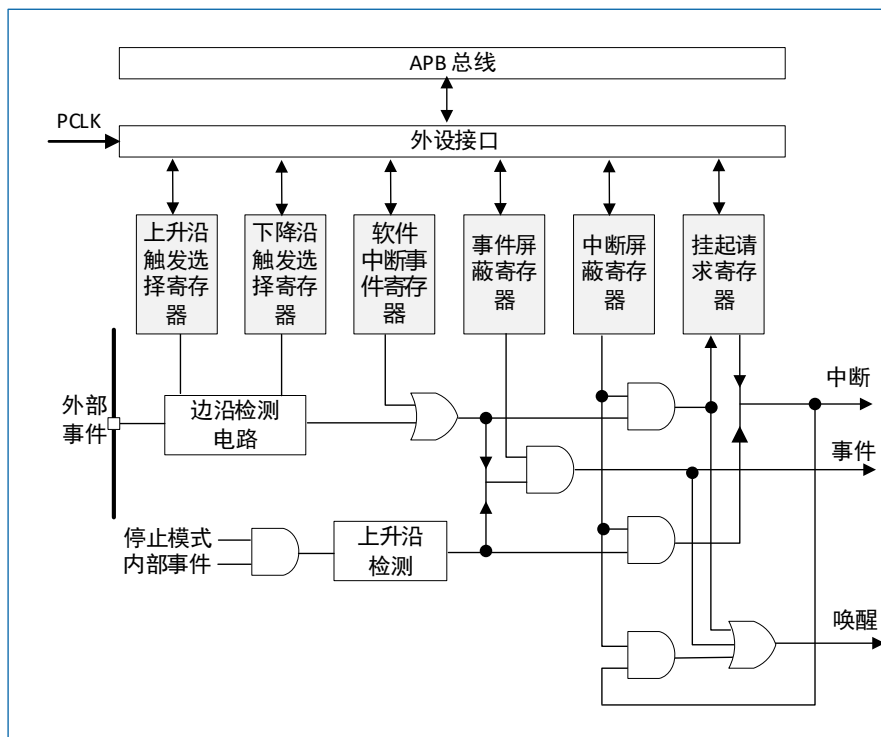
图 8-1 EXTI 框图
