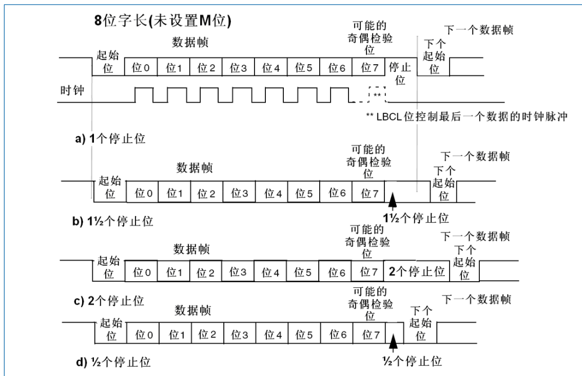
图 21-3 配置停止位
