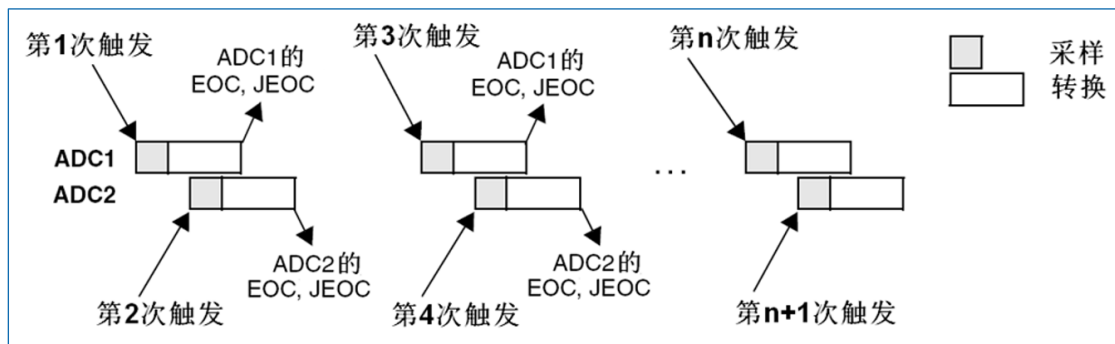
图 11-13 交替触发：每个 ADC1 的注入通道组
