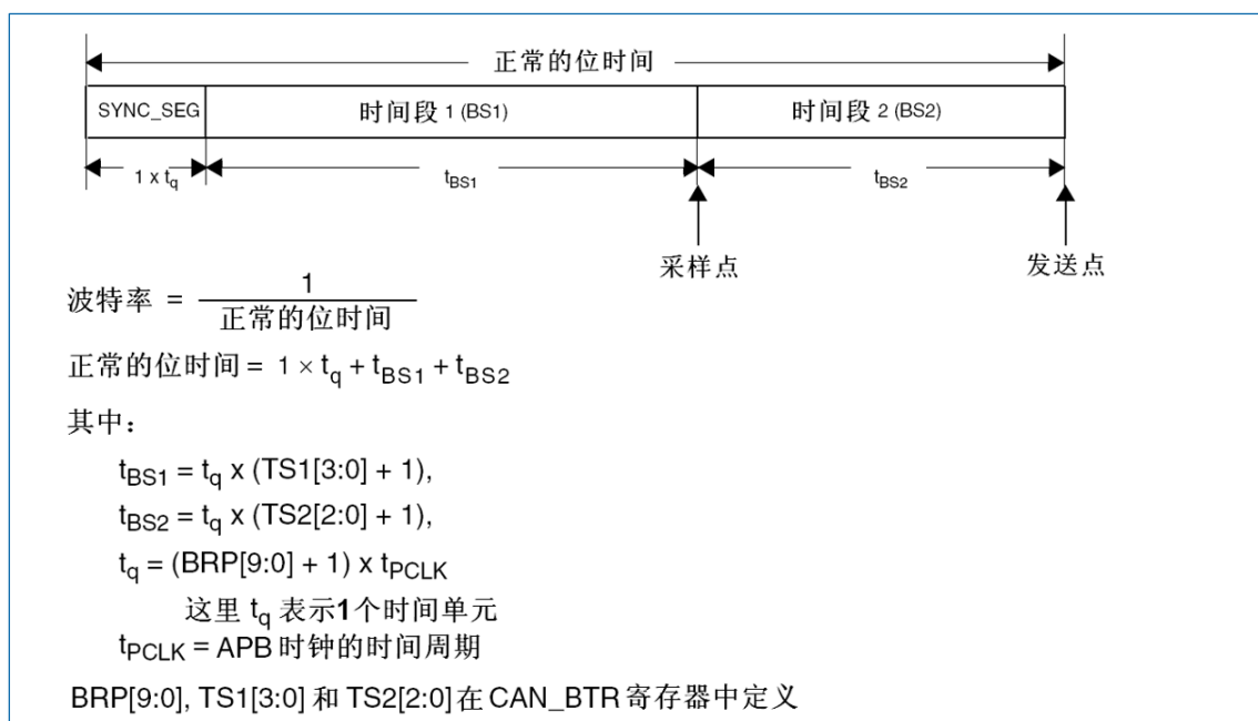
图 18-13 位时序
