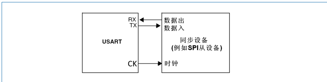
图 21-11 USART 同步传输的例子
