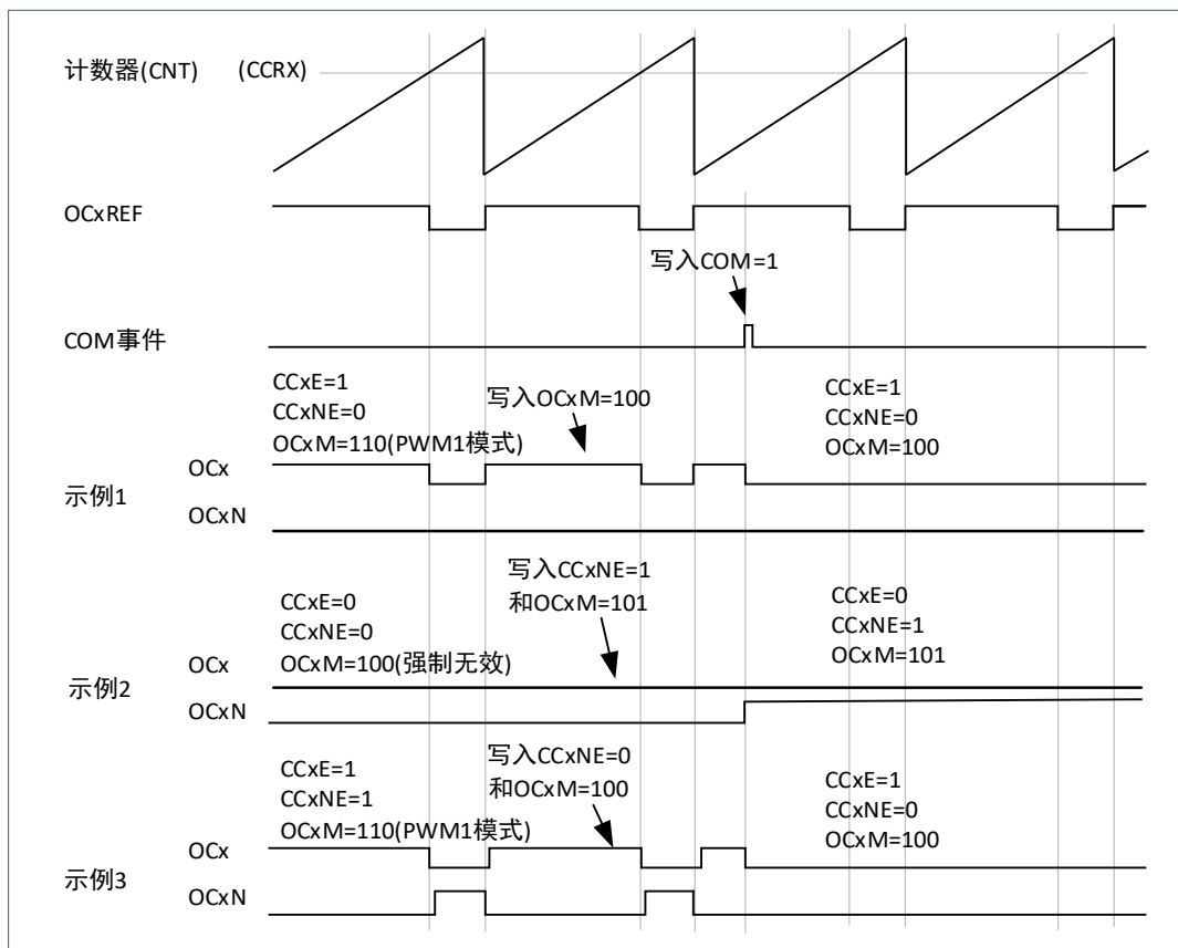
图 12-40 产生六步 PWM，使用 COM 的例子 (OSSR=1)
