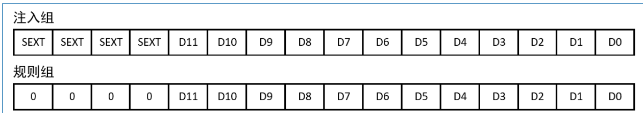
图 11-6 数据右对齐
