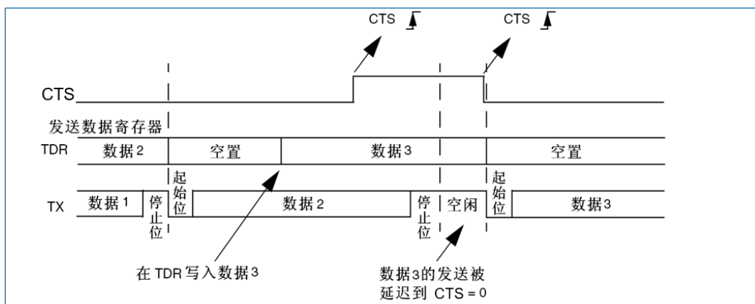
图 21-23 CTS 流控制
