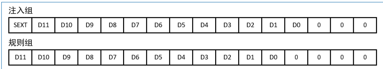
图 11-7 数据左对齐
