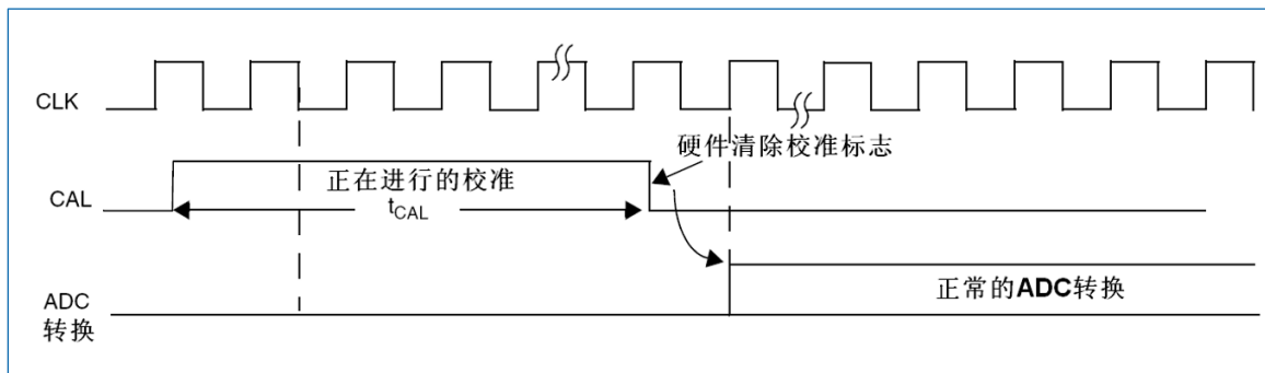
图 11-5 校准时序图
