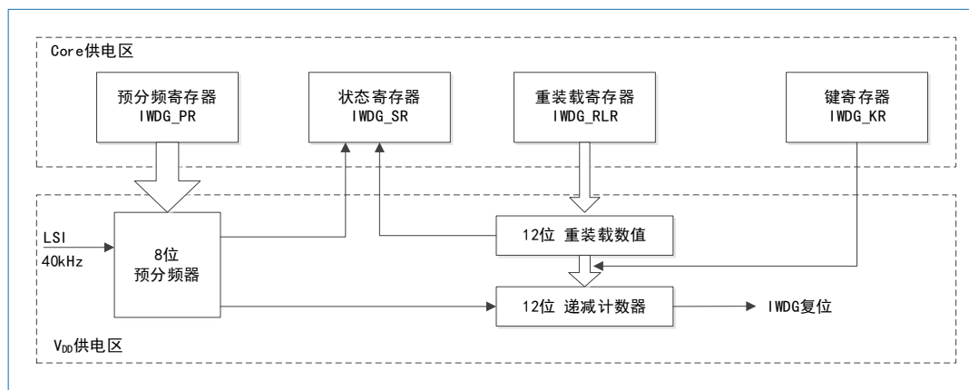
图 15-1 IWDG 框图
