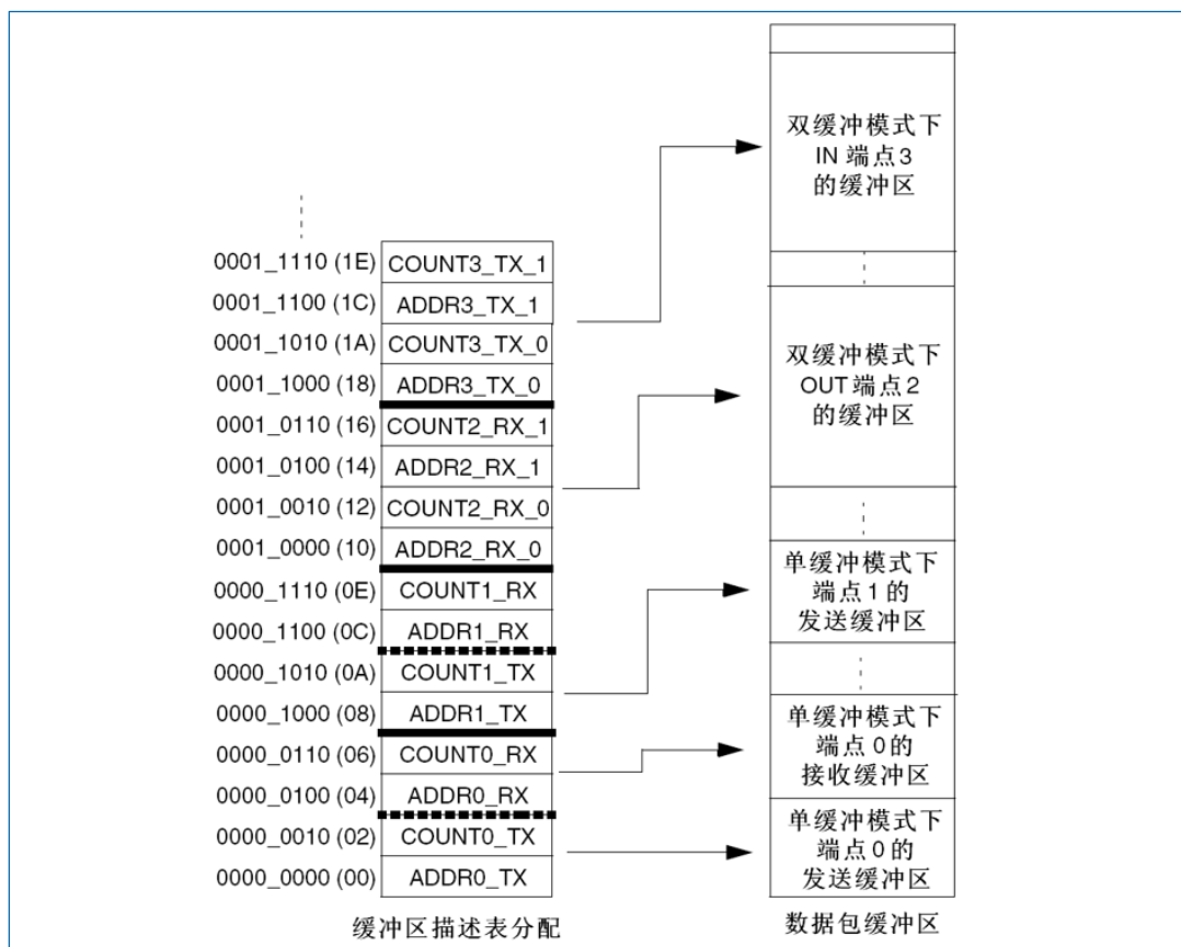
图 17-2 分组缓冲区对应的缓冲区描述表项定位
