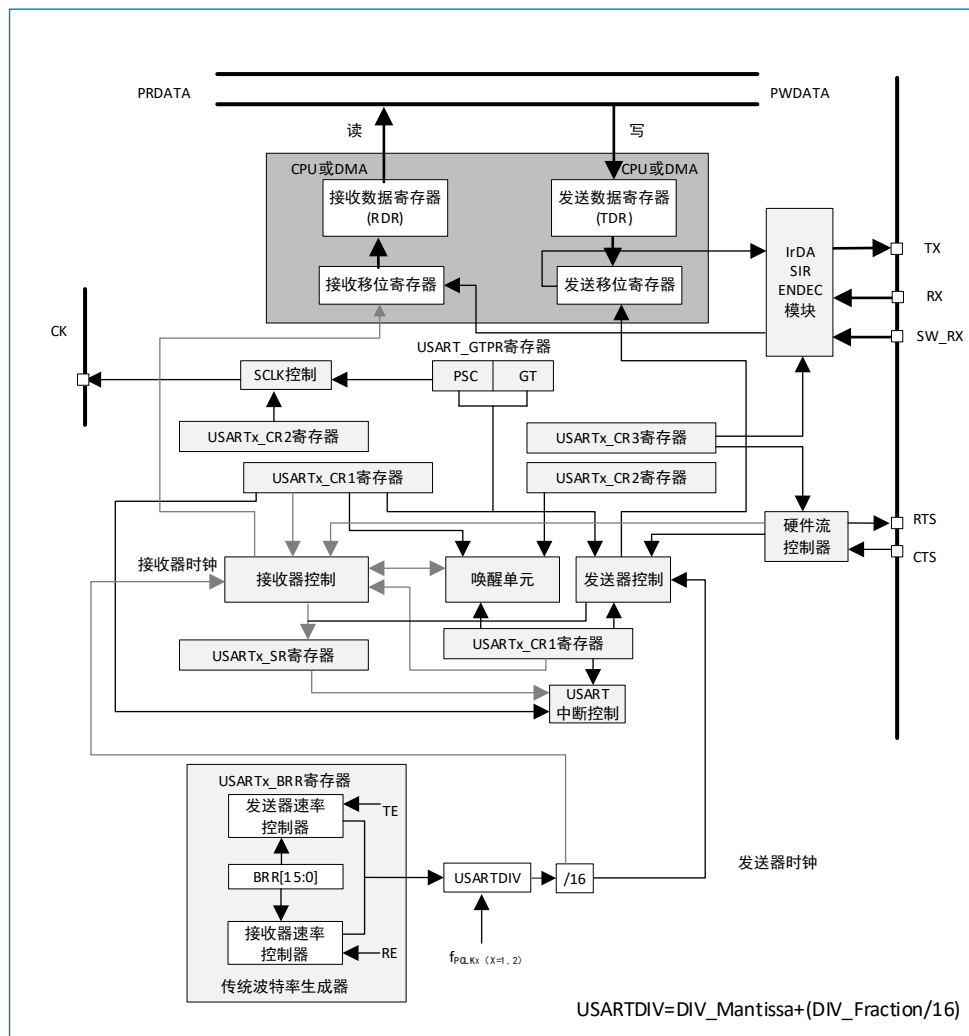
图 21-1 USART 框图
