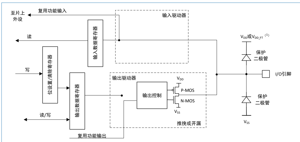
图 9-4 输出配置
