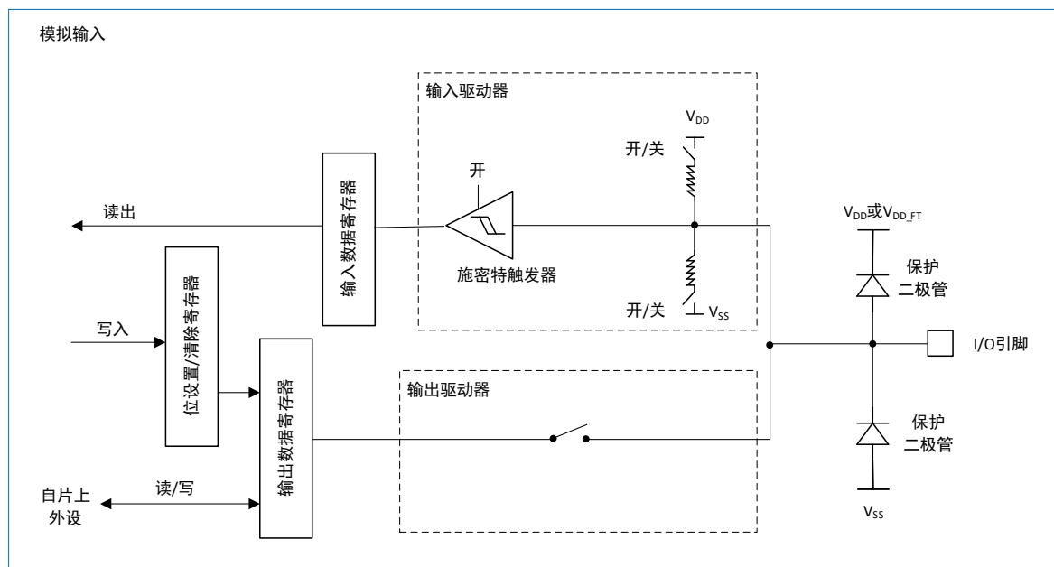
图 9-3 输入浮空/上拉/下拉配置
