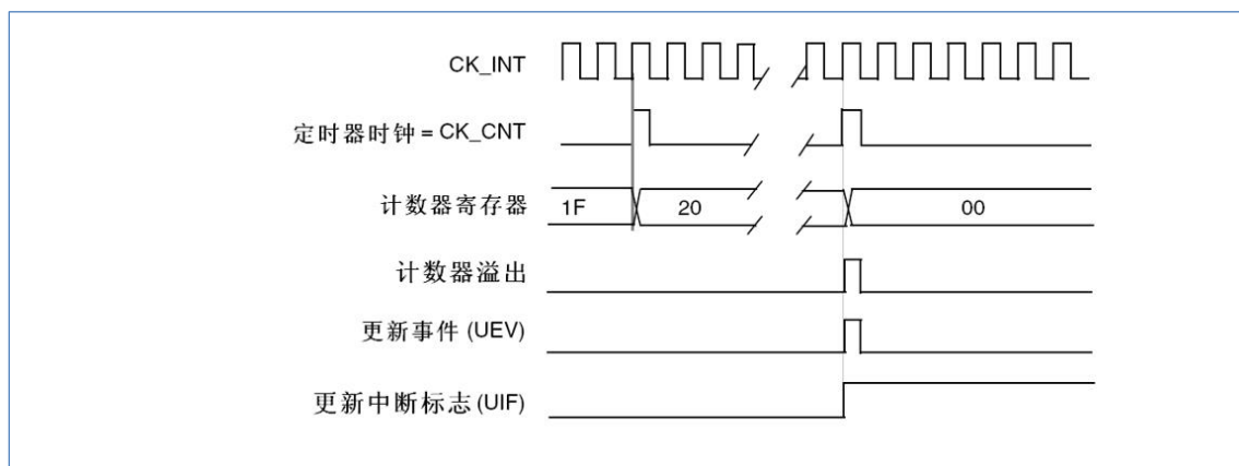
图 13-7 计数器时序图，内部时钟分频因子为 N
