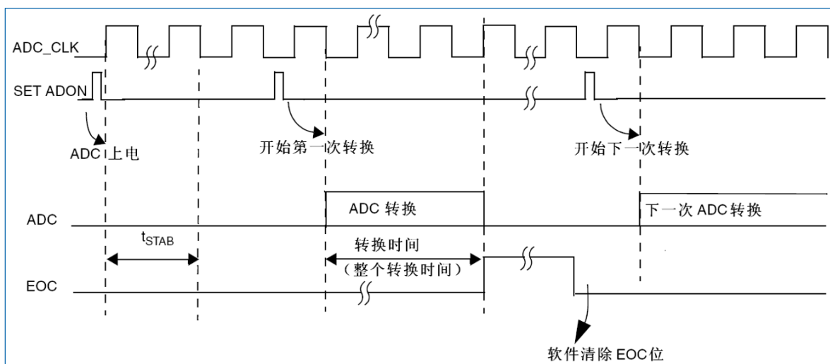
图 11-2 时序图
