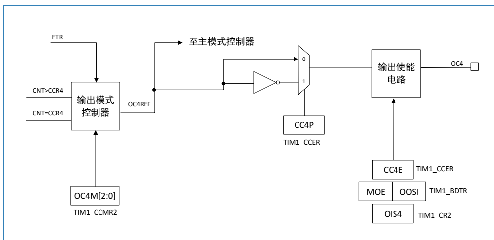
图 12-30 捕获/比较通道的输出部分（通道 4）
