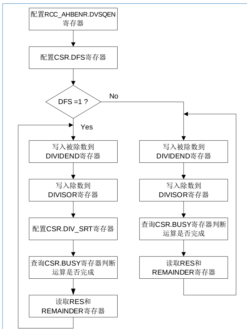
图 22-2 除法运算流程示意图
