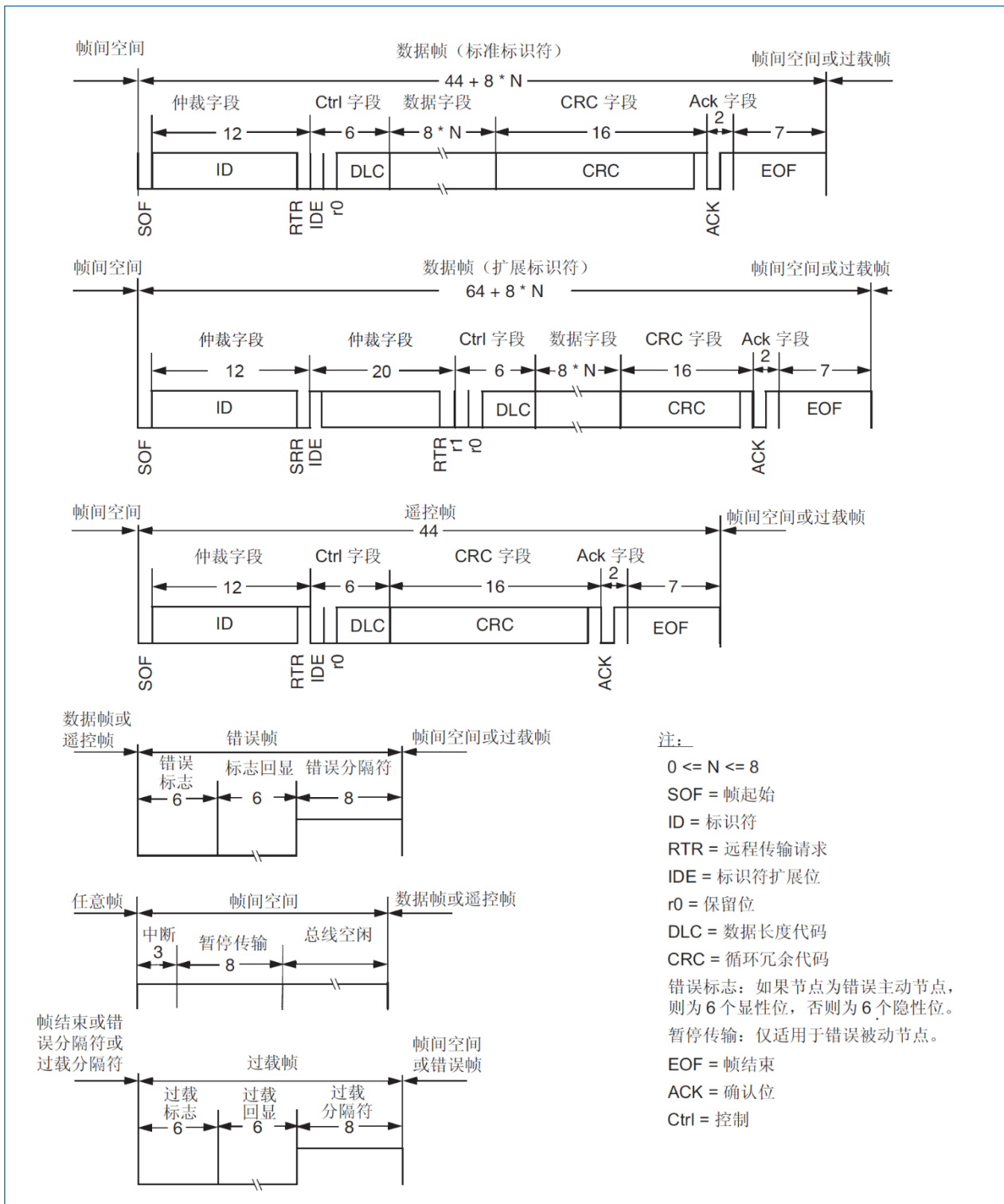
图 18-14 各种 CAN 帧
