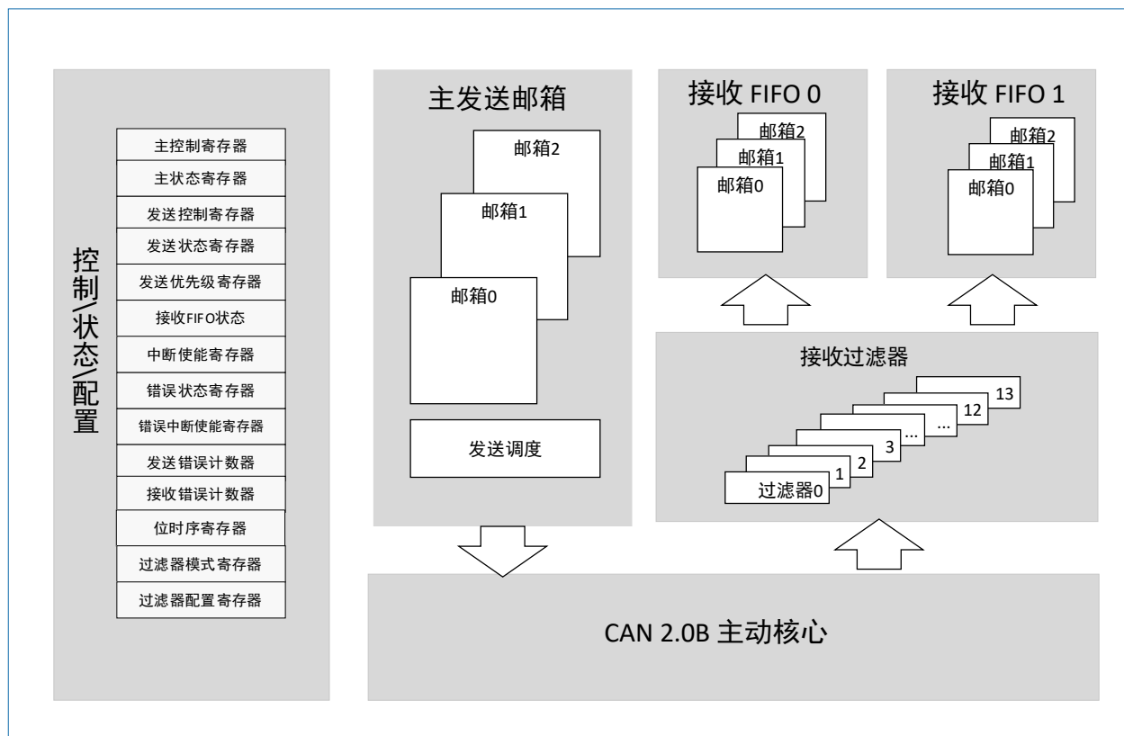
图 18-2 CAN 框图
