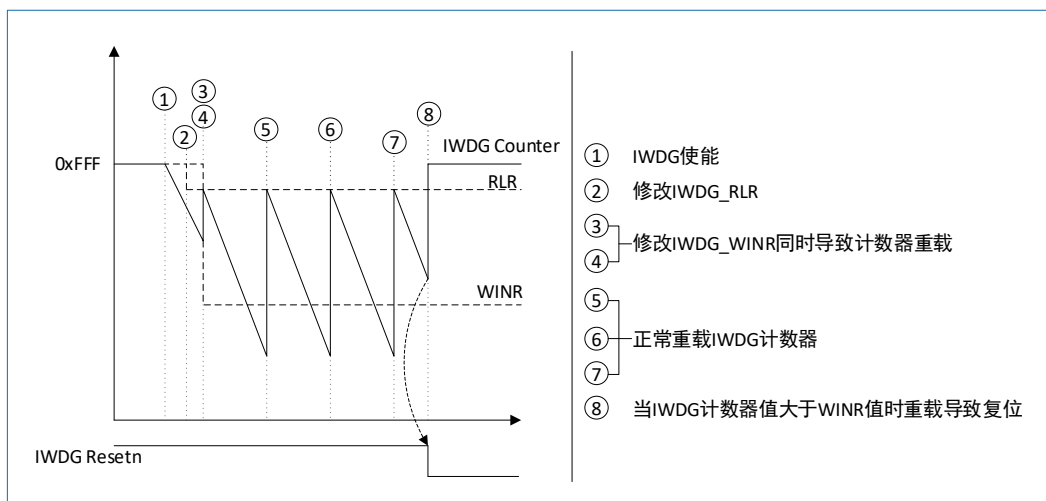
图 15-2 IWDG 使能窗口选项时的工作说明
