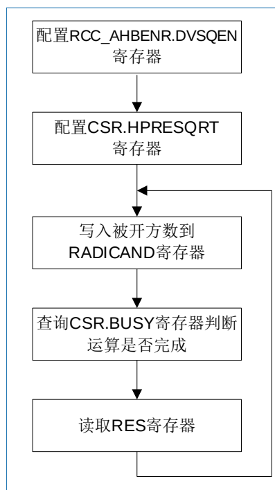
图 22-3 开方运算流程图
