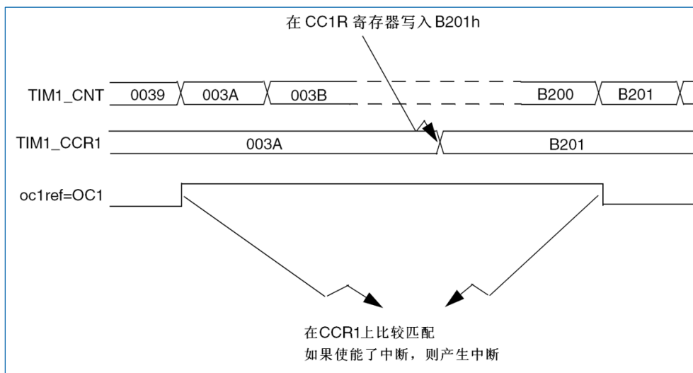
图 12-32 输出比较模式，翻转 OC1
