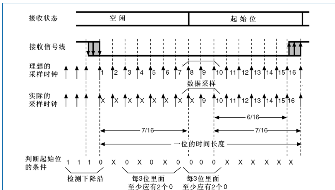
图 21-5 起始位检测
