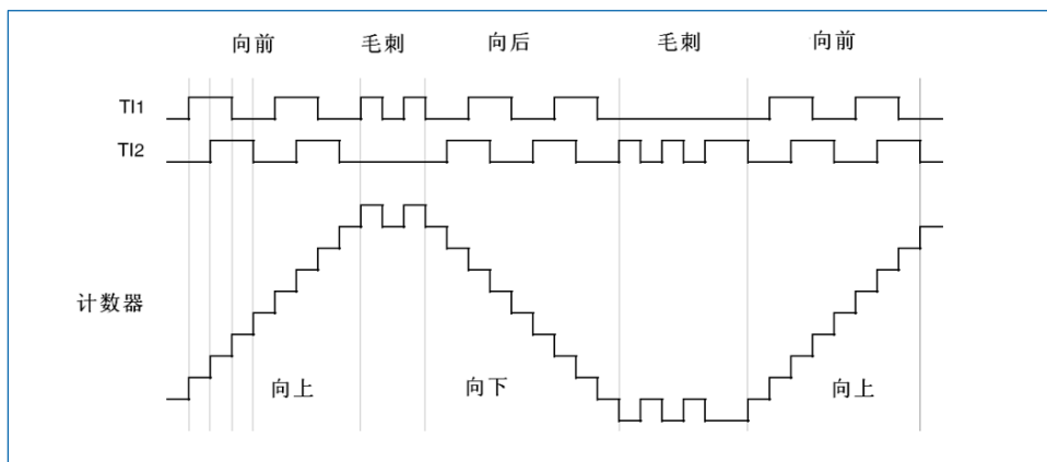
图 12-42 编码器模式下的计数器操作实例
