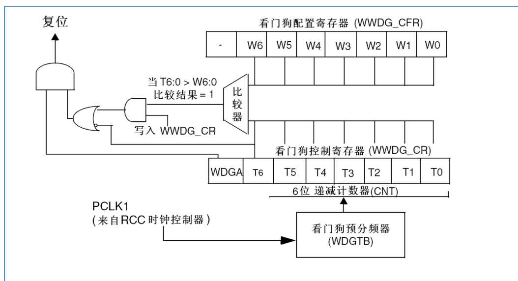
图 16-1 看门狗框图
