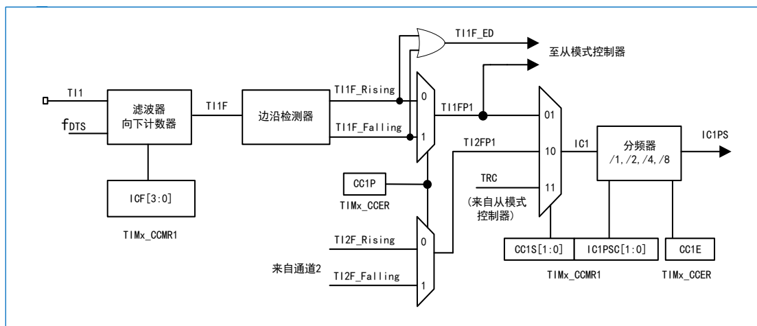
图 12-27 捕获/比较通道（如：通道 1 输入部分）
