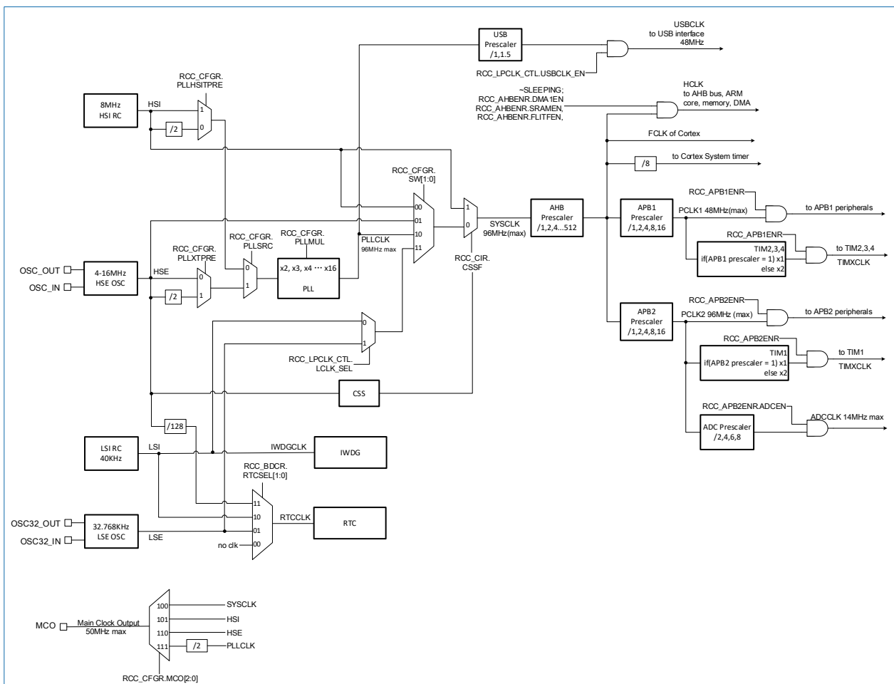
图 7-2 时钟树
