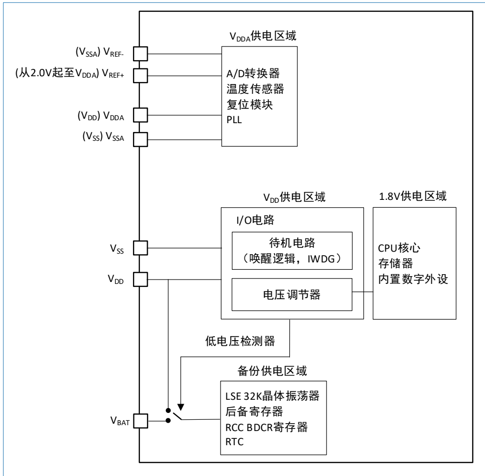
图 5-1 电源框图
