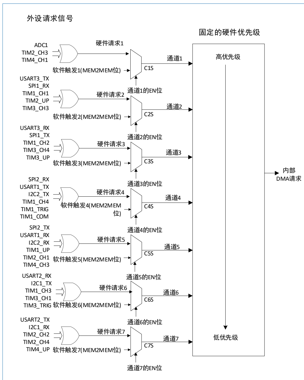
图 10-2 DMA 请求映射
