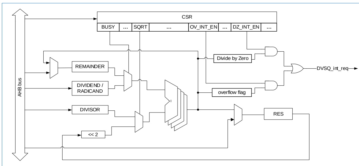
图 22-1 DVSQ 结构图
