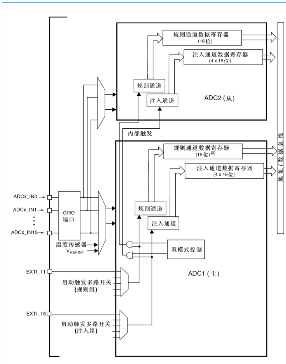
图 11-8 双 ADC 框图
