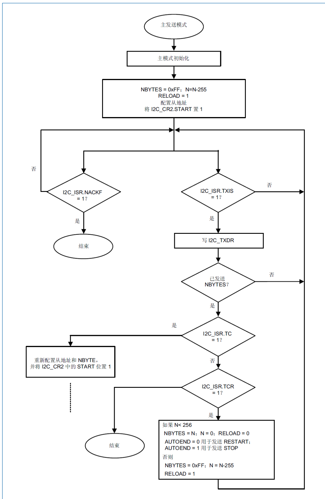
图 18-19 I2C 主发送器的传输序列流程图 (N&gt;255 字节)
