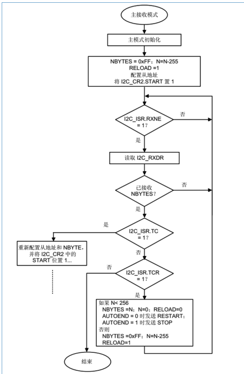
图 18-22 I2C 主接收器的传输序列流程图 (N&gt;255 字节)
