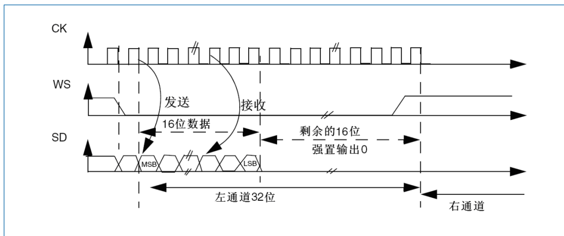
图 20-21 I2S Philips 标准 (16 位扩展为 32 位数据包帧, CPOL=0)
