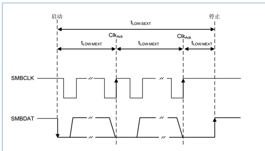
图 18-24 t_{\text{LOW: SEXT}} 和 t_{\text{LOW: MEXT}} 的超时时间间隔
