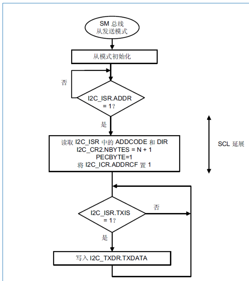
图 18-25 SMBus 从发送器的传输序列流程图 (N 字节+PEC)
