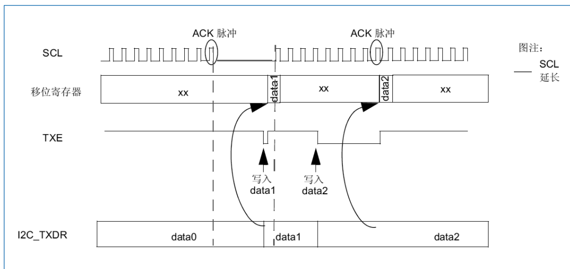
图 18-6 数据发送
