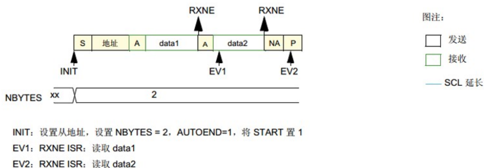
示例：I2C 主器件接收 2 个字节，自动结束模式 (STOP)
