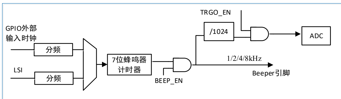
图 21-1 蜂鸣器框图
