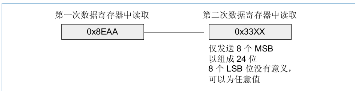
图 20-20 接收 0x8EAA33
