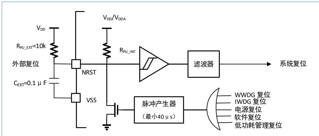
图 6-1 复位电路
