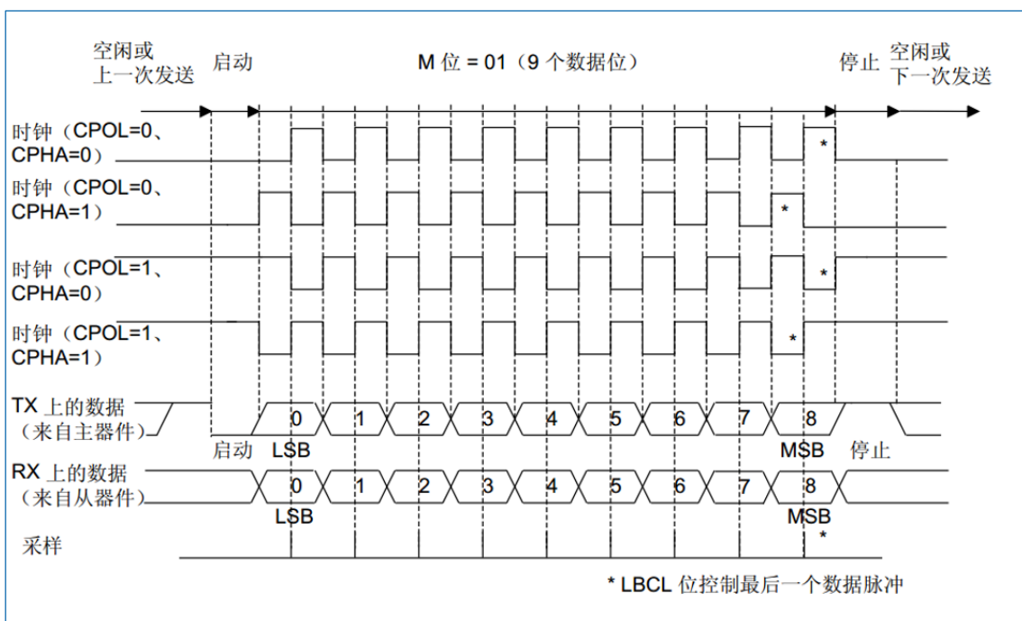
图 19-14 USART 数据时钟时序图 (M 位=01)
