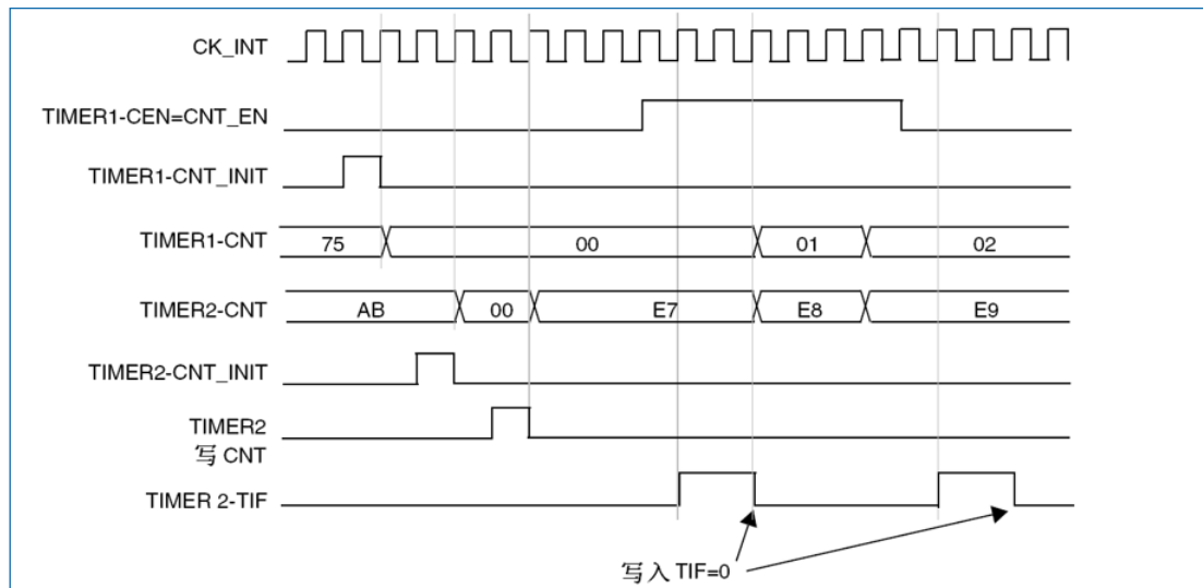
图 13-43 通过使用 TIMx 可以控制 TIMy
