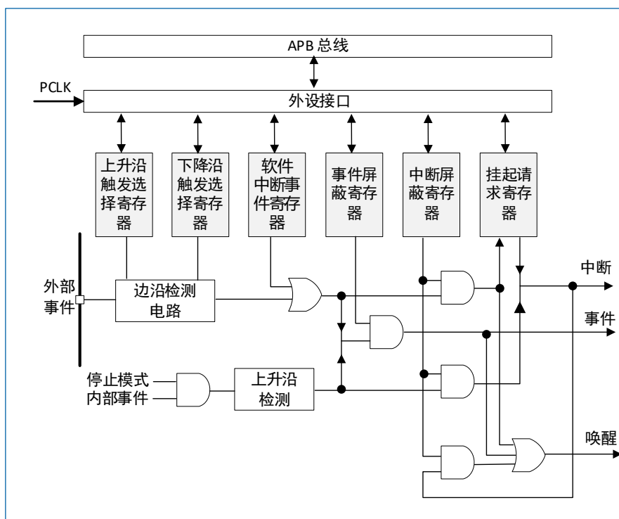
图 10-1 EXTI 框图
