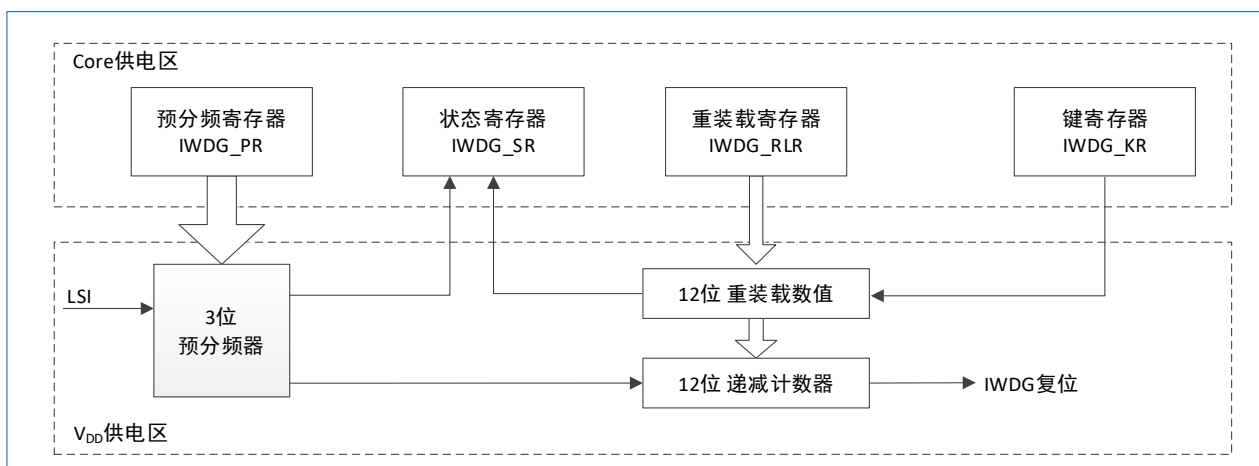
图 16-1 IWDG 框图
