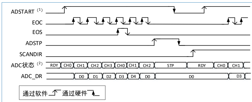
图 11-9 连续序列转换，软件触发
