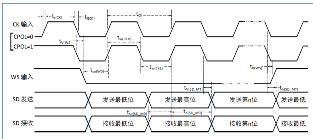
图 20-37 I2S 总线主模式时序图（飞利浦协议）
