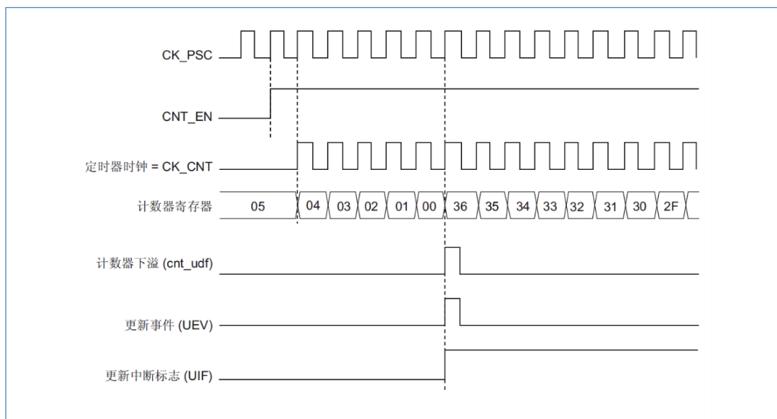
图 13-10 计数器时序图，内部时钟分频因子为 1
