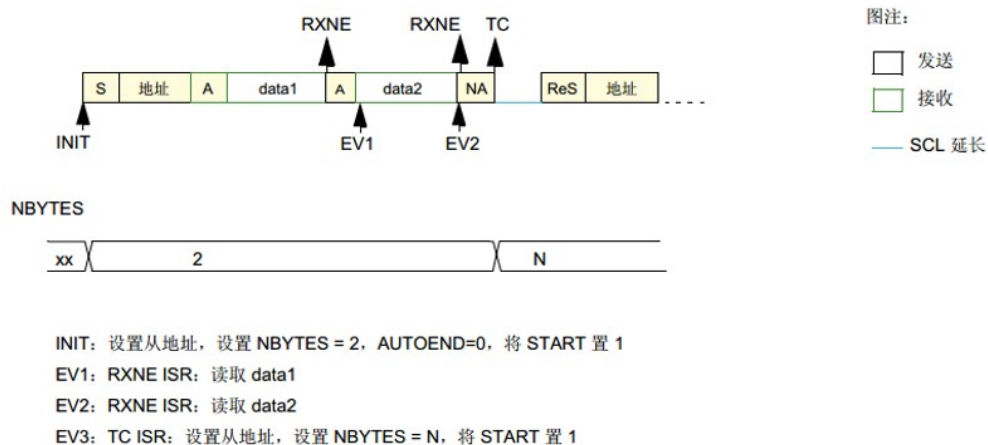
示例：I2C 主器件接收 2 个字节，软件结束模式 (RESTART)
