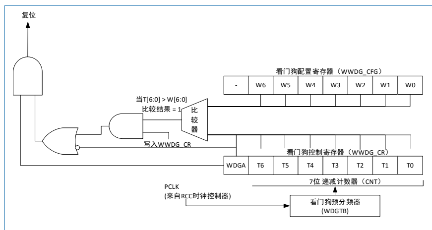
图 17-1 WWDG 框图
