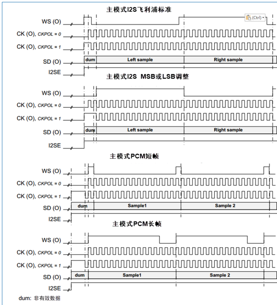
图 20-34 主模式下启动序列
