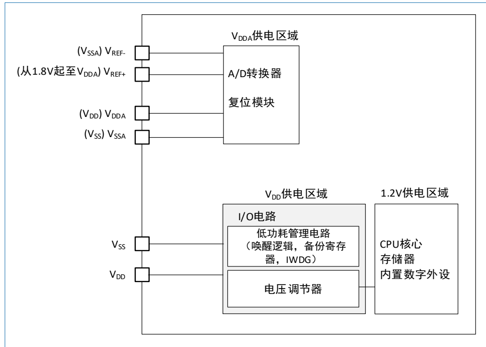
图 5-1 电源框图
