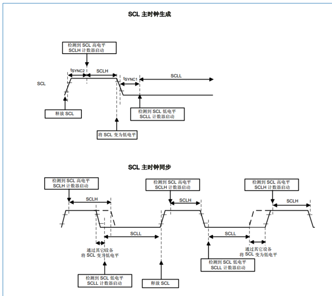
图 18-14 主时钟生成
