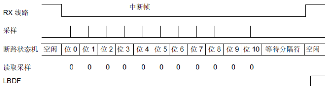
图 19-10 LIN 模式下的断路检测 (11 位断路长度——LBDF 位置 1)
