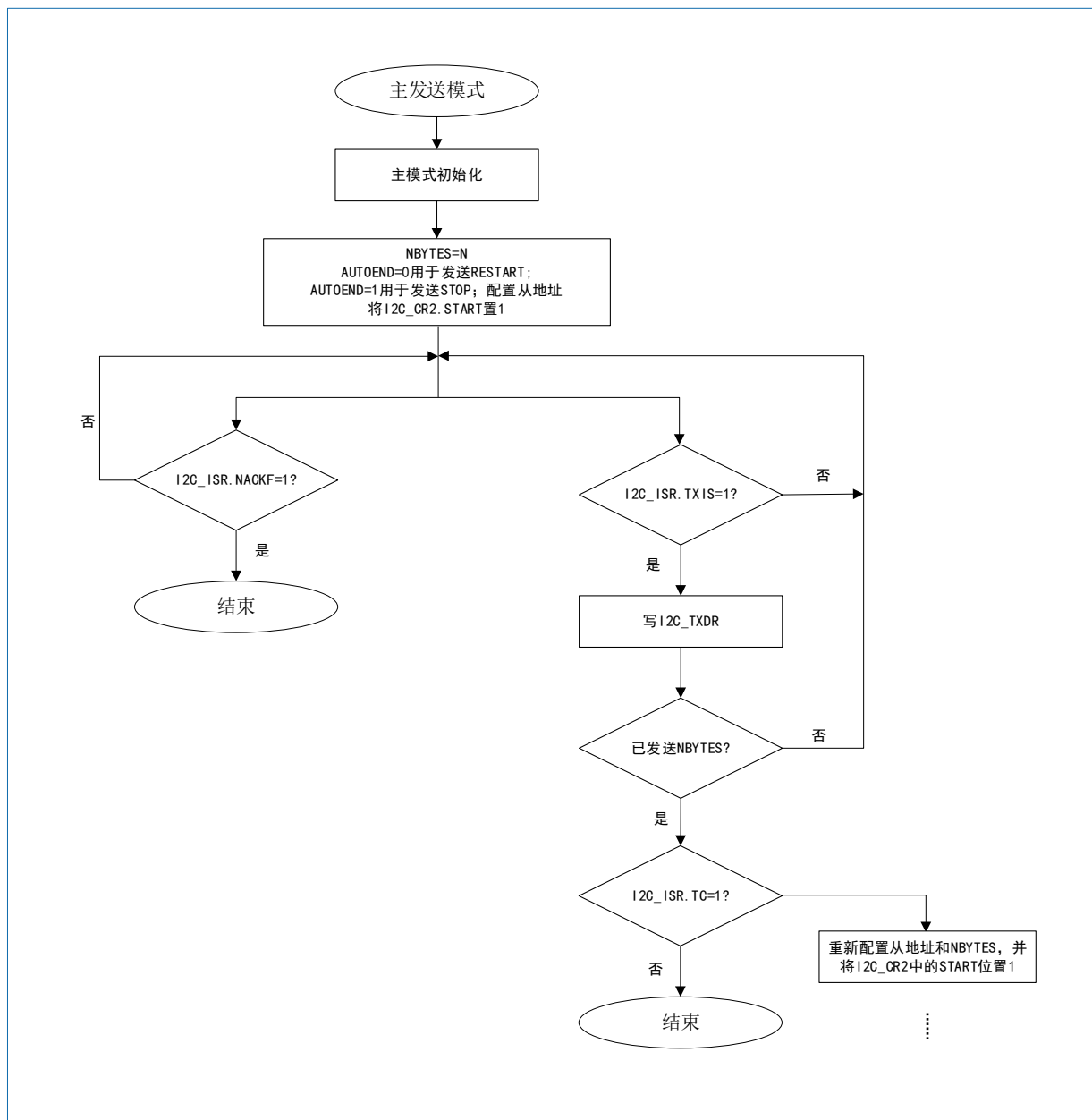
图 18-18 I2C 主发送器的传输序列流程图 (N ≤ 255 字节)
