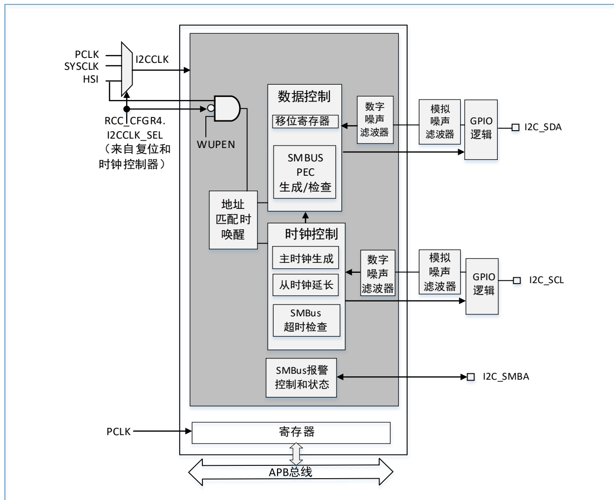
图 18-1 I2C 框图
