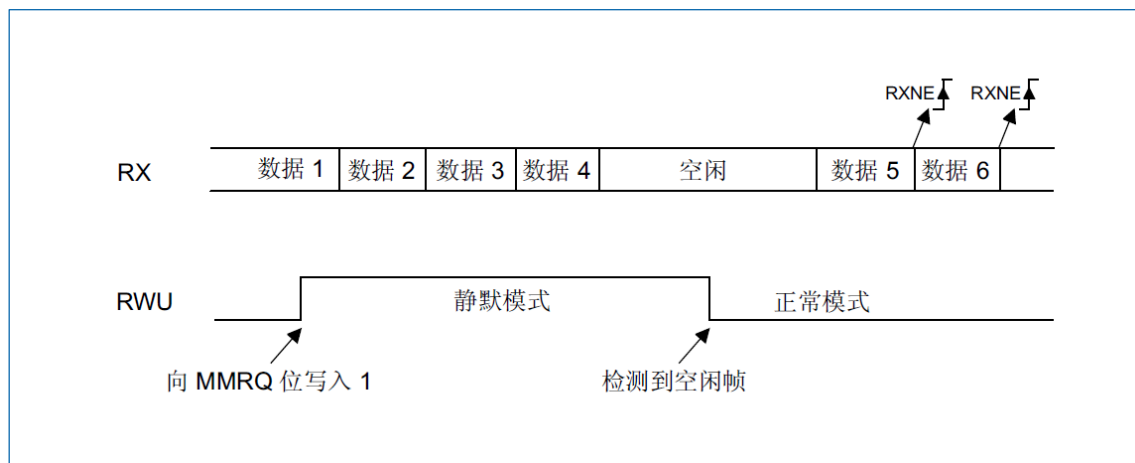
图 19-8 使用空闲线路检测时的静默模式
