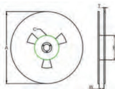
图3 轮盘尺寸图
