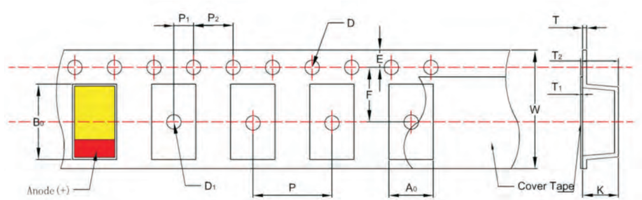
图2载带尺寸图
