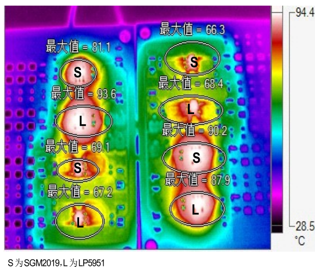
图 1 类似器件不同 \theta_{ja} 标称散热热像对比
