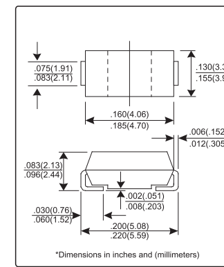
SMB(DO-214AA)
