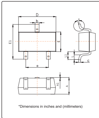
SOT-23
