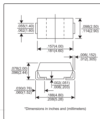
SMA(DO-214AC)
