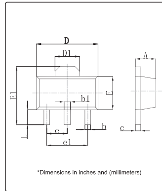
SOT-89
