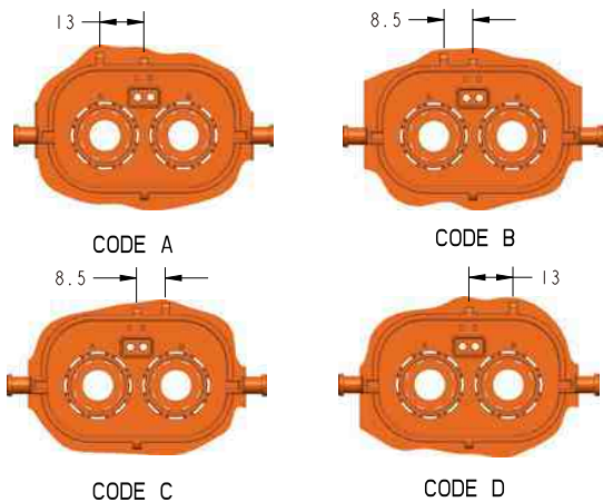
2-Pole Receptacle 2芯插座编码
