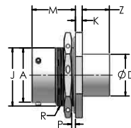
07: Jam nut Receptacle 锁紧螺母插座
