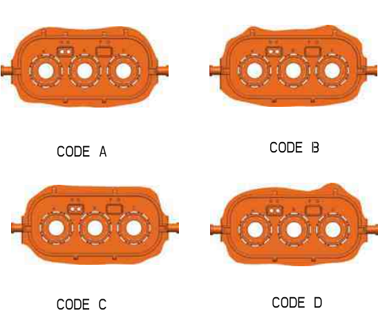
3-Pole Receptacle 3芯插座编码
