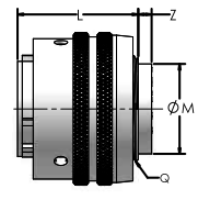
06: Straight Plug 直插头
