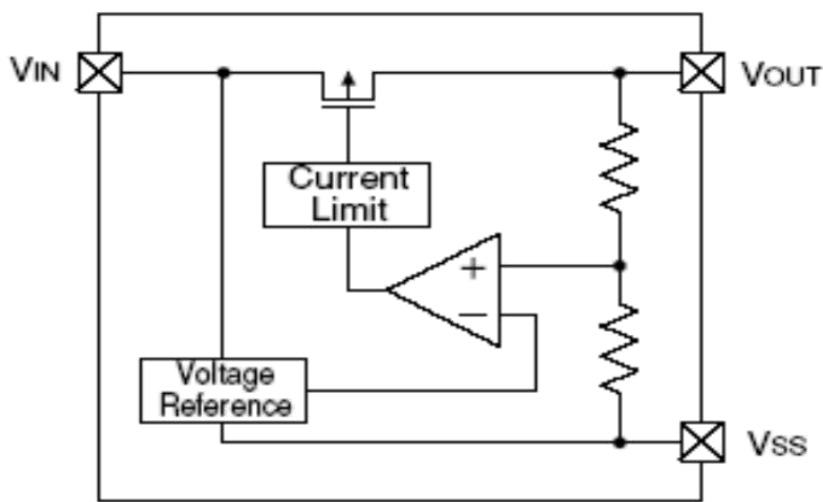
功能块框图
