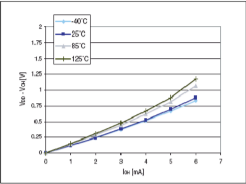
图34： V_{DD} - V_{OH} @ V_{DD} = 3.3\text{ V} （标准端口）
