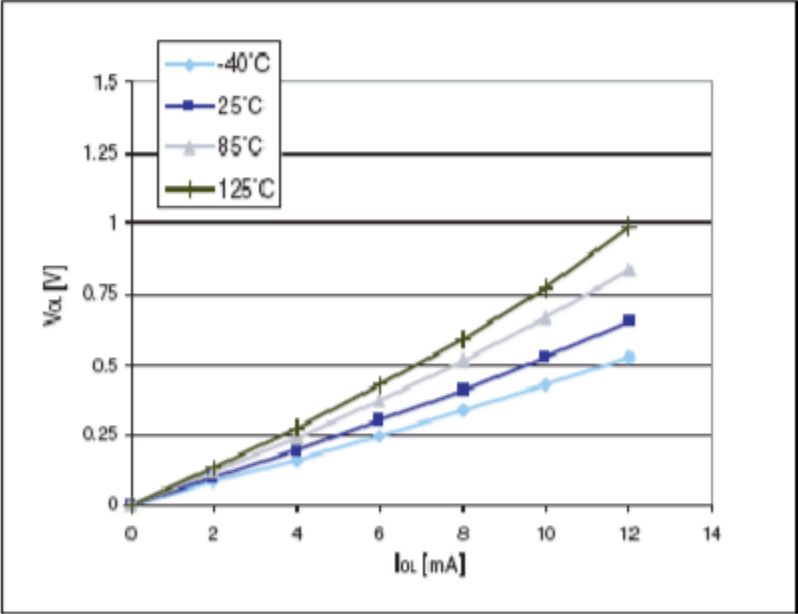
图32：Typ. V_{OL} @ V_{DD} = 3.3\text{ V} （高接收端口）
