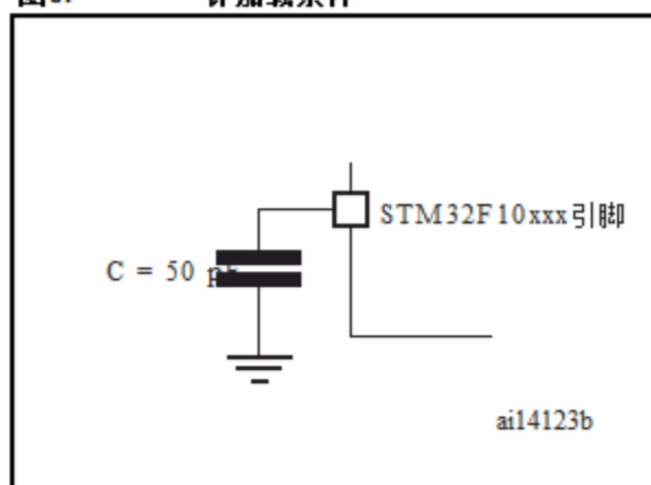
图8. 针加载条件
