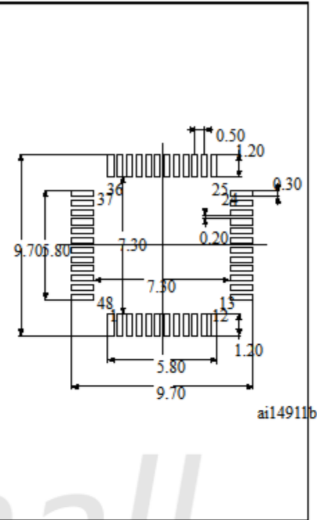
图43. 推荐的 足迹 (1) (2)
