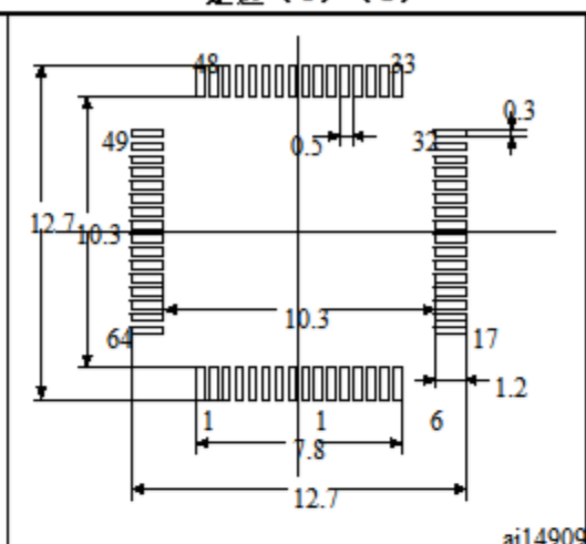
图39. 推荐的 足迹 (1) (2)
