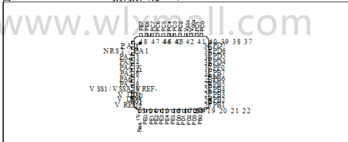
图7. STM8L151Cx 48引脚引脚 (无LCD)
