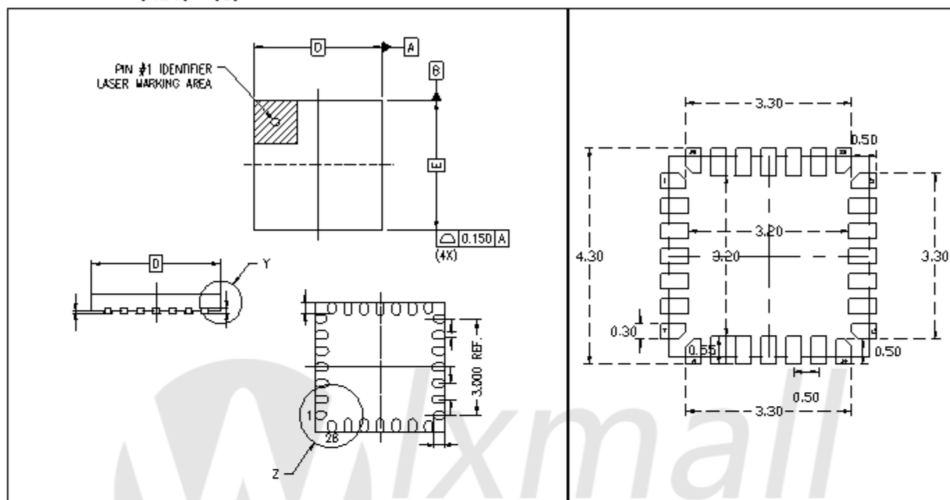
图42. UFQFPN28 - 28引线非常非常细细 间距四边形无引线封装外形 (4x4) (1)
