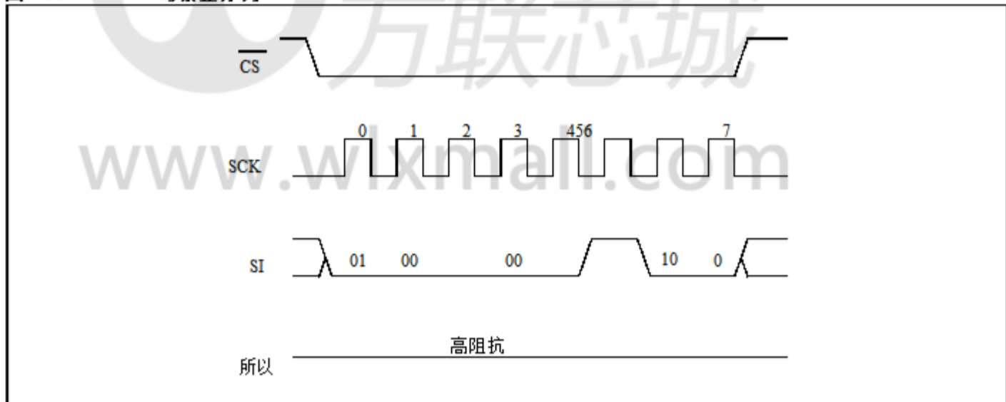
图 3-5: 写禁止序列
