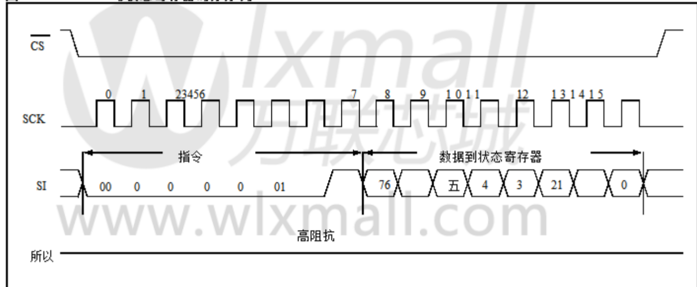
图 3-7: 写状态寄存器时序序列
