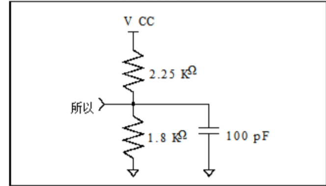
图1-4: 交流测试电路
