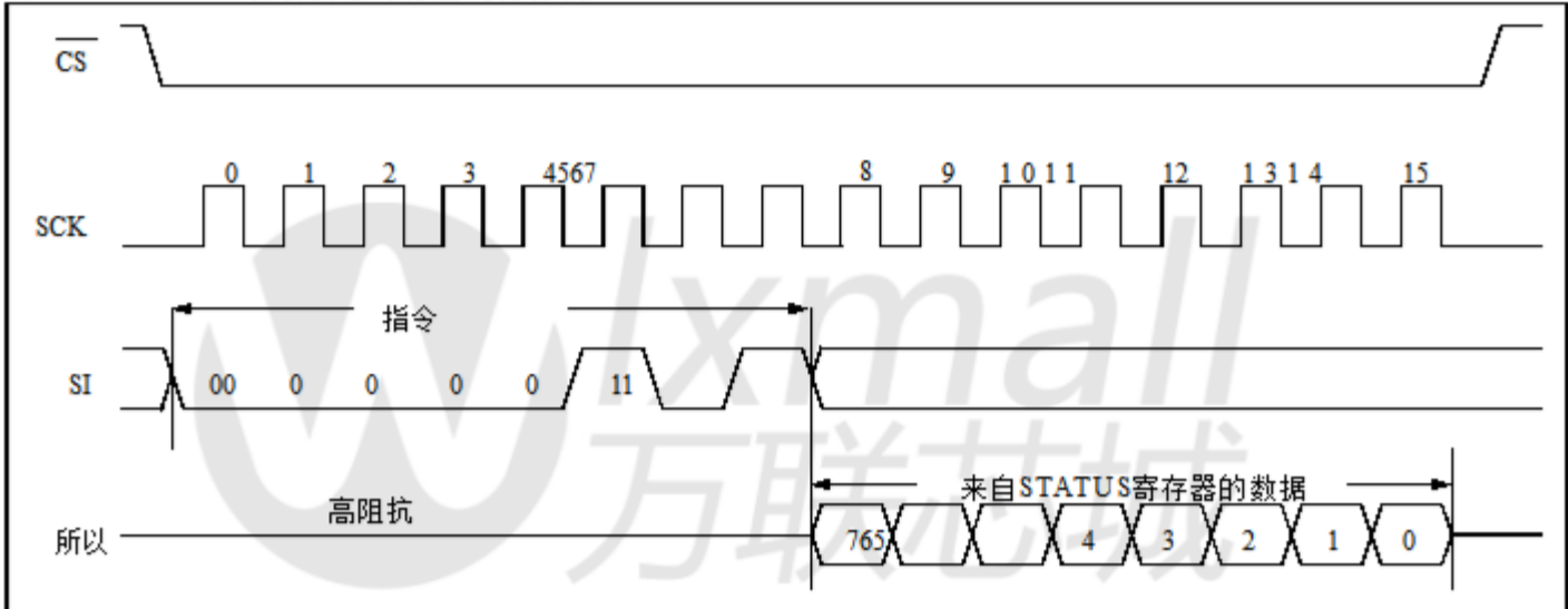
图 3-6: 读取状态寄存器时序序列
