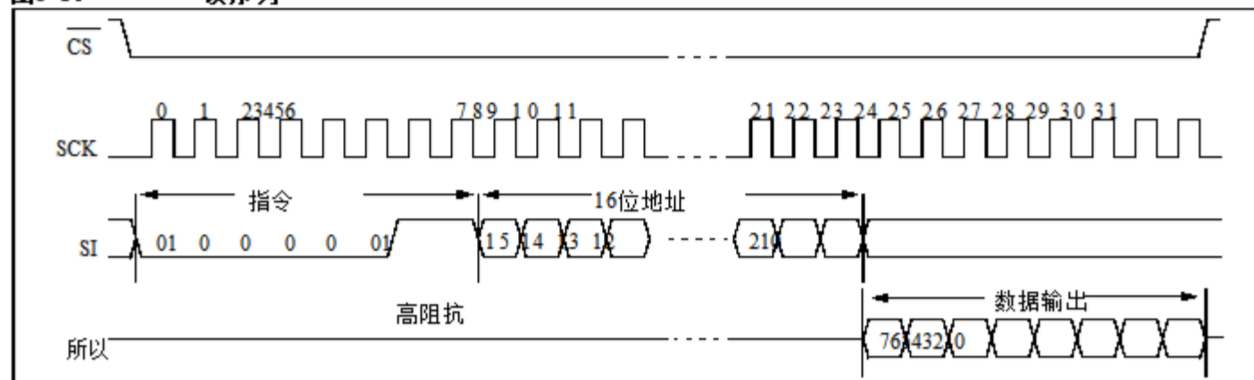
图3-1: 读序列
