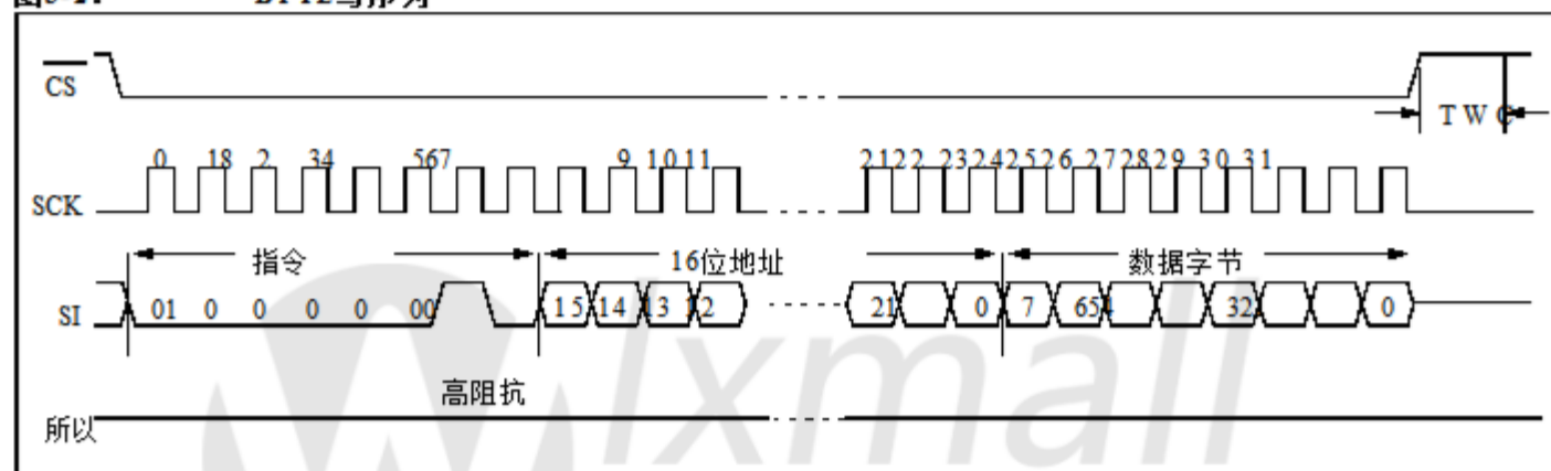
图3-2: BYTE写序列
