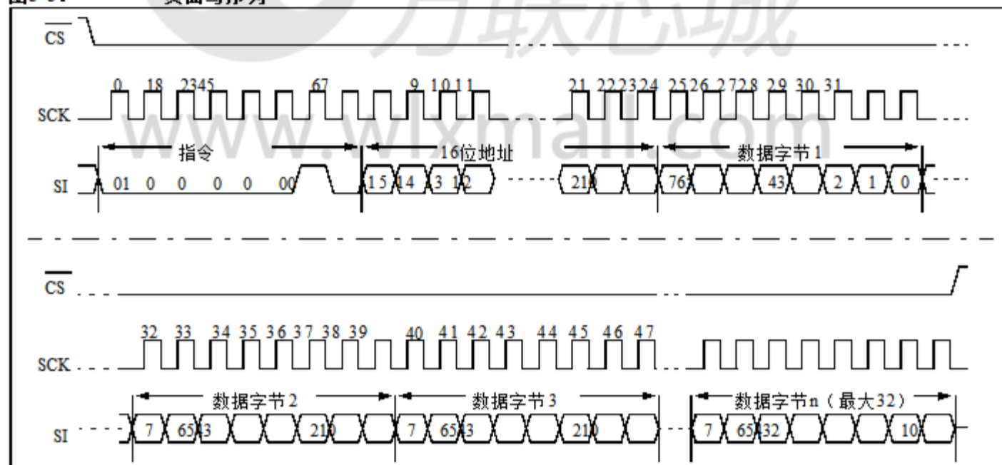
图3-3: 页面写序列
