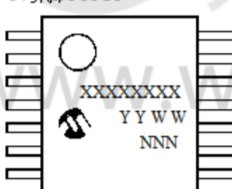
14引脚TSSOP
