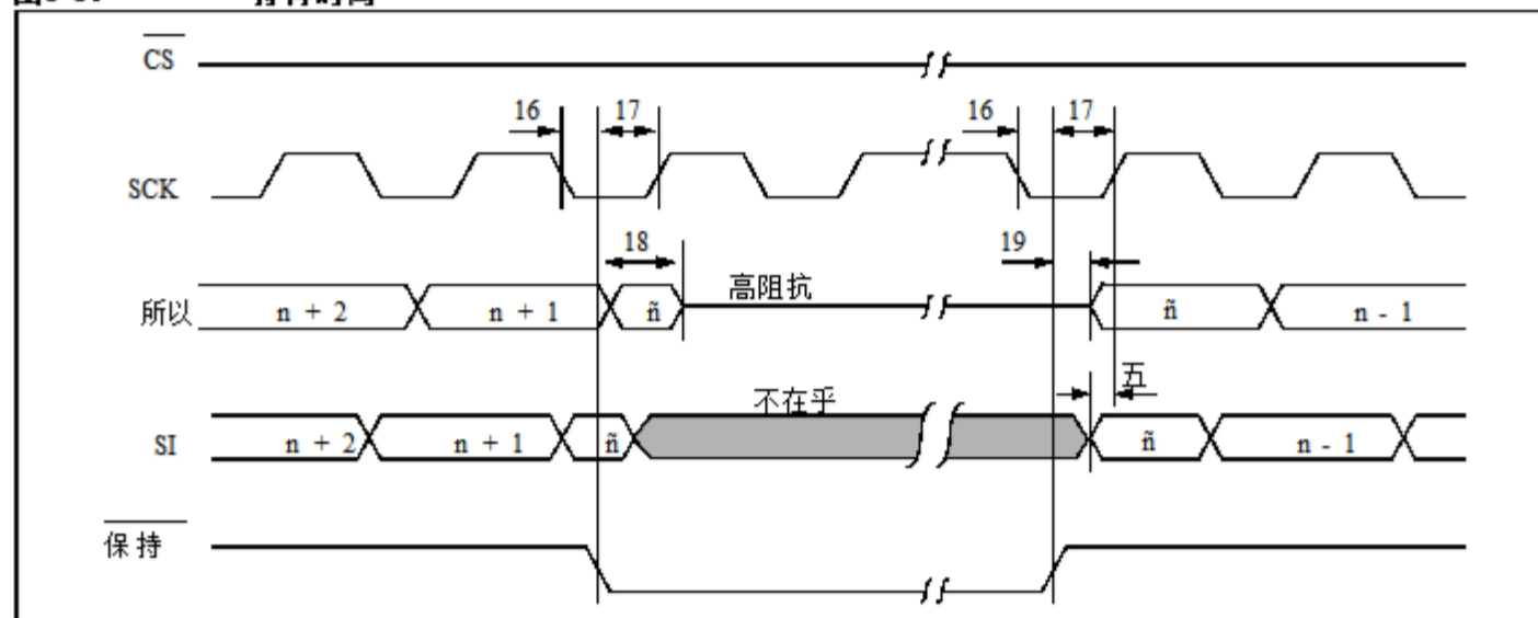
图1-1: 持有时间
