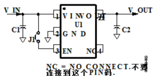
图3. ADP150UJZ-RedyKit评估板原理图
