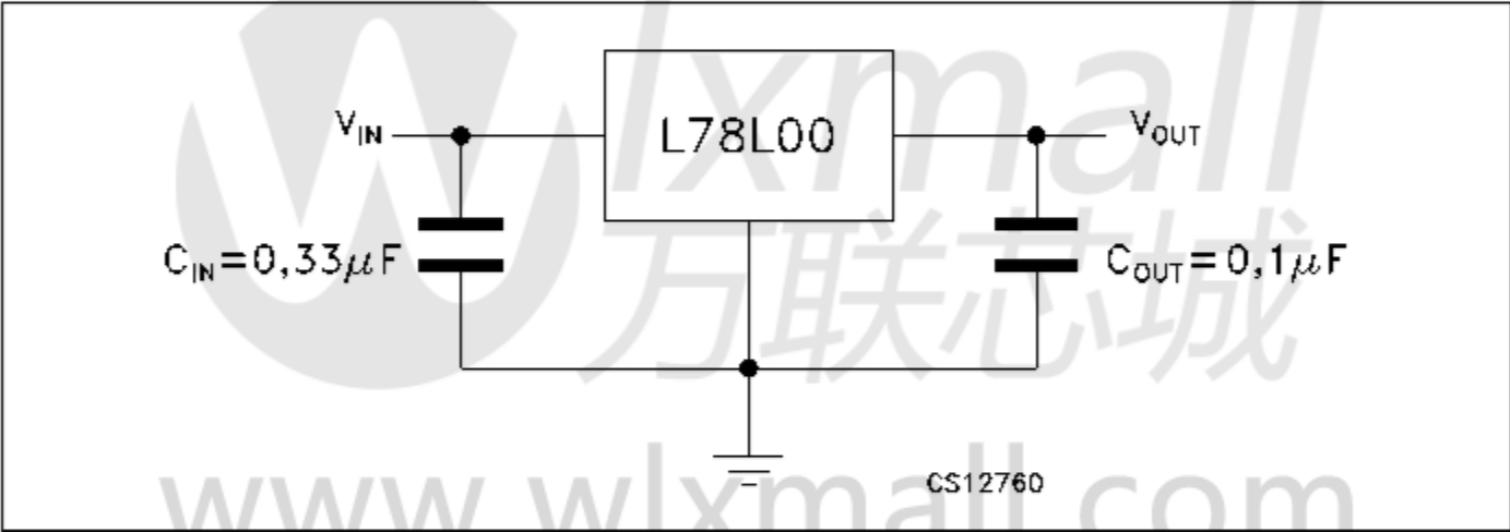
图3.测试电路
