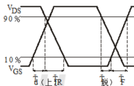
图10b - 开关时间波形
