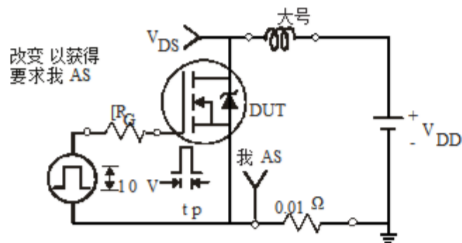
图12a - 无钳位电感测试电路
