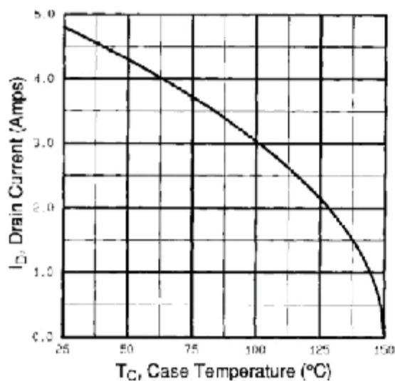
图9 - 最大漏极电流与外壳温度的关系
