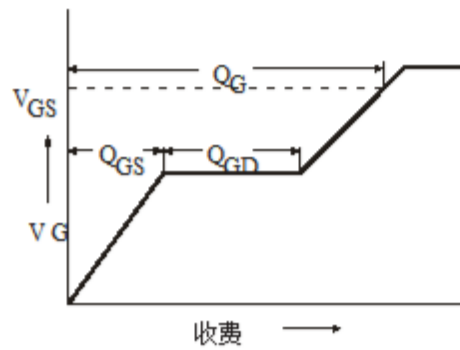
图13a - 基本门电荷波形
