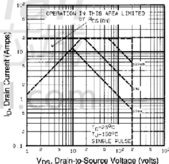
图8 - 最大安全工作区域
