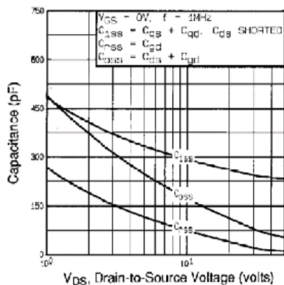
图5 - 典型电容与漏源电压
