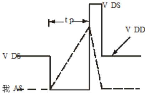
图12b - 非钳位感应波形
