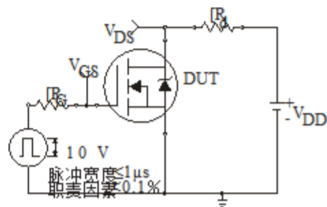
图10a - 开关时间测试电路
