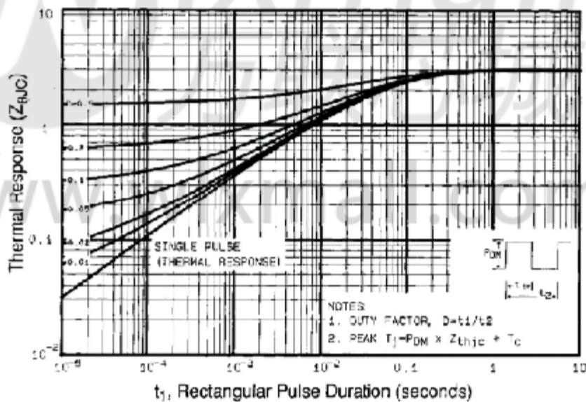
图11 - 最大有效瞬态热阻抗，结到外壳
