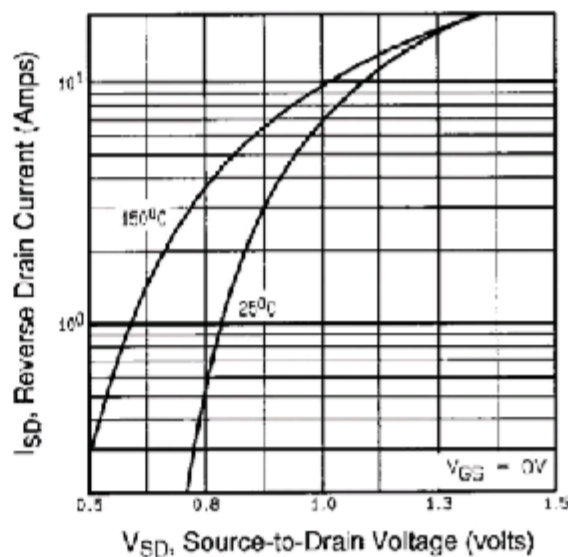
图7 - 典型的源极 - 漏极二极管正向电压
