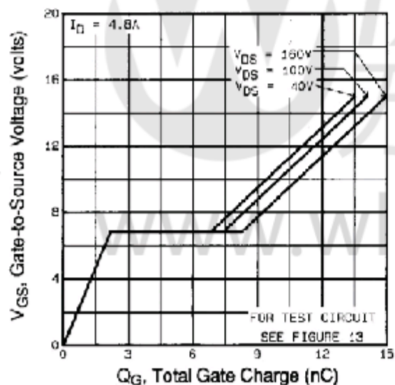
图6 - 典型栅极电荷与栅源电压的关系
