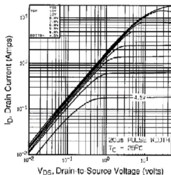
图1 - 典型输出特性, T_C = 25^\circ\text{C}
