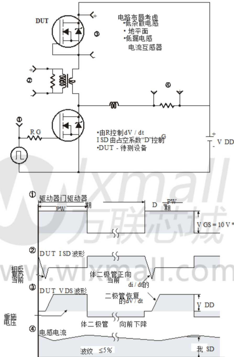
峰值二极管恢复 dV/dt 测试电路
