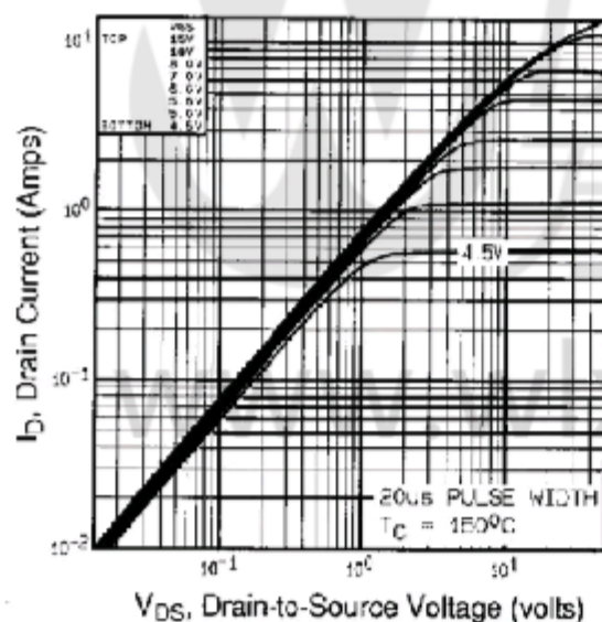
图2 - 典型输出特性, T_C = 150^\circ\text{C}
