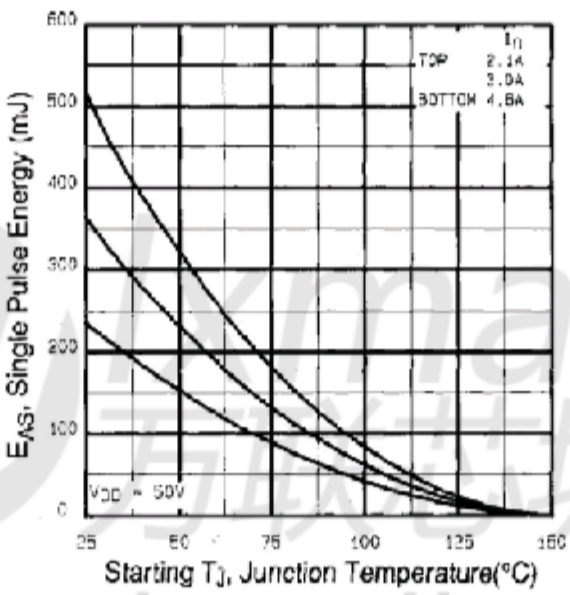
图12c - 最大雪崩能量与漏电流
