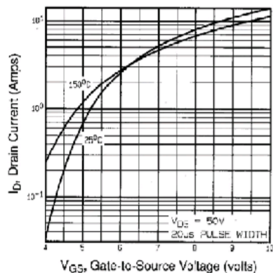
图3典型的传输特性
