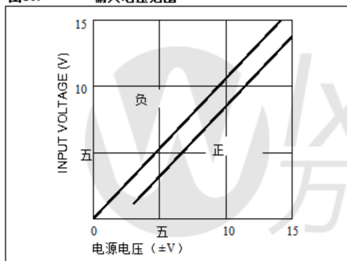
图10. 输入电压范围
