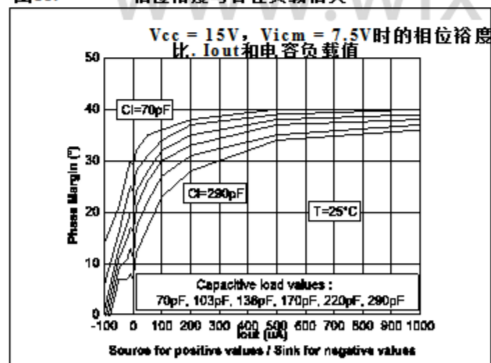
图18. 相位裕度与容性负载相关
