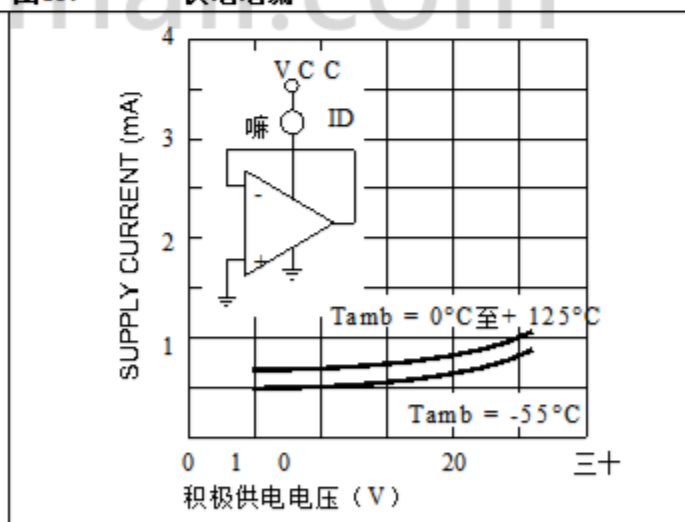
图13. 供电电流
