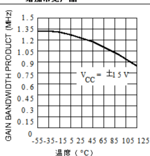
图15. 增加带宽产品
