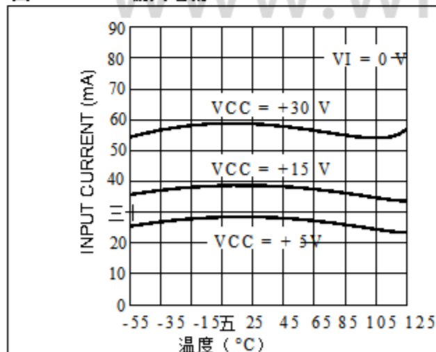
图6. 输入电流
