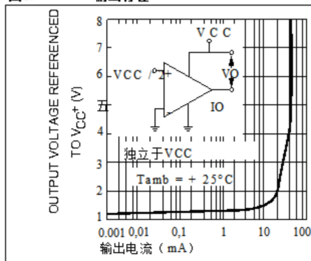
图8. 输出特性
