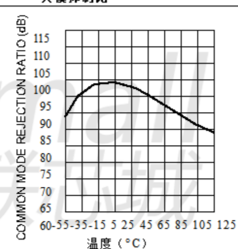
图17. 共模抑制比
