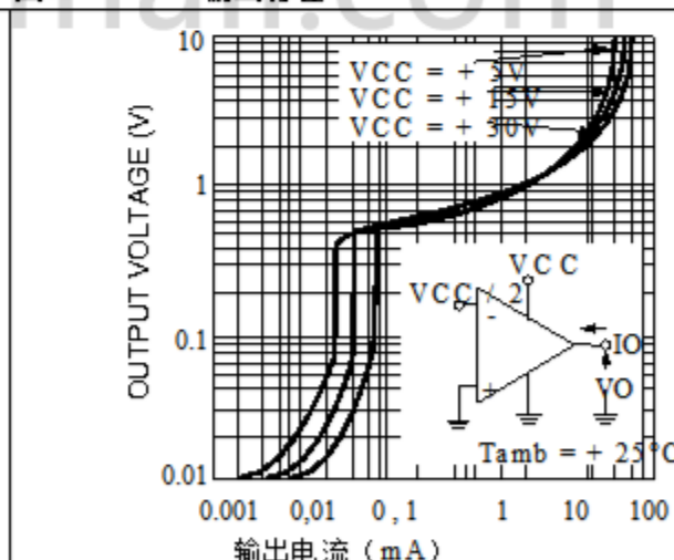
图7. 输出特性
