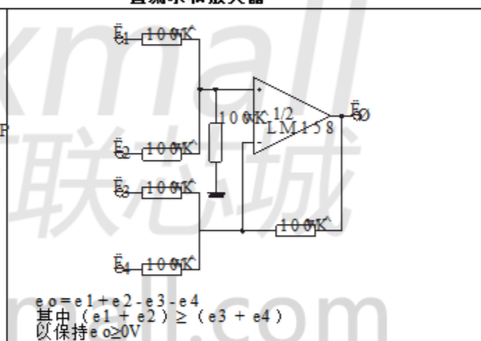
图22. 直流求和放大器
