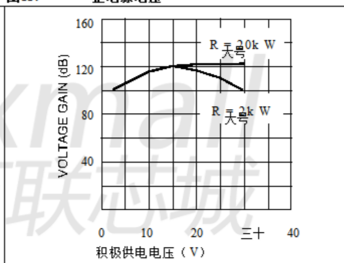
图11. 正电源电压
