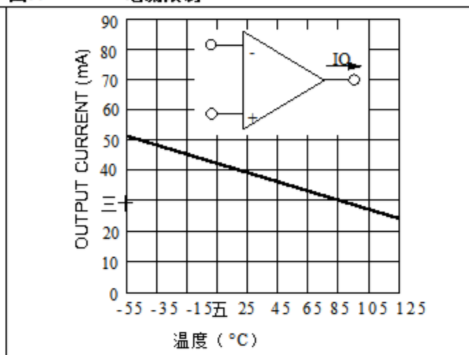
图9. 电流限制
