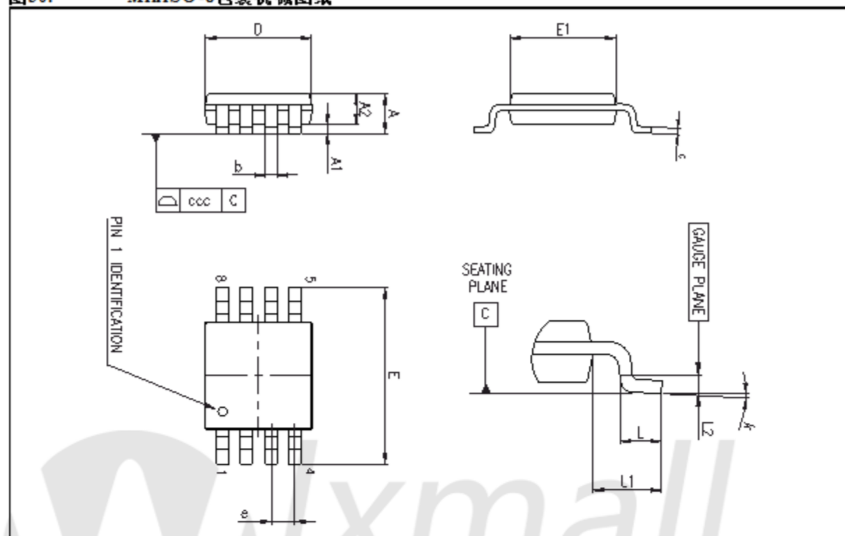
图30. MiniSO-8包装机机械图纸
