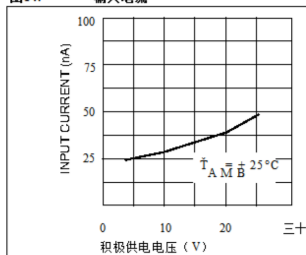
图14. 输入电流
