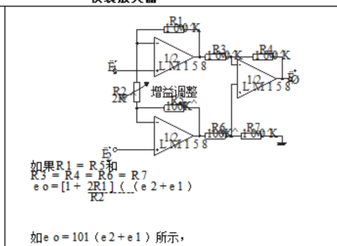
图24. 高输入Z可调增益直流仪表放大器
