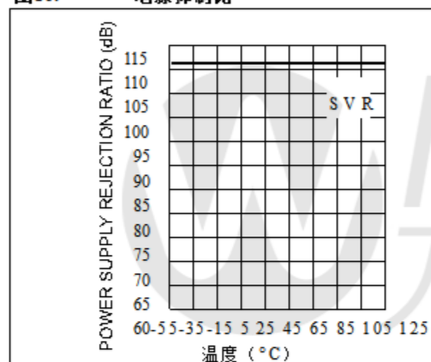
图16. 电源抑制比
