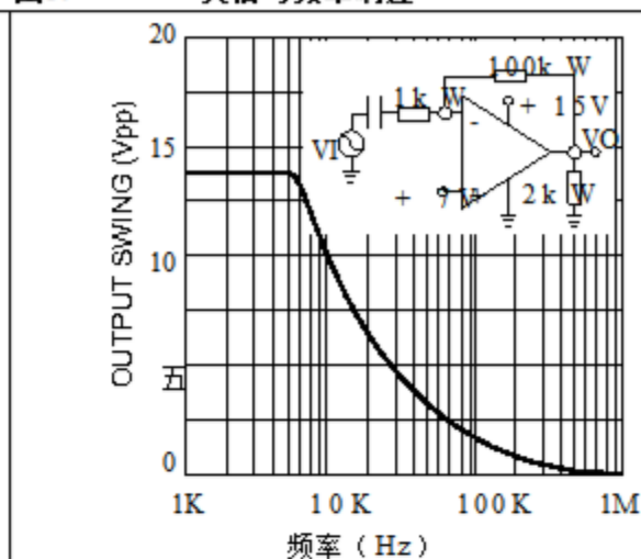
图3. 大信号频率响应
